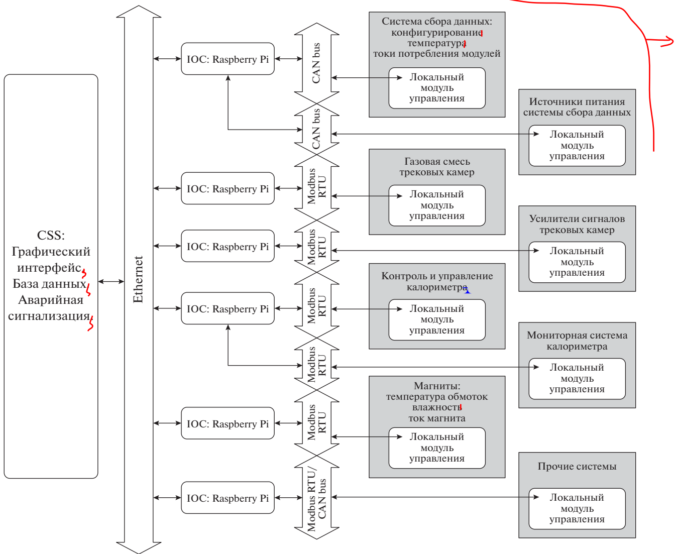
Рис. 1. Архитектура системы управления детекторами установки СПАСЧАРМ.
