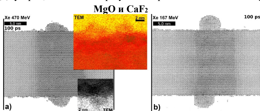
Рис. 11.4 – (a) Кристаллический бугорок на поверхностях плёнки MgO, образованного после облучения 470 МэВ Хе по сравнению с изображениями ABF STEM на вставках; и (b) имитированный МД бугорок, возникший в результате пролёта 167 МэВ Хе в MgO
