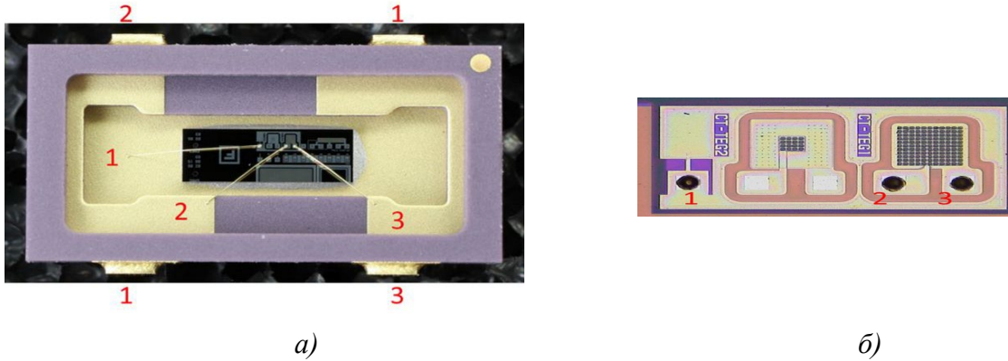
Рис. 5.10 – Фотографии тестовой структуры в корпусе (а) и части тестовой структуры (б), на которой расположена матрица 11x11 ячеек (цифрами отмечены электроды: 1 – общий катод, 2 – анод одной ячейки, 3 – анод 120 ячеек)
