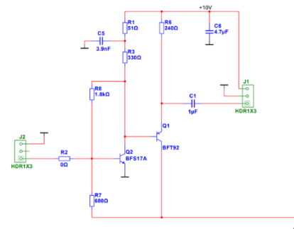
Рис. 5.12– Схема усилителя
