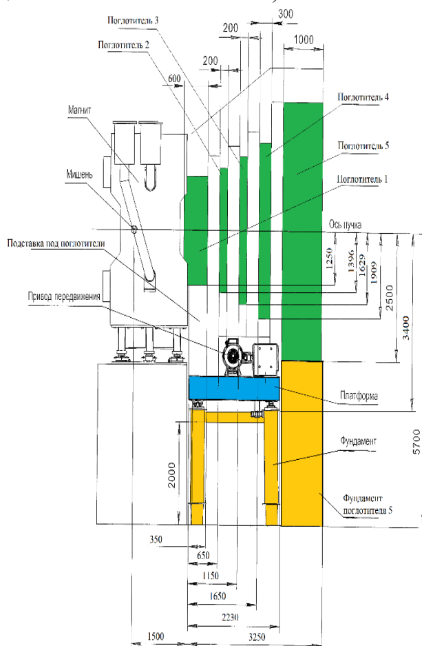
Рис. 12.28 – Схема расположения поглотителей в детекторе MUCH
