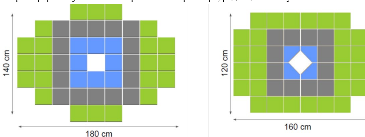
Рис. 12.15 - Схема общего вида переднего адронного калориметра (слева) и схема отдельного модуля PSD (справа)
