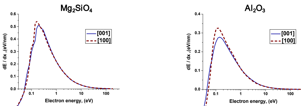
Рис. 11.16 – Упругие потери энергии электронов с начальными импульсами по направлениям [100] и [001] в кристаллах Mg_2SiO_4 и \alpha-Al_2O_3
