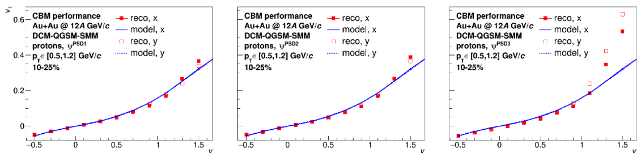
Рис. 12.59 – Направленный поток протонов как функция быстроты, извлеченный относительно плоскостей симметрии из подсобытий PSD1, PSD2 и PSD3; центральность 10-25%; линиями показаны значения, полученные из генератора столкновений
