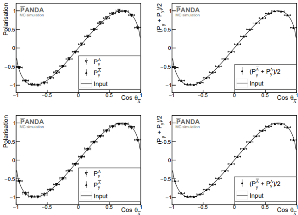
Рис. 14.3 – Поляризация \bar{\Lambda} (черный) и \Lambda (открытый) при p_{\text{beam}}=1,642 ГэВ/с
