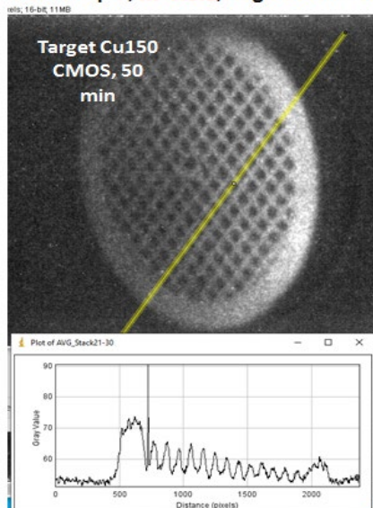
Рис. 11.2 – Рентгеновское изображение профиля пучка и мишени (вверху), полученное с использованием камеры sCMOS и профиль интенсивности (внизу)
