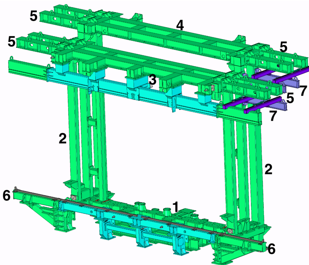
Рис. 12.41 – Общий вид надстройки МУСН
