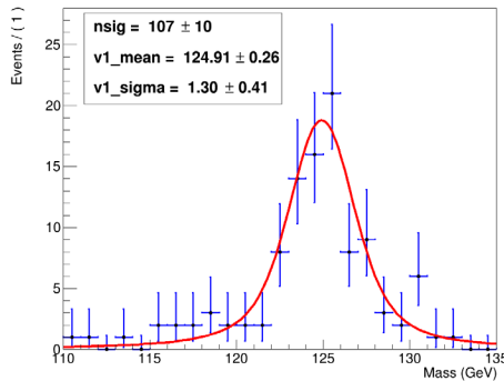
Рис. 5.5 – Распределение по разности масс M(jjll) - M(jj) + M(Z_{nom}) в канале e^+e^- \rightarrow Z_1(nn)H(Z^*Z)
