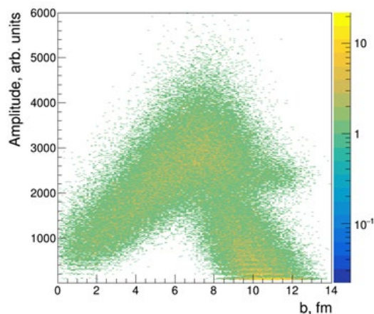
Рис. 8.10 – Корреляция между амплитудой FWall и прицельным параметром, полученная для событий MB, сгенерированных с помощью модели DCM-QGSM-SMM для Ag + Ag при 1.58 ГэВ/нуклон
