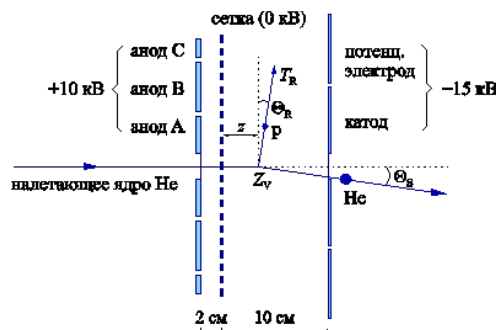
Рис. 6.2 – Схематическое изображение (не в масштабе) одного из шести модулей ИКАРа вместе с типичным событием рассеяния налетающего ядра He на протоне в рабочем объёме, где T_R – энергия протона отдачи, z – расстояние от точки взаимодействия Z_V до сетки, а \Theta_R и \Theta_S – углы рассеяния протона и налетающего ядра, соответственно
