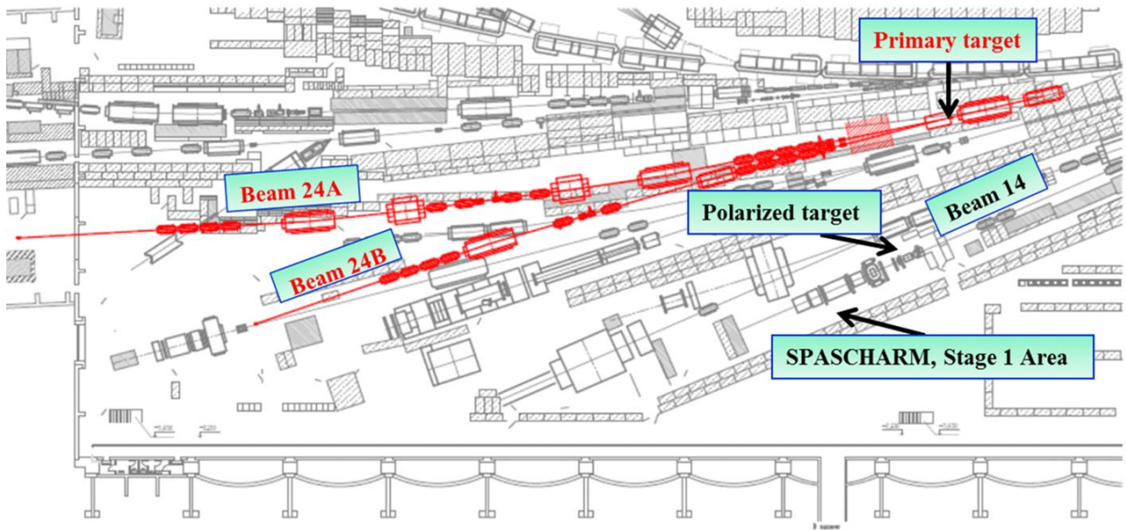
Рис. 2.1 Схема размещения каналов 24А и 24В в экспериментальном зале 1ВВ ускорителя У-70
