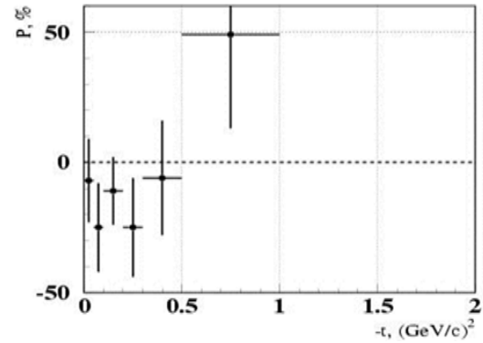
Рис. 1.15 Асимметрия в реакции \pi p^+ \rightarrow \eta'(958)n при энергии 40 ГэВ [131], когда \eta'(958) -мезон регистрировался в моде распада на два \gamma -кванта
