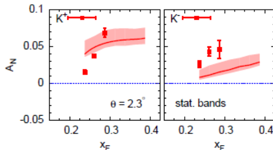
Рис. 5.17 Зависимость A_N(x_F) для K^\pm , из работы [164]
