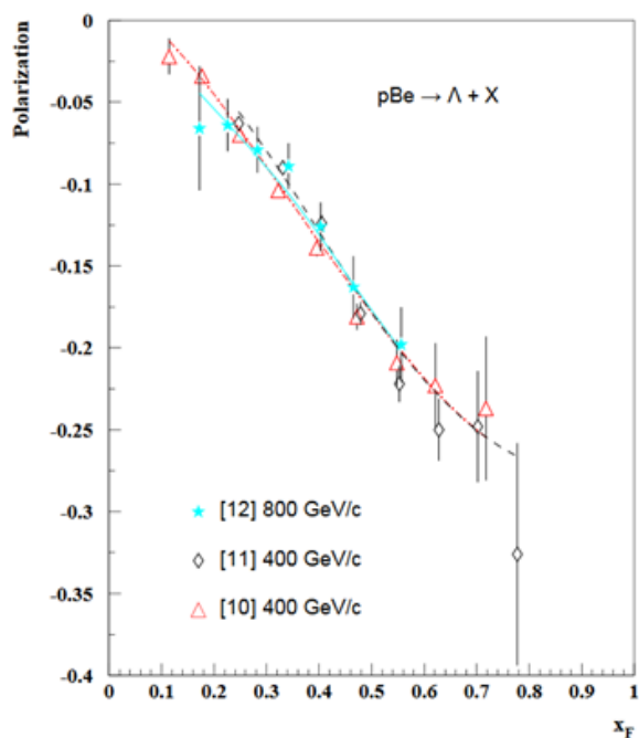
Рис. 5.9 P_N в реакции pBe \rightarrow \Lambda + X
