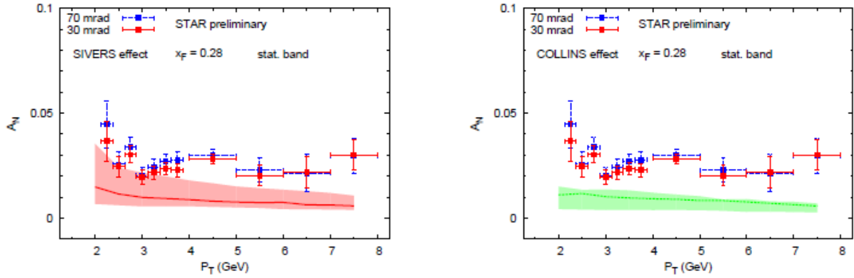
Рис. 5.18 Зависимость A_N(p_T) для реакции p^+p^- \rightarrow \pi^0 X , из работы [165], и предсказания в рамках моделей Сиверса (слева) и Коллинза (справа)
