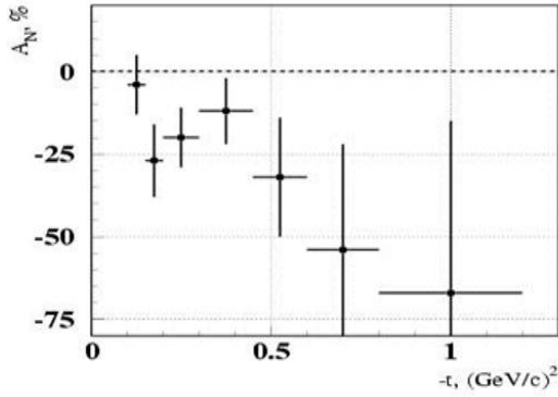
Рис. 1.14 Асимметрия в реакции \pi p^+ \rightarrow \omega(782)n при энергии 40 ГэВ [55], когда \omega(782) -мезон регистрировался в моде распада на \pi^0 и \gamma
