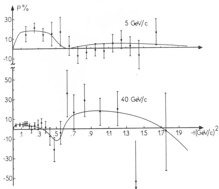
Рис. 5.3 Модель оддерона [130] в применении к описанию поляризации в реакции \pi^- p^\uparrow \rightarrow \pi^0 n при импульсах 5 и 40 ГэВ/с [53]
