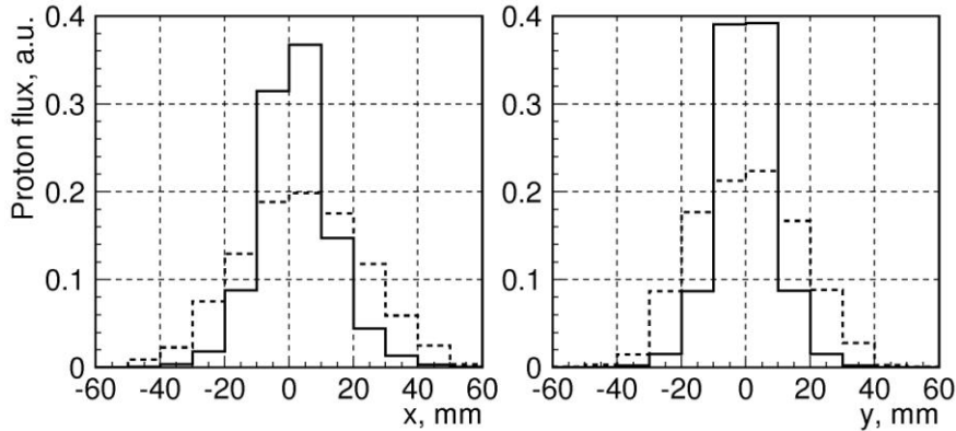
Рис. 2.7 Профили пучка на мишени экспериментальной установки для p = 45 \text{ ГэВ}/c и \sigma_p/p_0 = 1.2\% (сплошная линия) и для p = 15 \text{ ГэВ}/c и \sigma_p/p_0 = 4.5\% (пунктирная линия)
