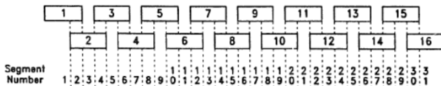
Рис. 2.13 Структура «гребешкового» годоскопа мечения пучка с перекрывающимися сцинтилляторами.
