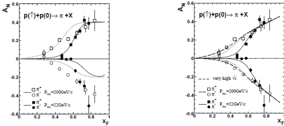
Рис. 5.19 A_N(x_F) для p^\uparrow p \rightarrow \pi^\pm X для разных значений параметров Берлинской модели [171]
