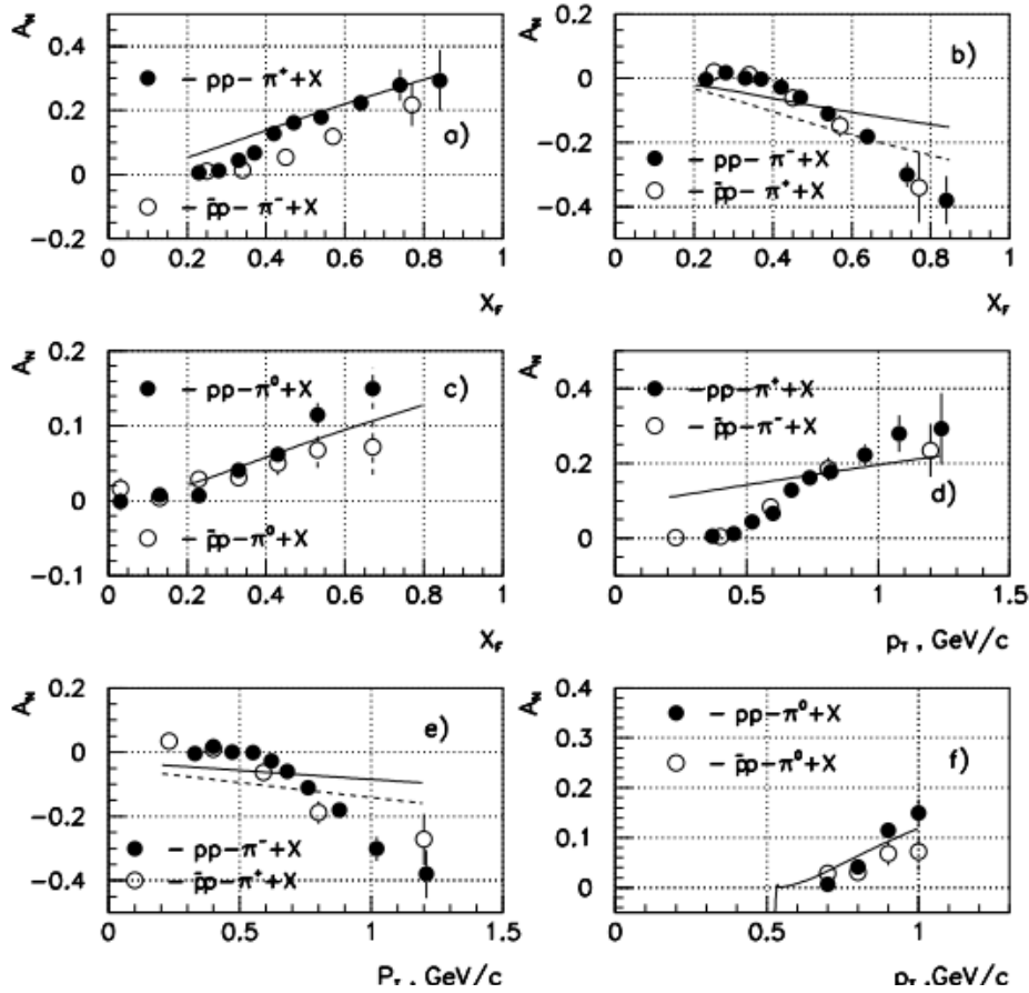
Рис. 5.26 Сравнение данных E704 для p^+p (черные кружочки) [23] и p^-p (открытые кружочки) [189], из работы [187]
