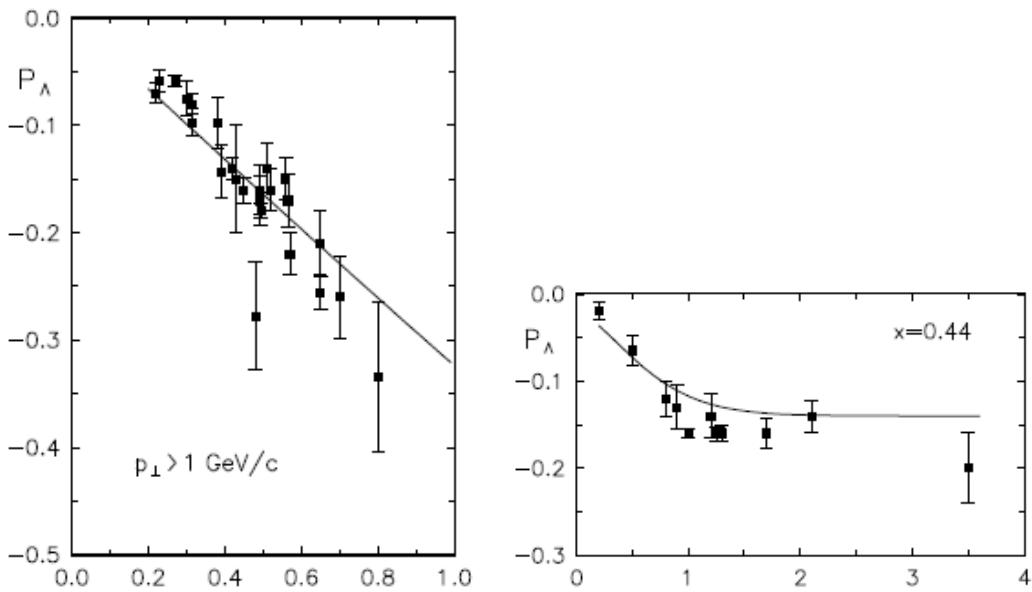
Рис. 5.24 P_N(x_F) для pp \rightarrow L^1 X (слева) и P_N(p_T) для pp(A) \rightarrow L^1 X (справа) из работы [182]
