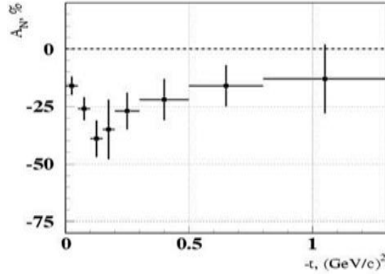
Рис. 5.4 Асимметрия в реакции \pi^+ p \rightarrow f_2(1270) n при энергии 40 ГэВ [131], когда f_2(1270) -мезон регистрировался в моде распада на два \pi^0 -мезона
