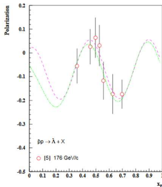
Рис. 5.14 P_N в реакции \bar{p}p \rightarrow \bar{\Lambda} + X
