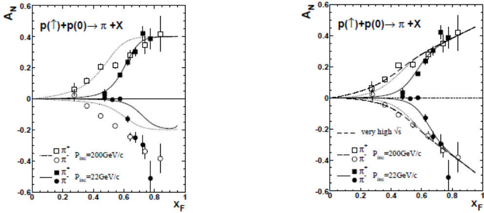
Рис. 5.19 A_N(x_F) для p^\uparrow p \rightarrow \pi^+ X для разных значений параметров Берлинской модели [183]
