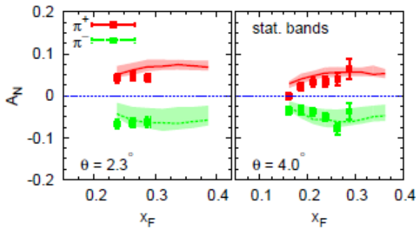
Рис. 5.15 Зависимость A_N(x_F) для p^+p^- \rightarrow \pi^\pm X , из работы [177]
