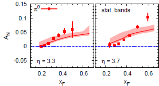
Рис. 5.16 Зависимость A_N(x_F) для p^+p^- \rightarrow \pi^0 X , из работы [177]
