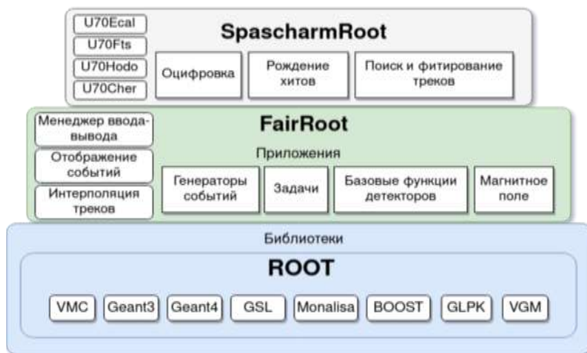
Рис. 3.52 Схематическая структура программной среды эксперимента СПАСЧАРМ: внизу — библиотеки сторонних разработчиков, в центре — среда FairRoot, вверху — конкретная реализация SpascharmRoot
