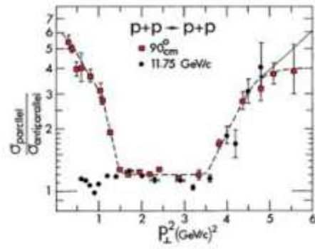
Рис. 5.2 Отношение упругих сечений \sigma^{\uparrow\uparrow}/\sigma^{\uparrow\downarrow} в зависимости от P_{\perp}^2 [140]
