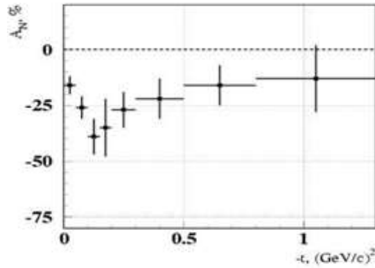
Рис. 5.4 Асимметрия в реакции \pi^- p^\dagger \rightarrow f_2(1270) n при энергии 40 ГэВ [143], когда f_2(1270) -мезон регистрировался в моде распада на два \pi^0 -мезона
