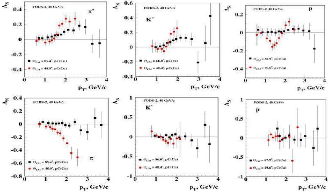
Рис. 5.7 Зависимость A_N(p_T) для процессов инклюзивного образования \pi^+ , \pi^- , p и \bar{p} в p^\dagger A -соударениях при двух углах рождения адронов и импульсе 40 ГэВ/с
