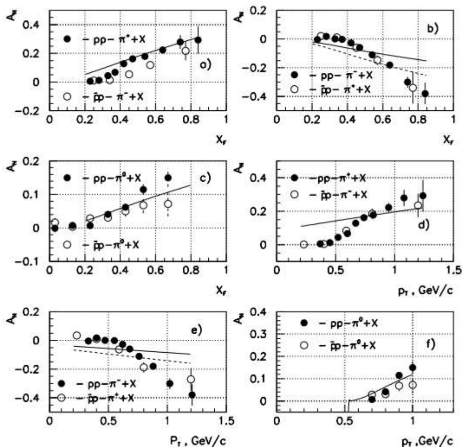
Рис. 5.26 Сравнение данных E704 для p^+p (черные кружочки) [26] и \bar{p}^+p (открытые кружочки) [201], из работы [199]
