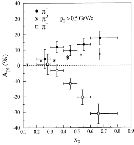
Рис. 1.7 Слева A_N в \bar{p}^1 -взаимодействии в инклюзивном рождении заряженных [33] и нейтральных [32] мезонов, справа — аналогичный результат для pp -взаимодействия [26, 32]
