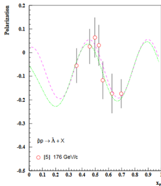
Рис. 5.14 P_N в реакции \tilde{p}p \rightarrow \tilde{\Lambda} + X
