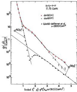
Рис. 5.1 Сечение протон-протонного упругого рассеяния в зависимости от скейлинговой переменной p_T^2 = \beta^2 P_{\perp}^2 \sigma_{tot}(s)/38.3 [139].
