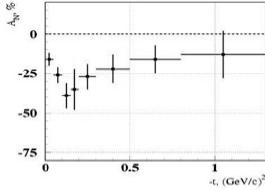
Рис. 5.4 Асимметрия в реакции \pi^- p^\uparrow \rightarrow f_2(1270) n при энергии 40 ГэВ [143], когда f_2(1270) -мезон регистрировался в режиме распада на два \pi^0 -мезона
