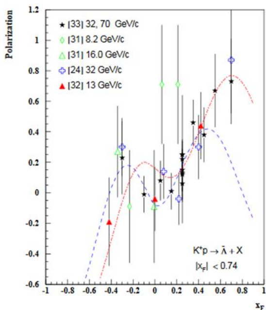
Рис. 5.13 P_N в реакции K^*p \rightarrow \tilde{\Lambda} + X
