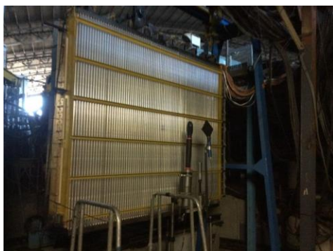
Рис. 3.29 Четвертая станция камер на рабочем месте с установленным перед ней триггерным счетчиком на взаимодействии; справа — третья станция, расположенная сразу после магнита.
