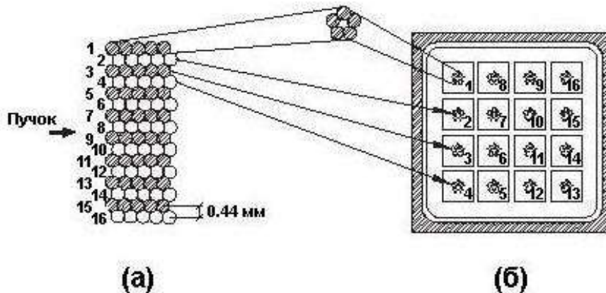
Рис. 3.5 Схематическое изображение части сцинтилляционной волоконной кассеты (а) и расположение волокон на фотокатоде 16-анодного ФЭУ Hamamatsu R7600-200-M16 (б)
