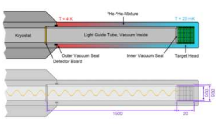
Рис. 3.19 Поляризованная мишень-сцинтиллятор (Майнц)
