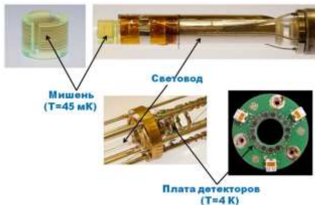
Рис. 3.18 Основные внутренние узлы созданной совместными усилиями (Майнц-Бонн-Бохум-ОИЯИ) мишени-сцинтиллятора
