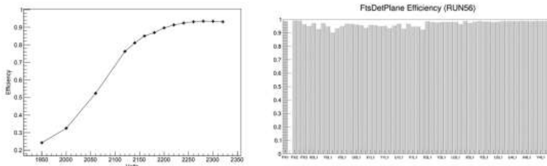
Рис. 3.32 Слева – зависимость эффективности одного из слоев камеры от напряжения, справа – эффективность всех слоев трековой системы, полученная на вторичных треках
