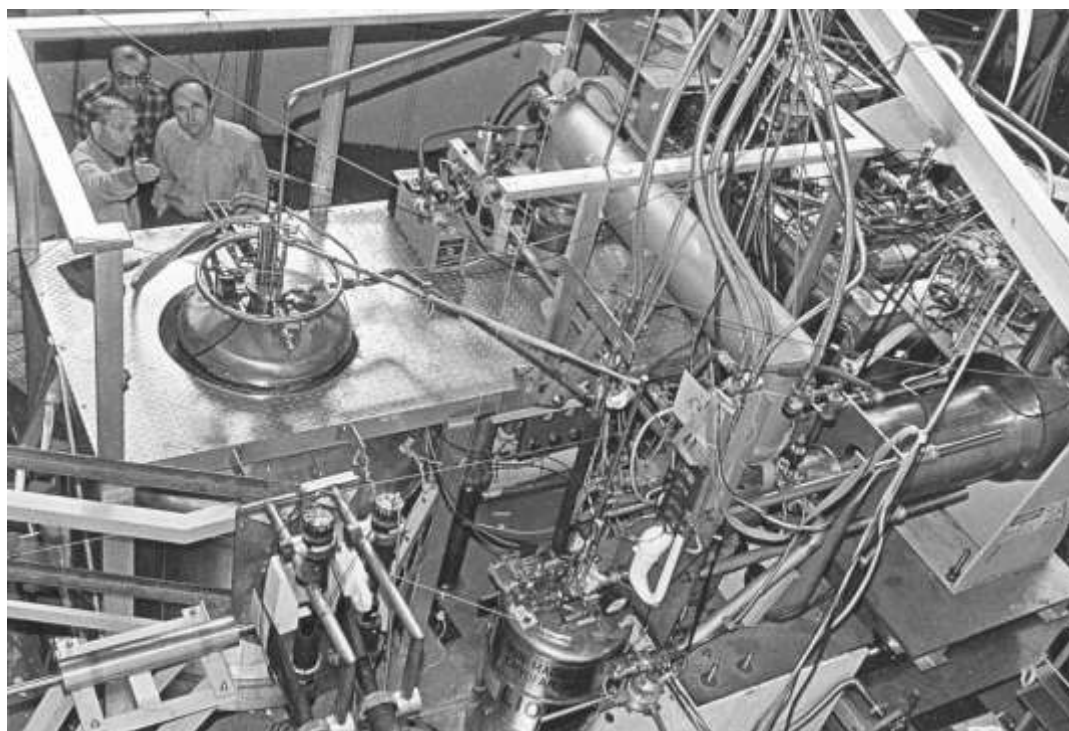
Рис. 3.15 Фотография комплекса продольной поляризованной мишени
