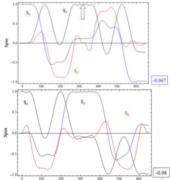
Рис. 2.28 Спиновые траектории для поперечной (сверху) и продольной (снизу) поляризации
