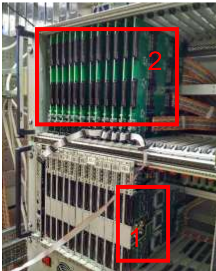
Рис. 3.49 Мезонинная плата, установленная на модуль ЕвроМИСС — 1; переходные платы — 2
