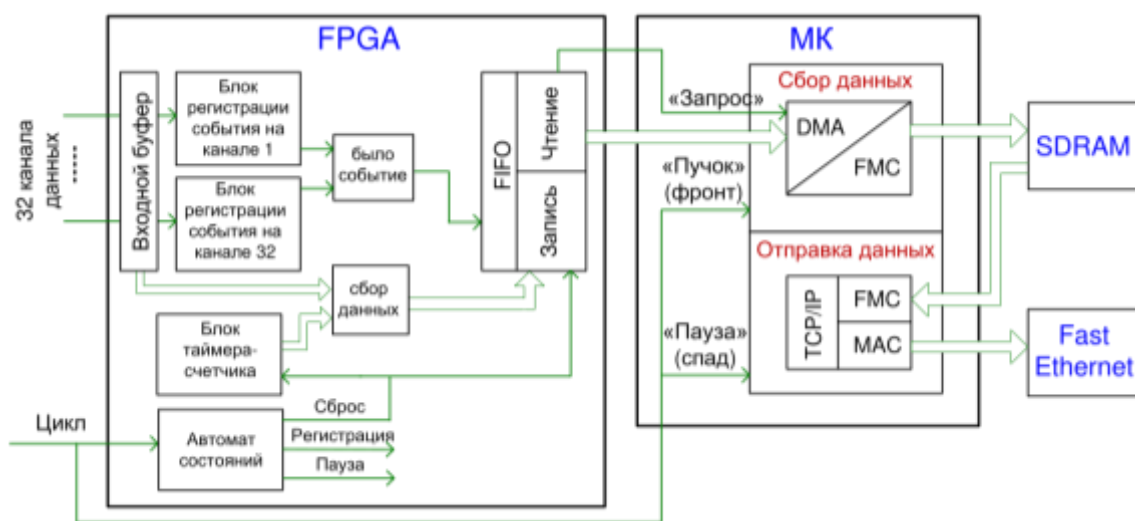
Рис. 2.18 Общий алгоритм взаимодействия двух плат прототипа
