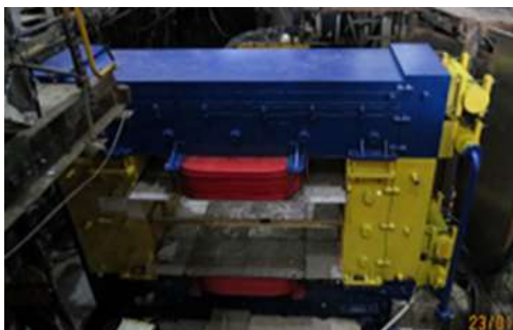
Рис. 3.20 Фотография спектрометрического магнита М31 на канале 14
