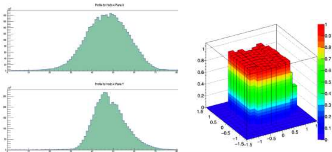
Рис. 3.7 Профили пучка (слева) и зависимость эффективности волоконного годоскопа от координаты (справа)
