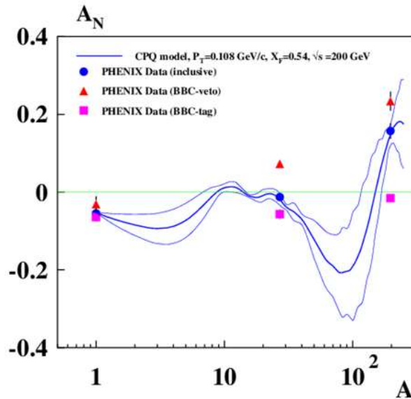
Рис. 1.9 Зависимость A_N(A) для реакции p^\dagger A \rightarrow nX в эксперименте ФЕНИКС [29]
