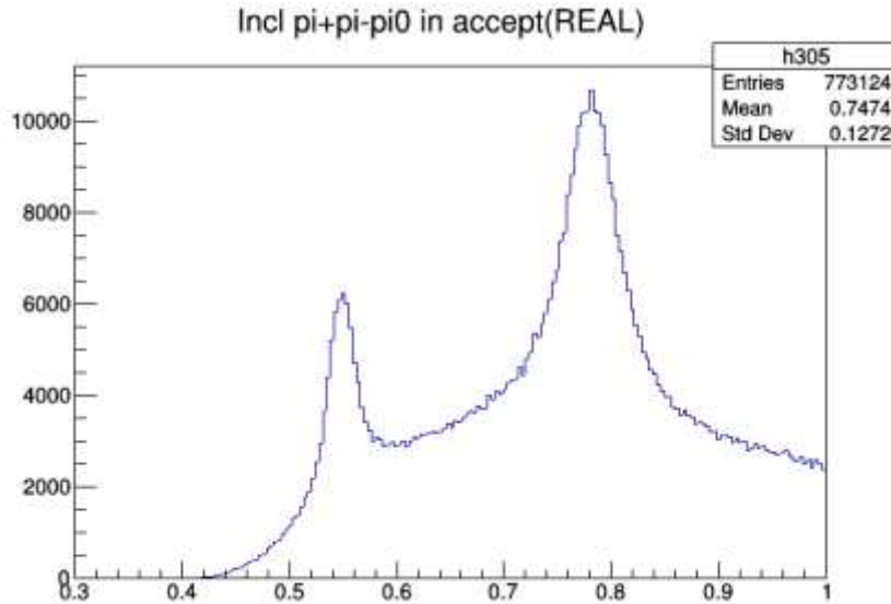
Рис. 1.11 Спектры масс \pi^+ \pi^- \pi^0 в ГэВ/с 2
