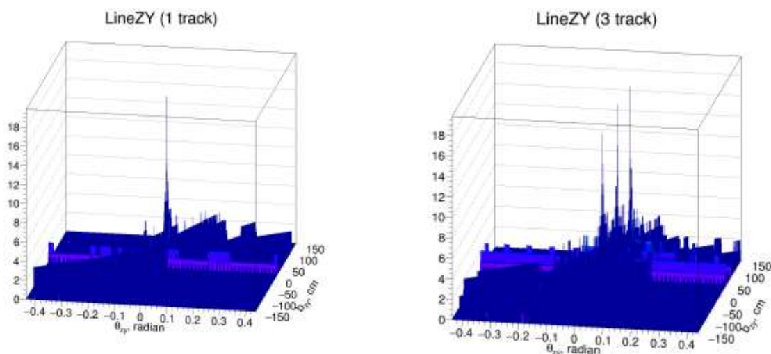
Рис. 3.58 Примеры полученных пространств Хафа в плоскости ZY для одного трека (слева) и трех (справа)
