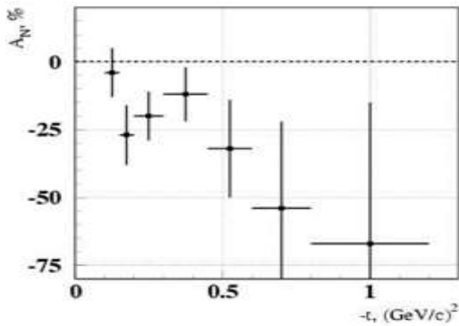
Рис. 1.14 Асимметрия в реакции \pi p^{\uparrow} \rightarrow \omega(782)n при энергии 40 ГэВ [62], \omega -мезон регистрировался в моде распада на \pi^0 и \gamma
