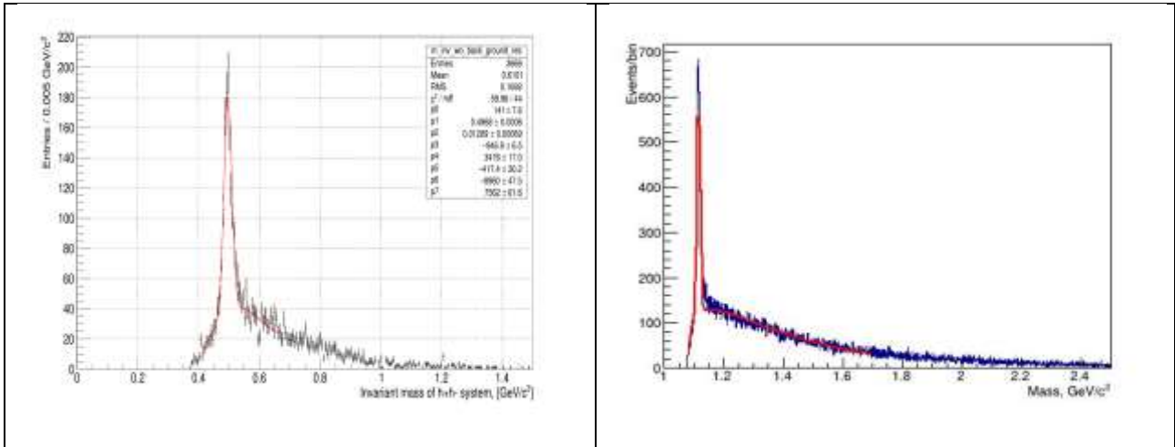
Рис. 1.16 – Массовые спектры h^+h^- пар, полученные при первом анализе данных на пучке \pi^- мезонов (слева) и K^- мезонов (справа)
