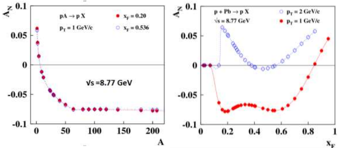
Рис. 1.10 Предсказания A_N в рамках модели хромомагнитной поляризации кварков
