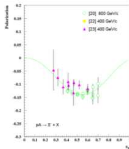
Рис. 5.10 P_N в реакции pA \rightarrow \Xi^- + X
