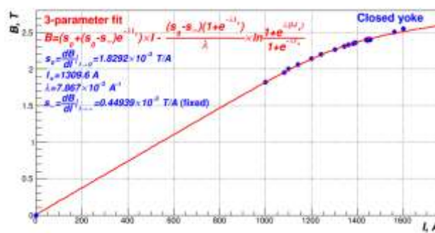
Рис. 3.12 Нагрузочная кривая магнита ДИНОЗАВР поляризованной мишени при сомкнутых полюсах
