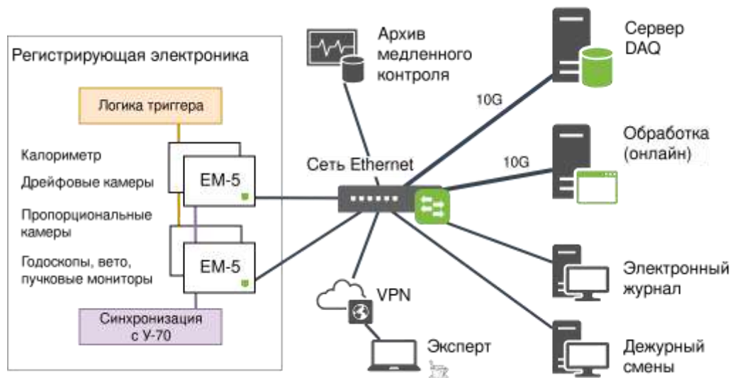
Рис. 3.46 Сеть системы сбора данных установки
