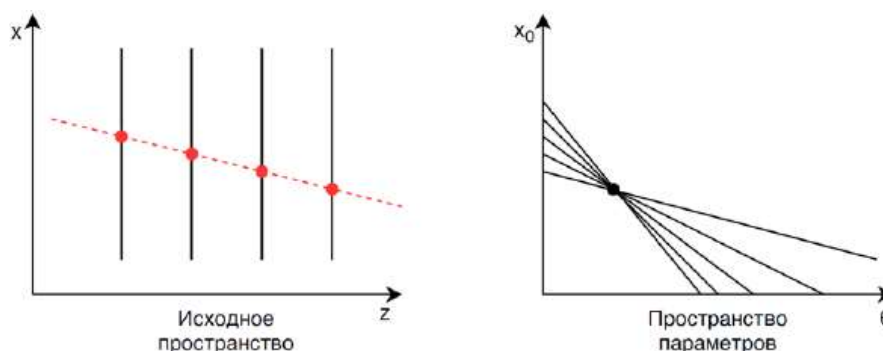
Рис. 3.57 Иллюстрация основного принципа преобразования Хафа для одного трека
