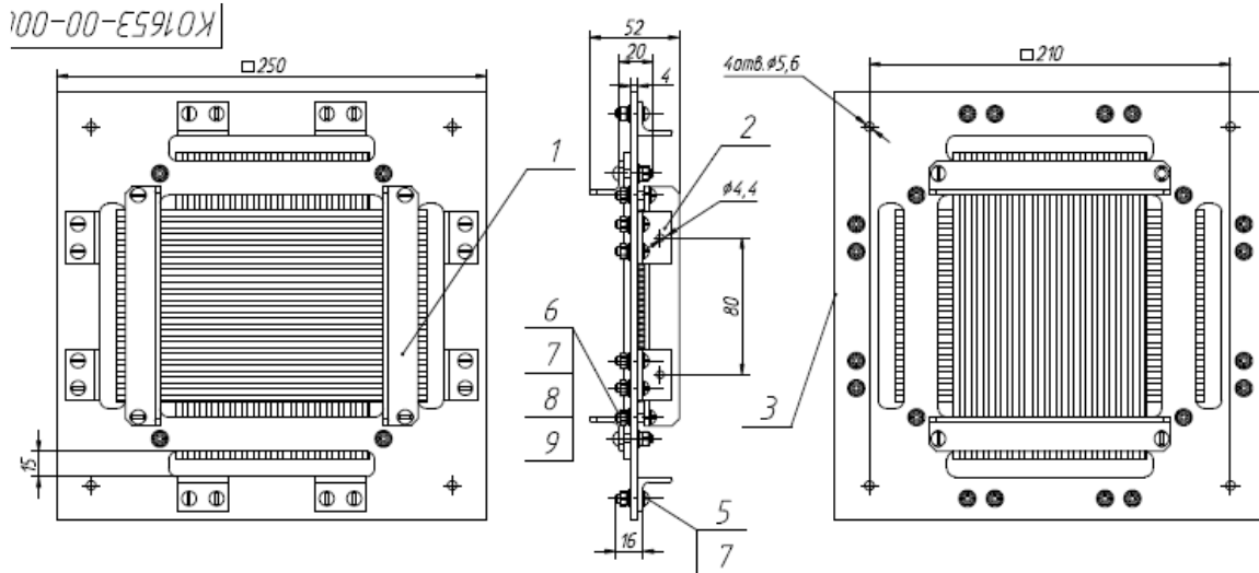
Рис. 2.15 Рама двухкоординатного годоскопа на 32 канала по каждой координате
