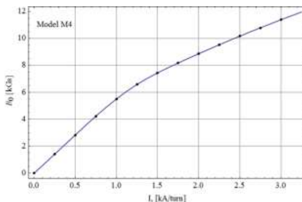
Рис. 3.21 Нагрузочная кривая для модели спектрометрического магнита М31
