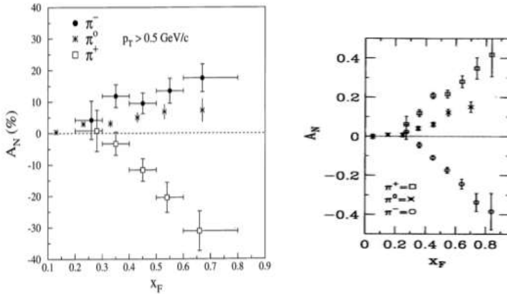
Рис. 1.7 Слева A_N в \bar{p}p -взаимодействии в инклюзивном рождении заряженных [33] и нейтральных [32] мезонов, справа — аналогичный результат для pp -взаимодействия [26, 32]
