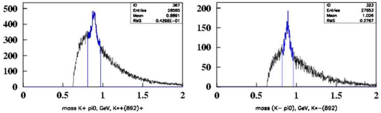
Рис. 6.2 Эффективная масса продуктов распада в процессах \mu p \rightarrow h + X : где h = K^*(892)^+ \rightarrow K^+ \pi^0 (вверху) и h = \bar{K}^*(892)^- \rightarrow K^- \pi^0 (внизу)
