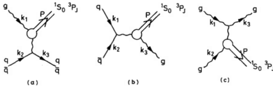
Рис. 1.3 Типичные диаграммы образования кваркония
