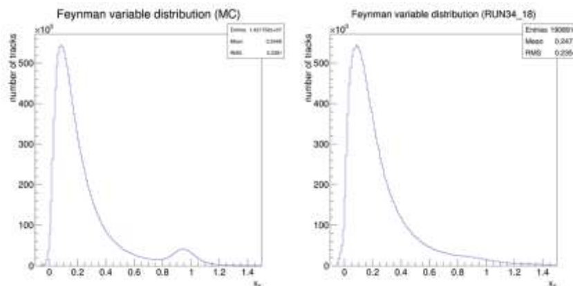
Рис. 3.60 – Распределения по переменной Фейнмана для событий, симулированных методом Монте Карло (слева) и данных эксперимента (справа)
