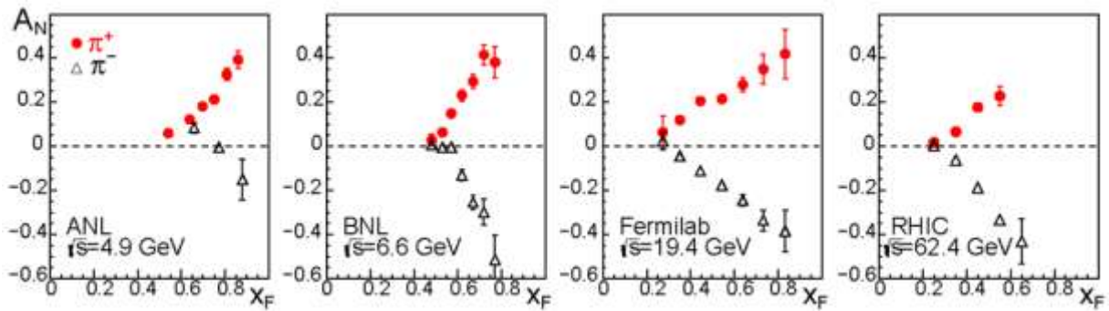
Рис. 1.6 A_N для реакций p\uparrow p \rightarrow \pi^+ + X . Данные ZGS [24], AGS [25], FNAL [26], RHIC [27]. Компиляция экспериментальных данных из публикации [31]
