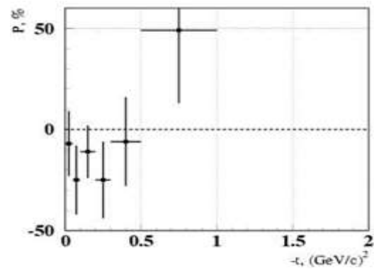
Рис. 1.15 Асимметрия в реакции \pi p^{\uparrow} \rightarrow \eta'(958)n при энергии 40 ГэВ [60], \eta' -мезон регистрировался в моде распада на два \gamma -кванта
