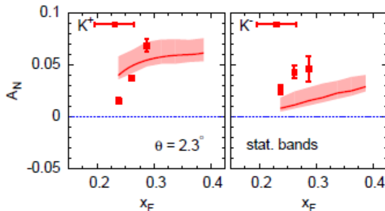
Рис. 5.17 Зависимость A_N(x_F) для K^\pm , из работы [176]
