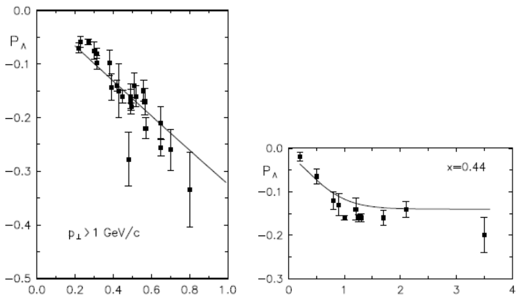
Рис. 5.24 P_N(x_F) для pp \rightarrow \Lambda^+ X (слева) и P_N(p_T) для pp(A) \rightarrow \Lambda^+ X (справа) из работы [194]
