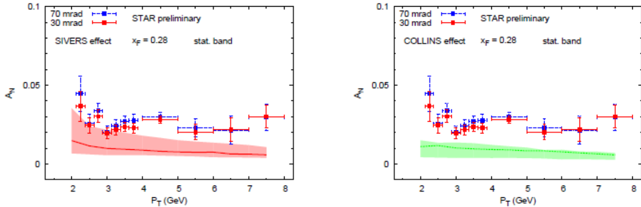
Рис. 5.18 Зависимость A_N(p_T) для реакции p^\uparrow p \rightarrow \pi^0 X , из работы [177], и предсказания в рамках моделей Сиверса (слева) и Коллинза (справа)
