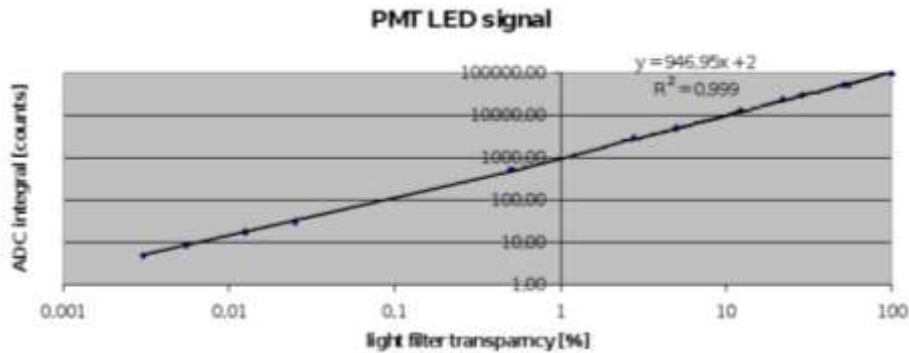
Рис. 3.38 Проверка линейности фотоумножителя
