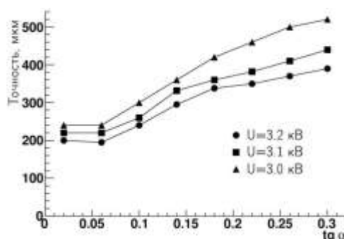
Рис. 3.35 Зависимость точности дрейфовых камер от тангенса угла наклона трека при различных напряжениях на потенциальных проволоочках и фиксированном пороге дискриминации. Угол отсчитывается от нормали к плоскости камеры в плоскости, перпендикулярной направлению проволоочек.
