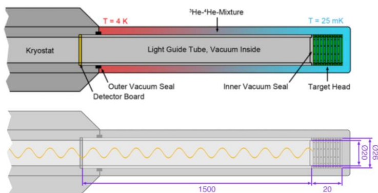
Рис. 3.19 Поляризованная мишень-сцинтиллятор (Майнц)
