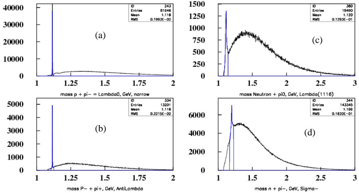
Рис. 6.9 Эффективная масса продуктов распада в процессе K^-p \rightarrow h + X : h = \Lambda \rightarrow p \pi^- (a); h = \tilde{\Lambda} \rightarrow \tilde{p} \pi^+ (b); h = \Lambda \rightarrow n \pi^0 (c); h = \Sigma^- \rightarrow n \pi^- (d)
