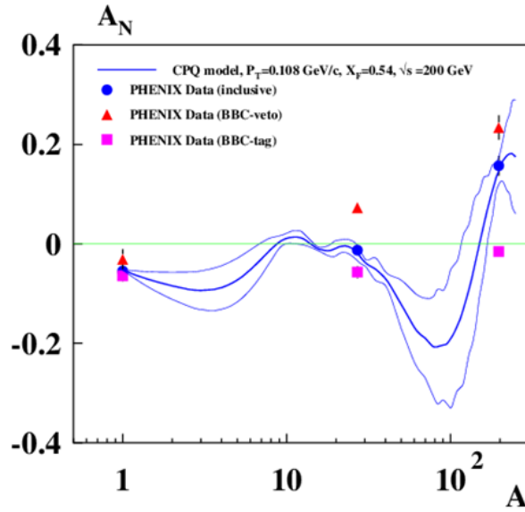
Рис. 1.9 Зависимость A_N(A) для реакции p^\dagger A \rightarrow nX в эксперименте ФЕНИКС [29]
