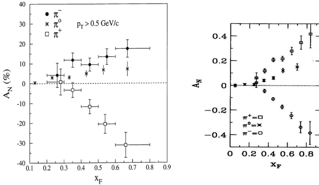
Рис. 1.7 Слева A_N в \bar{p}^1 -взаимодействии в инклюзивном рождении заряженных [33] и нейтральных [32] мезонов, справа — аналогичный результат для pp -взаимодействия [26, 32]
