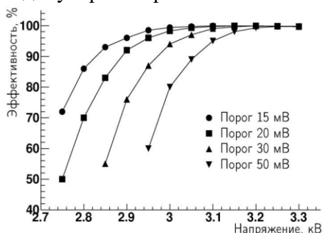
Рис. 3.34 Зависимость эффективности дрейфовой камеры от питающего напряжения при различных порогах дискриминации
