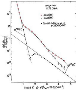
Рис. 5.1 Сечение протон-протонного упругого рассеяния в зависимости от скейлинговой переменной p_T^2 = \beta^2 P_{\perp}^2 \sigma_{tot}(s)/38.3 [139].
