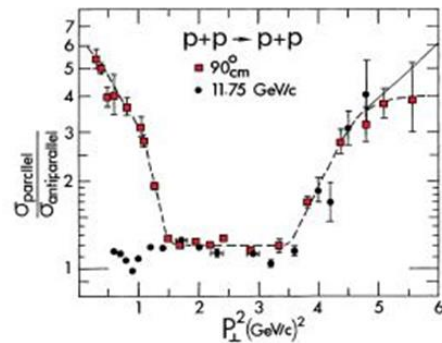
Рис. 5.2 Отношение упругих сечений \sigma^{\uparrow\uparrow}/\sigma^{\downarrow\downarrow} в зависимости от P_{\perp}^2 [140]
