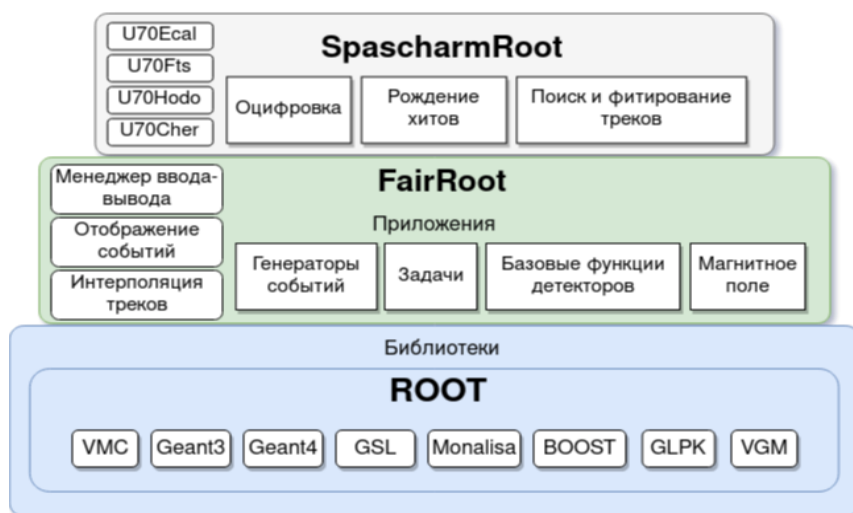
Рис. 3.52 Схематическая структура программной среды эксперимента СПАСЧАРМ: внизу — библиотеки сторонних разработчиков, в центре — среда FairRoot,верху — конкретная реализация SpascharmRoot
