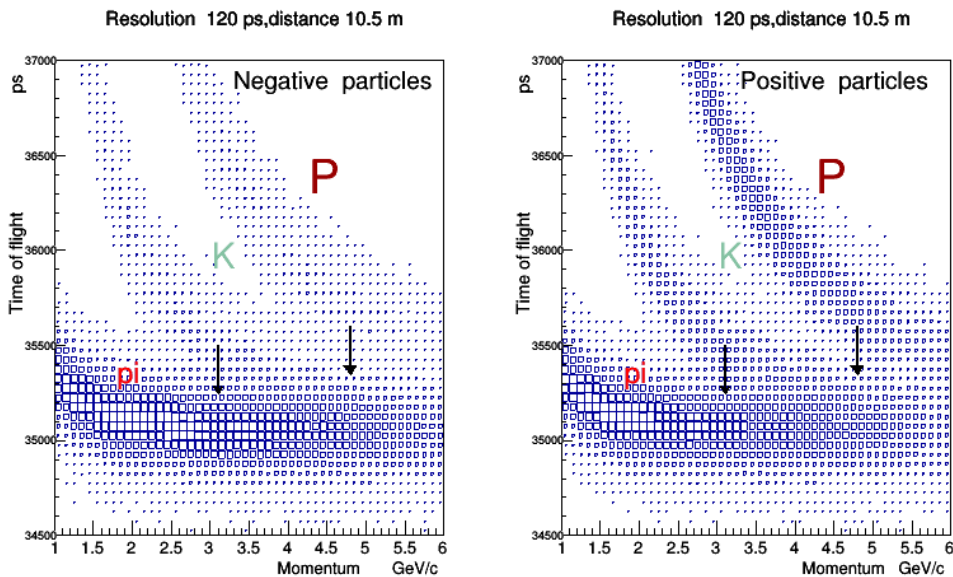
Рис. 3.42 Распределение по квадрату массы M^2 ( \text{ГэВ}^2/c^2 ) в зависимости от импульса частицы при расстоянии 7.6 м от мишени
