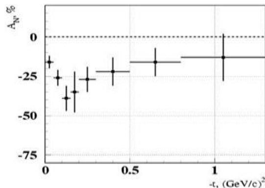
Рис. 5.4 Асимметрия в реакции \pi^- p^{\uparrow} \rightarrow f_2(1270) n при энергии 40 ГэВ [144], когда f_2(1270) -мезон регистрировался в моде распада на два \pi^0 -мезона
