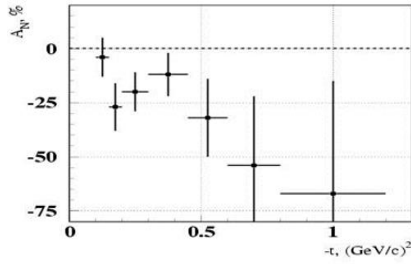
Рис. 1.15 Асимметрия в реакции \pi p^+ \rightarrow \omega(782)n при энергии 40 ГэВ [63], \omega -мезон регистрировался в моде распада на \pi^0 и \gamma
