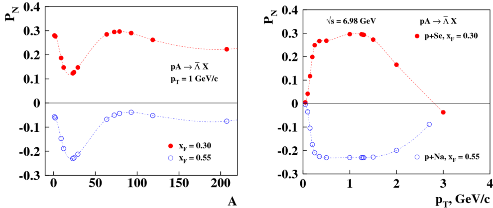
Рис. 1.13 Предсказания поляризации анти-лямбда гиперонов в pA -взаимодействии в рамках модели хромагнитной поляризации кварков
