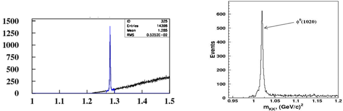
Рис. 1.9 Ожидаемые массовые спектры образования \Xi^- \rightarrow \Lambda \pi^- (слева) и \phi -мезона (справа)
