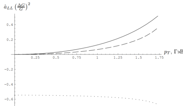
Рис. 1.5 – Зависимость партонных спиновых асимметрий gg \rightarrow \psi g (сплошная линия), gg \rightarrow \chi_{c1} g (пунктирная линия) и gg \rightarrow \chi_{c2} g (точечная линия) от поперечного импульса чармония (рисунок из 22)
