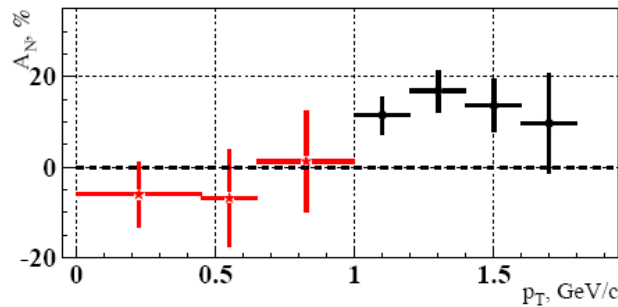
Рис. 1.14 Зависимость A_N(p_T) для реакции \pi^- d_T \rightarrow \pi^0 X при энергии пучка 40 ГэВ в области фрагментации \pi^- -пучка [57] (значение x_F лежит в интервале 0.7 < x_F < 1.0 )
