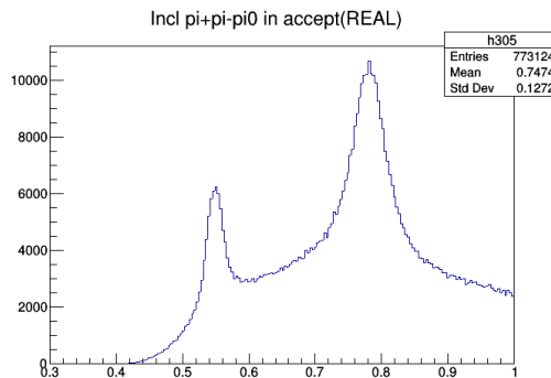
Рис. 1.12 Спектры масс \pi^+ \pi^- \pi^0 (единица измерения ГэВ/ c^2 )
