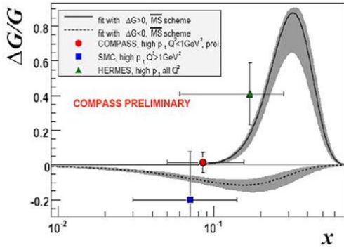
Рис. 1.1 Результат глобального анализа данных [16]
