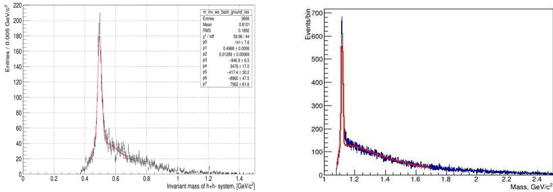
Рис. 1.17 – Массовые спектры h^+h^- пар, полученные при первом анализе данных на пучке \pi^- мезонов (слева) и K^- мезонов (справа)
