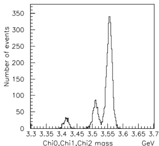
Рис. 1.6 Разделение \chi_{c_j} мезонов на установке СПАСЧАРМ
