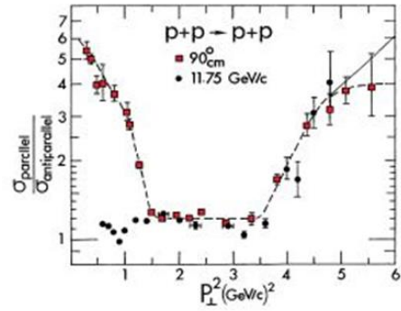
Рис. 5.2 Отношение упругих сечений \sigma^{\uparrow\uparrow}/\sigma^{\uparrow\downarrow} в зависимости от P^2_{\perp} [141]
