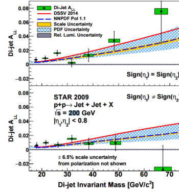
Рис. 1.2 Измерение двухспиновой асимметрии в эксперименте СТАР [17]
