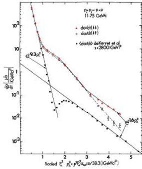
Рис. 5.1 Сечение протон-протонного упругого рассеяния в зависимости от скейлинговой переменной \rho^2_{\perp} = \beta^2 P^2_{\perp} \sigma_{tot}(s)/38.3 [140].
