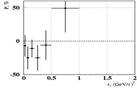
Рис. 1.16 Асимметрия в реакции \pi p^+ \rightarrow \eta'(958)n при энергии 40 ГэВ [61], \eta' -мезон регистрировался в моде распада на два \gamma -кванта
