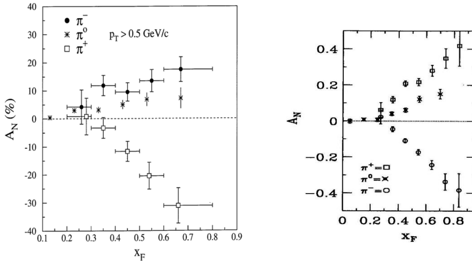
Рис. 1.8 Слева A_N в p\bar{p} -взаимодействии в инклюзивном рождении заряженных [34] и нейтральных [33] мезонов, справа — аналогичный результат для pp -взаимодействия [27, 33]
