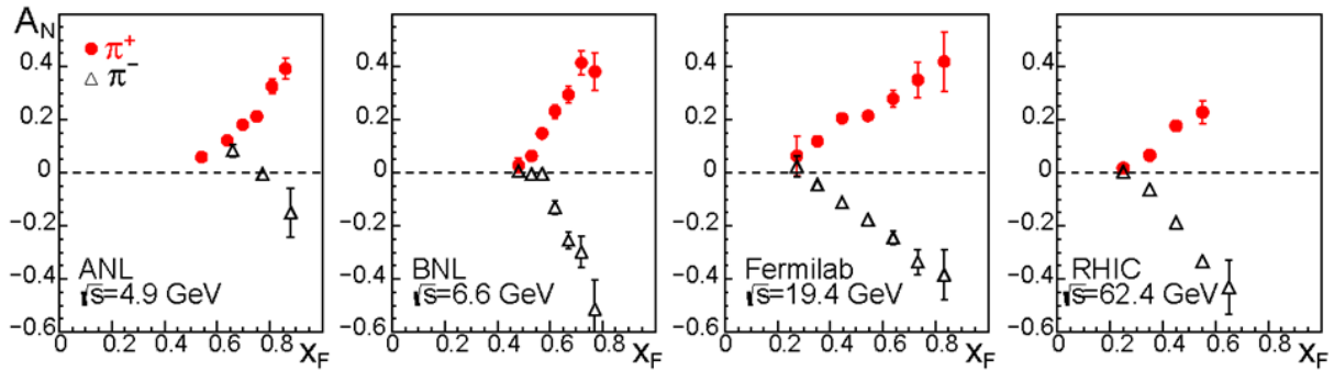
Рис. 1.7 A_N для реакций p\uparrow p \rightarrow \pi^\pm + X . Данные ZGS [25], AGS [26], FNAL [27], RHIC [28]. Компиляция экспериментальных данных из публикации [32]
