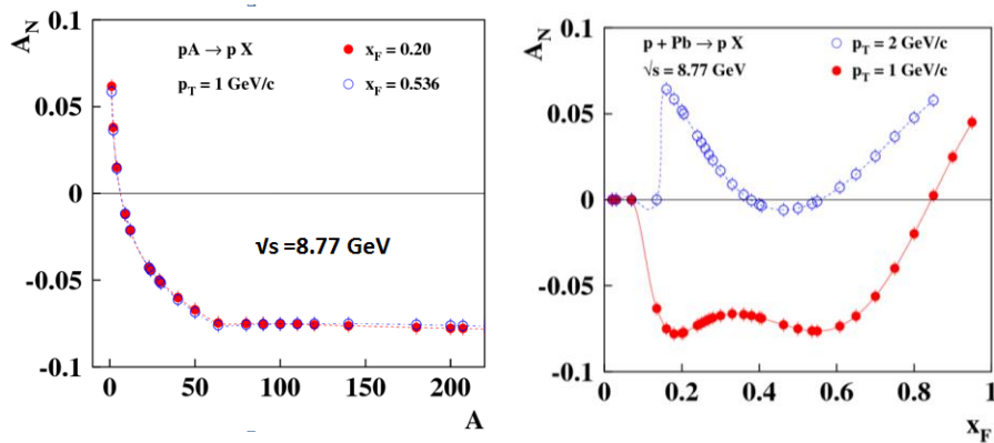
Рис. 1.11 Предсказания A_N в рамках модели хромагнитной поляризации кварков
