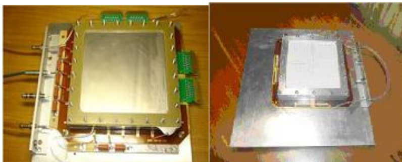
Рис. 3.27 Фотографии двух прототипов GEM детекторов
