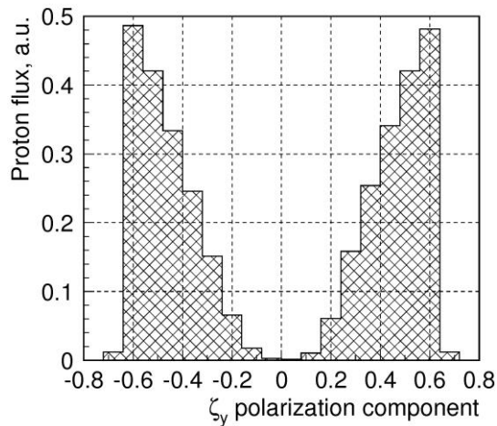
Рис. 2.9 Поляризация протонного пучка с импульсом 45 ГэВ/с на мишени установки для режимов корректора МС2 равных +0.12 Тл×м (слева) и -0.12 Тл×м (справа) при S4 = \pm 15 мм
