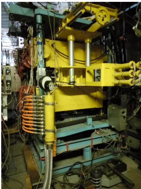
Рис. 3.11 Общий вид магнита ДИНОЗАВР — 2.4 Т с введённой в рабочее положение охранной системой и рабочими коммуникациями на установке СПАСЧАРМ на канале 14 ускорителя У-70
