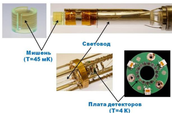
Рис. 3.18 Основные внутренние узлы созданной совместными усилиями (Майнц-Бонн-Бохум-ОИЯИ) мишени-сцинтиллятора
