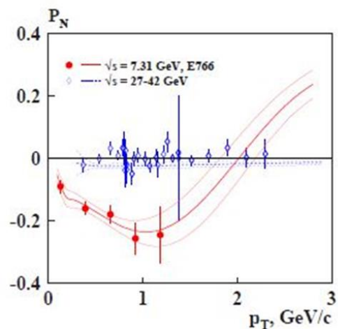
Рис. 5.12 P_N в реакции pA \rightarrow \tilde{\Lambda} + X
