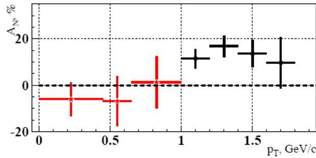
Рис. 1.13 Зависимость A_N(p_T) для реакции \pi d_1 \rightarrow \pi^0 X при энергии пучка 40 ГэВ в области фрагментации \pi^- -пучка [56] (значение x_F лежит в интервале 0.7 < x_F < 1.0 )
