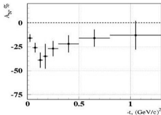
Рис. 5.4 Асимметрия в реакции \pi p^{\uparrow} \rightarrow f_2(1270) n при энергии 40 ГэВ [143], когда f_2(1270) -мезон регистрировался в моде распада на два \pi^0 -мезона
