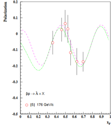
Рис. 5.14 P_N в реакции \bar{p}p \rightarrow \bar{\Lambda} + X
