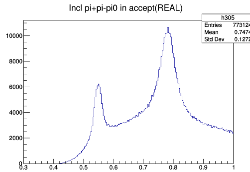
Рис. 1.11 Спектры масс \pi^+ \pi^- \pi^0 (единица измерений ГэВ/с 2 )
