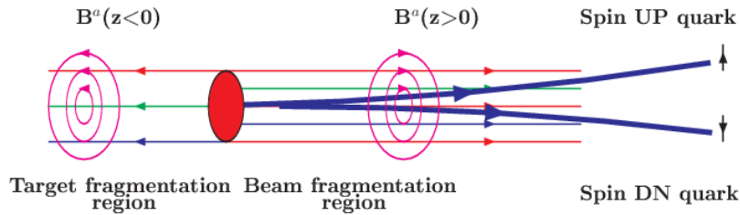
Рис. 5.27 Механизм хромоманнитной поляризации кварков (микроскопический аппарат Штерна-Герлаха). Кварк-пробник отклоняется влево или вправо в неоднородном поле B^a
