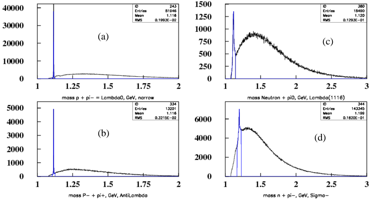
Рис. 6.9 Эффективная масса продуктов распада в процессе K^- p \rightarrow h + X : h = \Lambda \rightarrow p \pi^- (a); h = \tilde{\Lambda} \rightarrow \tilde{p} \pi^+ (b); h = \Lambda \rightarrow n \pi^0 (c); h = \Sigma^- \rightarrow n \pi^- (d)
