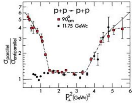
Рис. 5.2 Отношение упругих сечений \sigma^{\uparrow\uparrow}/\sigma^{\downarrow\downarrow} в зависимости от P^2_{\perp} [140]
