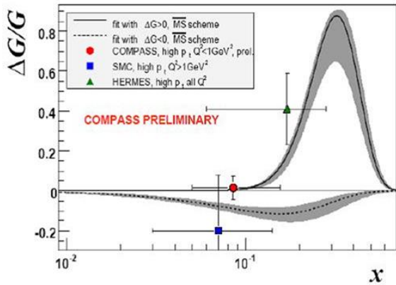
Рис. 1.1 Результат глобального анализа данных [16]
