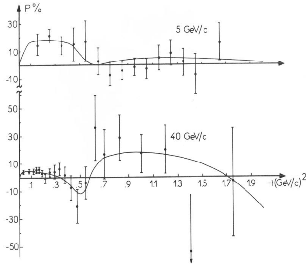
Рис. 5.3 Модель оддерона [142] в применении к описанию поляризации в реакции \pi^- p^{\uparrow} \rightarrow \pi^0 n при импульсах 5 и 40 ГэВ/с [59]
