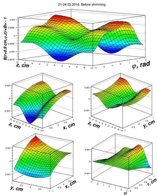
Рис. 3.10 Результаты первоначального измерения поля магнита поляризованной мишени
