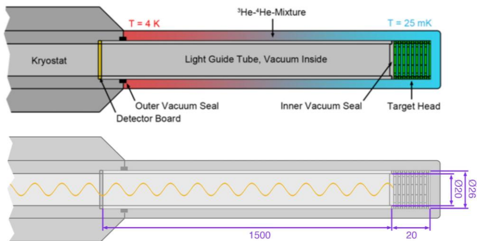
Рис. 3.16 Поляризованная мишень-сцинтиллятор (Майнц)
