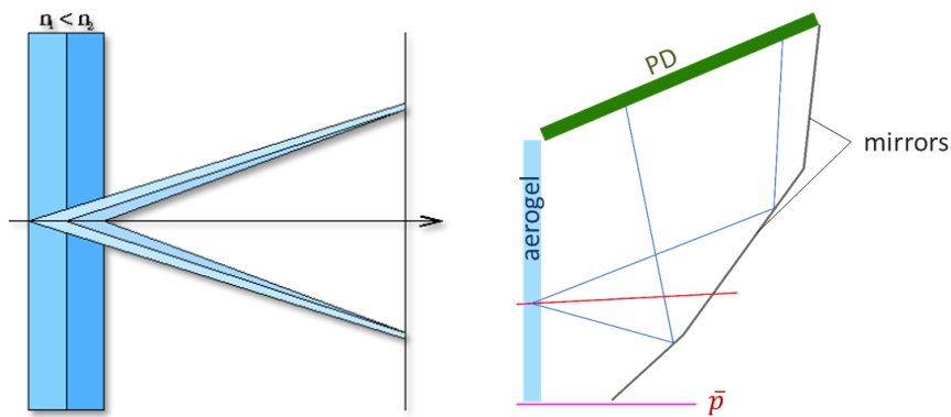
Рис. 3.37 Принцип фокусирования (слева) и принципиальная схема детектора на основе аэрогеля
