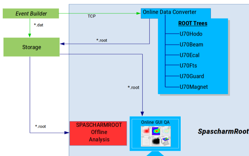
Рис. 3.53 Блок-схема программы обработки данных «в линию»
