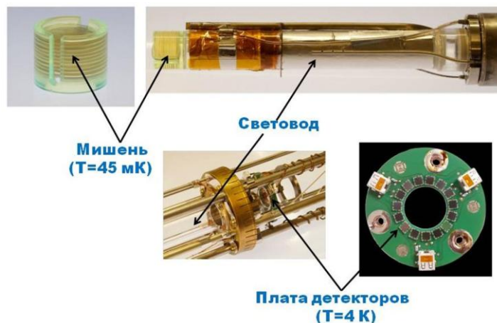
Рис. 3.15 Основные внутренние узлы созданной совместными усилиями (Майнц-Бонн-Бохум-ОИЯИ) мишени-сцинтиллятора
