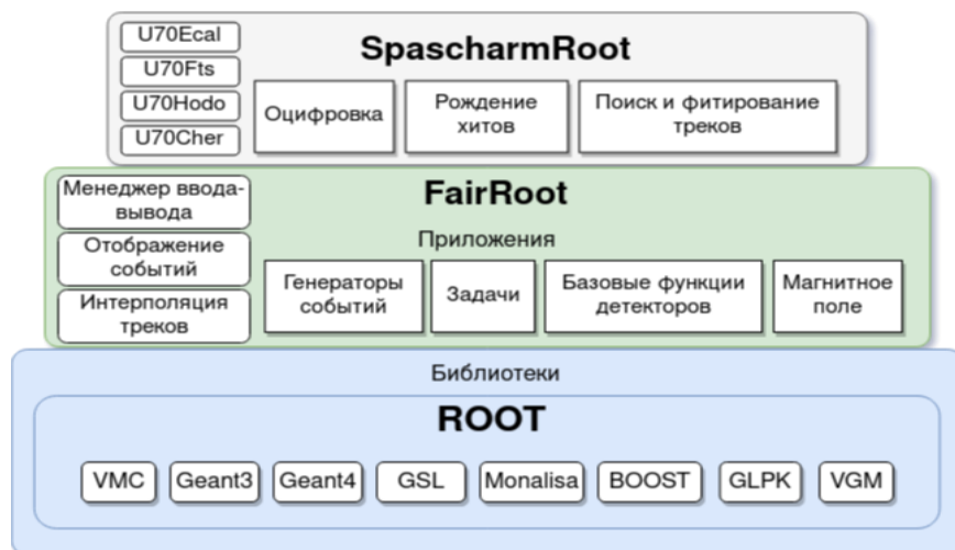
Рис. 3.49 Схематическая структура программной среды эксперимента СПАСЧАРМ: внизу — библиотеки сторонних разработчиков, в центре — среда FairRoot, вверху — конкретная реализация SpascharmRoot
