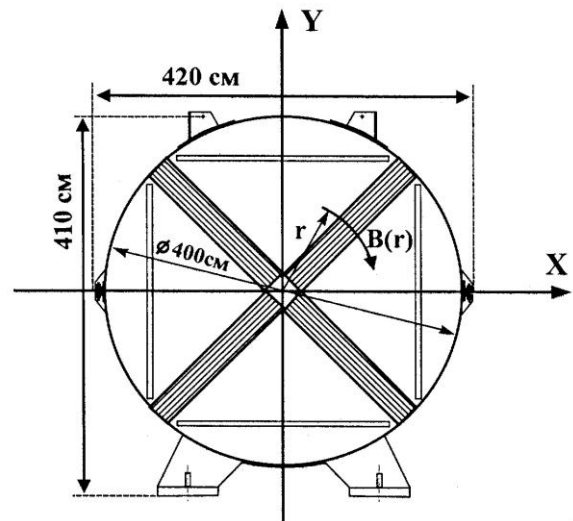
Рис. 3.40 Внешний вид магнита магнитного спектрометра установки «Нейтринный Детектор ИФВЭ-ОИЯИ»
