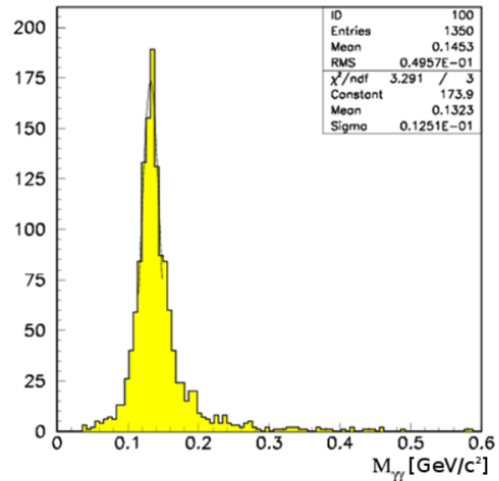
Рис. 3.35 Массовый спектр \pi^0 -мезонов с энергией от 1 до 2 ГэВ (детектор располагался на расстоянии 1.5 м от мишени)
