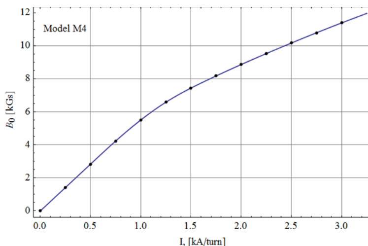
Рис. 3.18 Нагрузочная кривая для модели спектрометрического магнита М31
