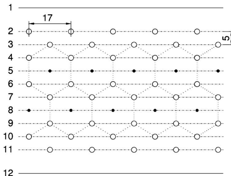
Рис. 3.28 Часть периодической структуры проволочных дрейфовых камер ЭПЕКУР (не в масштабе):
