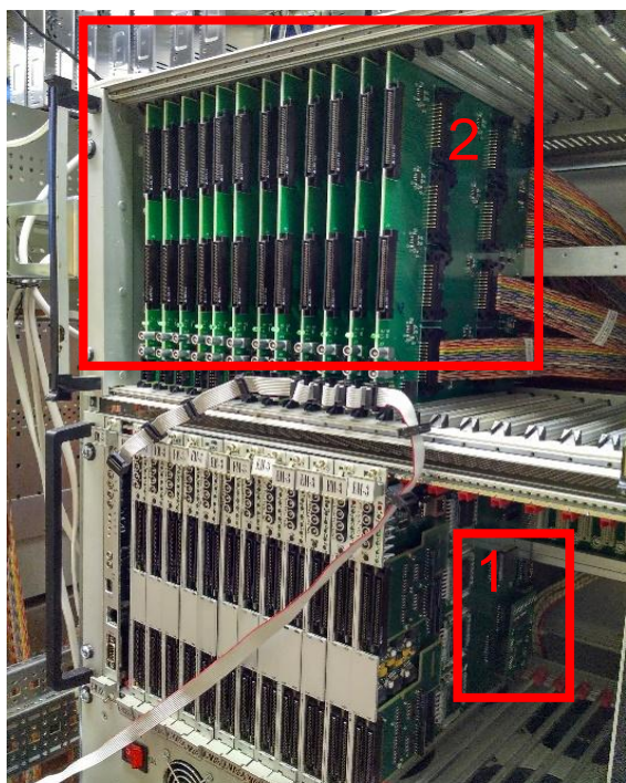
Рис. 3.45 Мезонинная плата, установленная на модуль ЕвроМИСС — 1; переходные платы — 2
