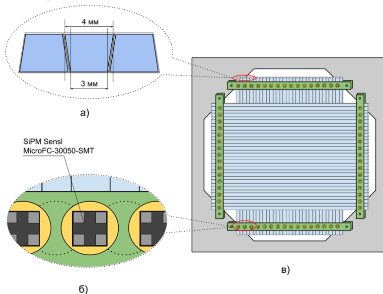
Рис. 2.14. Вариант конструкции однослойного годоскопа системы мечения. а) Вид с торца на сегменты сцинтиллятора. Трапециевидная форма позволяет улучшить эффективность регистрации на границе сегментов. б) Крепление фотодетекторов (кремниевых фотоумножителей) к сегментам сцинтиллятора. в) Общий вид двухкоординатного годоскопа.
