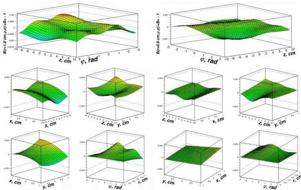
Рис. 3.11 Результаты измерения поля магнита поляризованной мишени после работ в начале 2017 г. (слева) и в настоящее время (справа)
