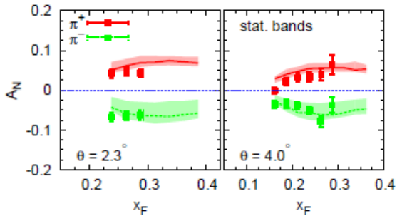
Рис. 5.15 Зависимость A_N(x_F) для p^\uparrow p \rightarrow \pi^\pm X , из работы [166].
