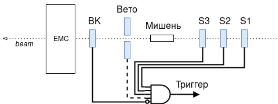
Рис. 3.41 Схема триггера установки
