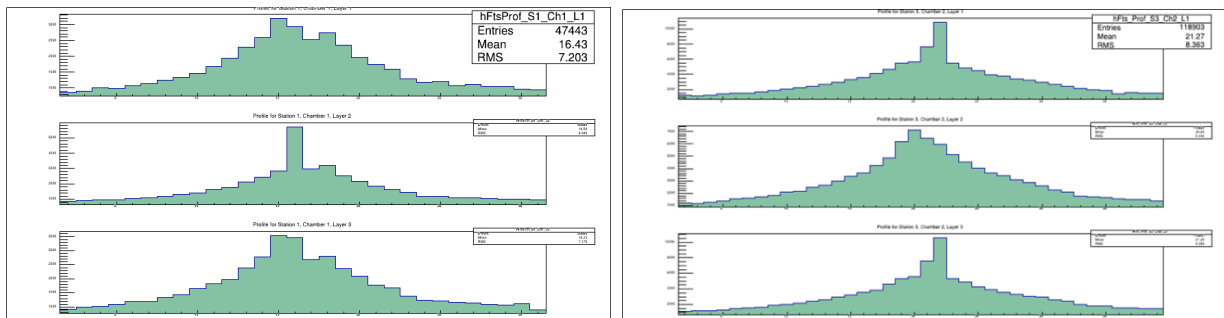
Рис. 3.26 Профили пучка в двух станциях дрейфовых трубок (скриншот программы онлайн-обработки данных)
