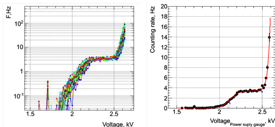
Рис. 3.24 Счетные характеристики всех трубок (слева) и усредненная характеристика всей камеры (справа)
