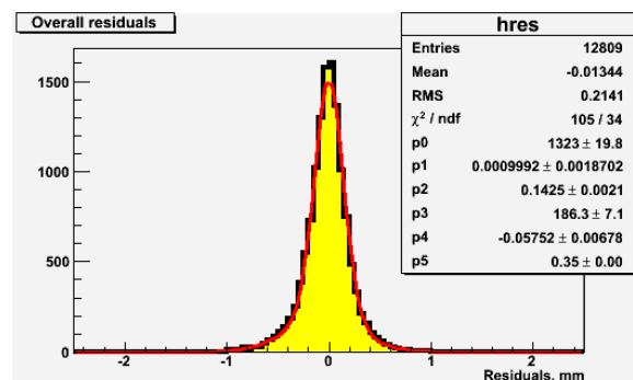
Рис. 3.27 Разность между восстановленной координатой трека и координатой в данной подплоскости
