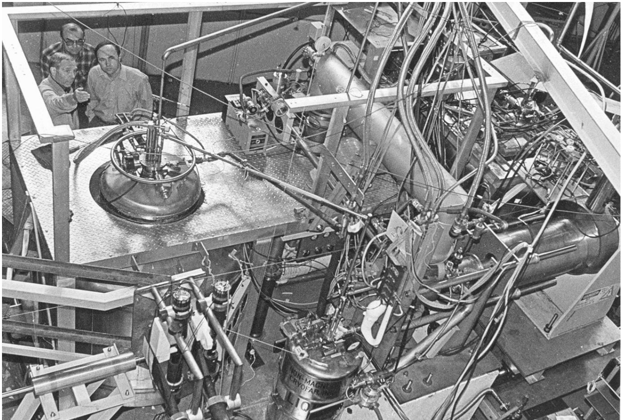
Рис. 3.12 Фотография комплекса продольной поляризованной мишени
