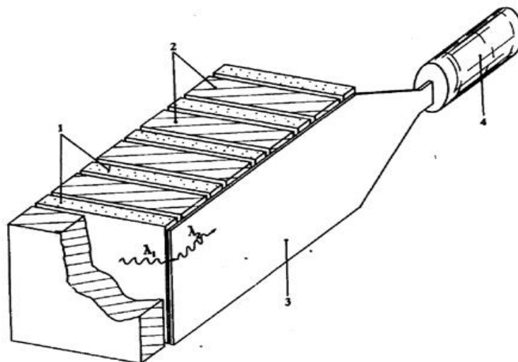
Рис. 3.36 Схематическое изображение модуля адронного калориметра: 1 — сцинтилляционные пластины; 2 — свинцовый поглотитель; 3 — спектростемитель (WLS); 4 — фотоумножитель
