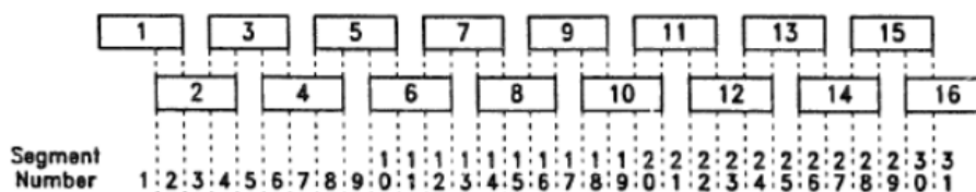
Рис. 2.13 Структура «гребешкового» годоскопа мечения пучка с перекрывающимися сцинтилляторами.
