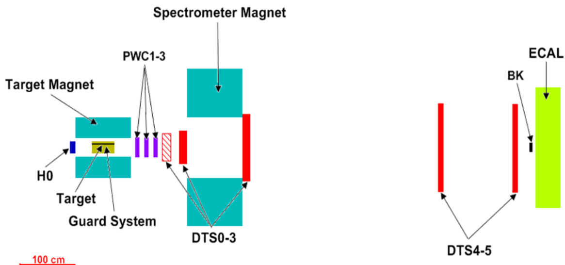
Рис. 3.2 Схема установки СПАСЧАРМ, детекторы показаны не в масштабе (детекторы DTS0-1 соответствуют детекторам DT1-2 при работе на канале 24)
