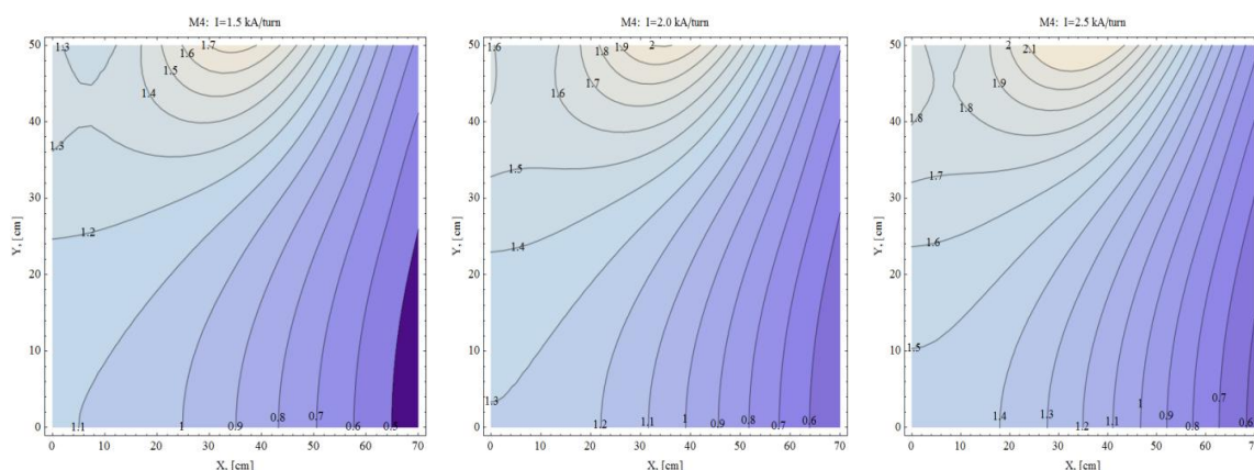
Рис. 3.19 Изолинии интегрального поля в четвертой части рабочей области 700 \times 500 мм 2 . I = 1.5, 2.0 и 2.5 кА/виток
