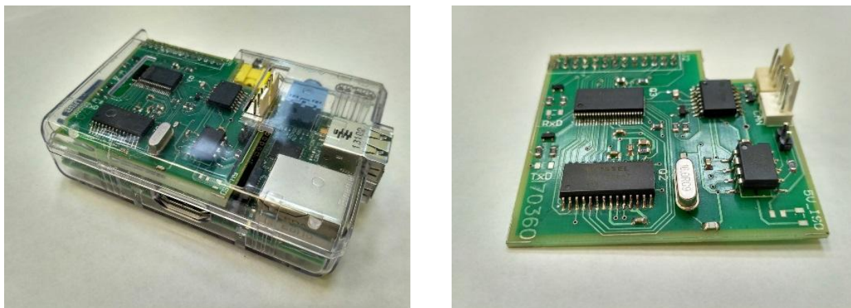
Рис. 3.44 Адаптер шин для Modbus RTU и CAN
