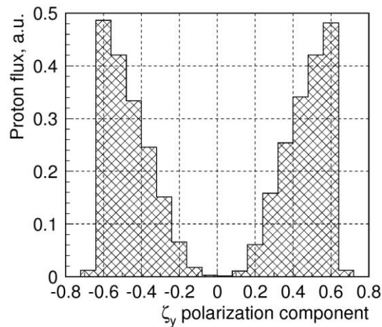
Рис. 2.9 Поляризация протонного пучка с импульсом 45 ГэВ/с на мишени установки для режимов корректора МС2 равных +0.12 \text{ Тл}\times\text{м} (слева) и -0.12 \text{ Тл}\times\text{м} (справа) при C4 = \pm 15 \text{ мм}
