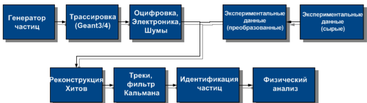
Рис. 3.51 Схематическое представление цепочки выполнения этапов в среде SpascharmRoot
