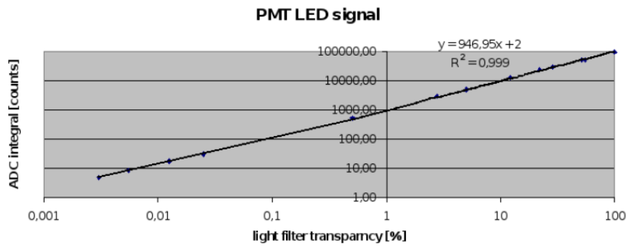
Рис. 3.33 Проверка линейности фотоумножителя
