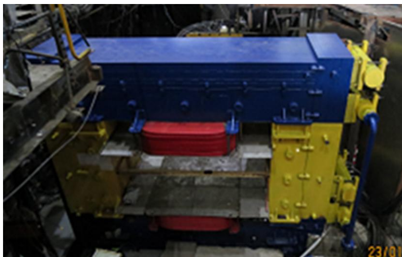
Рис. 3.17 Фотография спектрометрического магнита М31 на канале 14
