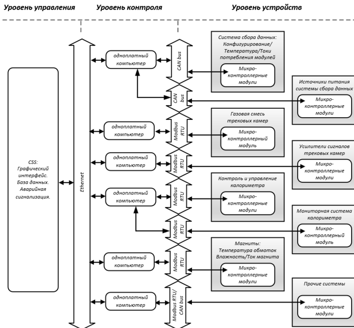
Рис. 3.43 Архитектура системы управления экспериментальной установки СПАСЧАРМ: Control System Studio (CSS)
