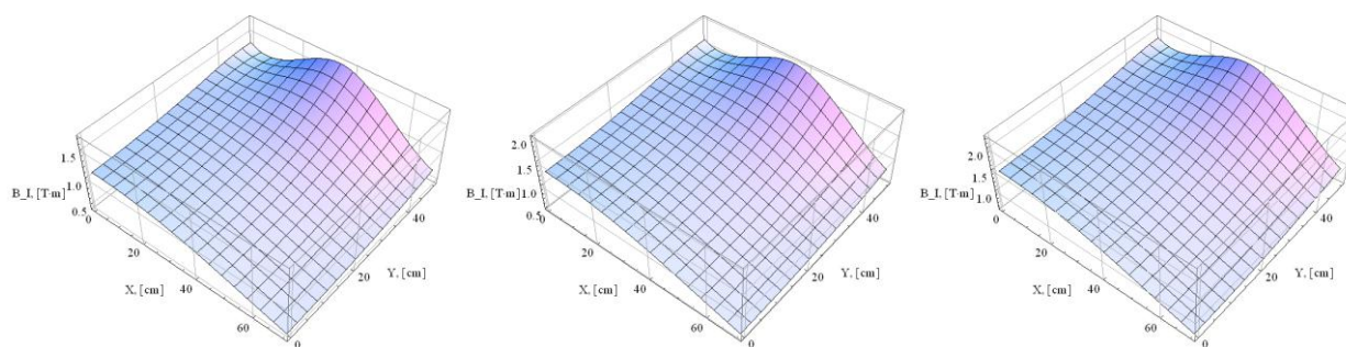
Рис. 3.20 Интегральное поле как функция поперечных координат (X,Y) в рабочей области. I = 1.5, 2.0 и 2.5 кА/виток
