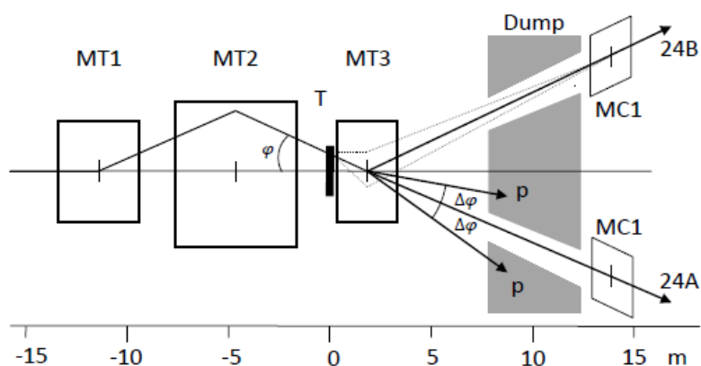
Рис. 2.3 Схема мишенной станции каналов 24А и 24В.
