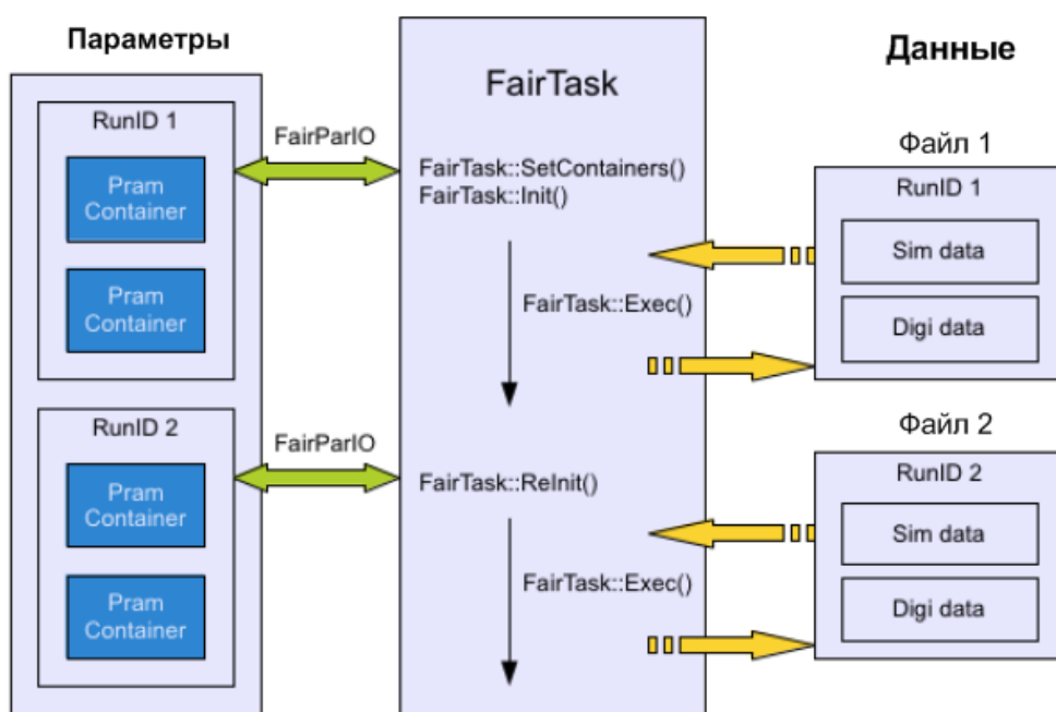
Рис. 3.50 Схематическое представление процессов в FairTask, а также механизма обращения к параметрам и данным. Данные и параметры связаны через уникальный идентификатор “RunID”
