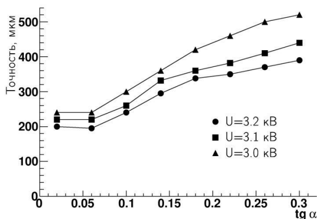
Рис. 3.30 Зависимость точности дрейфовых камер от тангенса угла наклона трека при различных напряжениях на потенциальных проволочках и фиксированном пороге дискриминации. Угол отсчитывается от нормали к плоскости камеры в плоскости, перпендикулярной направлению проволочек.
