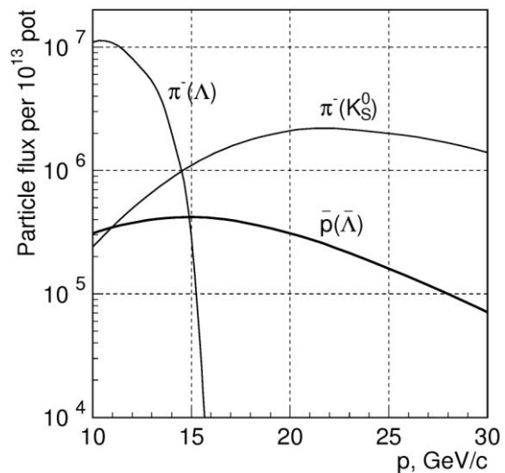
Рис. 2.10 Интенсивность пучка поляризованных антипротонов и фоновых \pi^- -мезонов в конце канала при максимальном \Delta p/p , рассчитанная на 10^{13} падающих на мишень протонов с энергией 60 ГэВ
