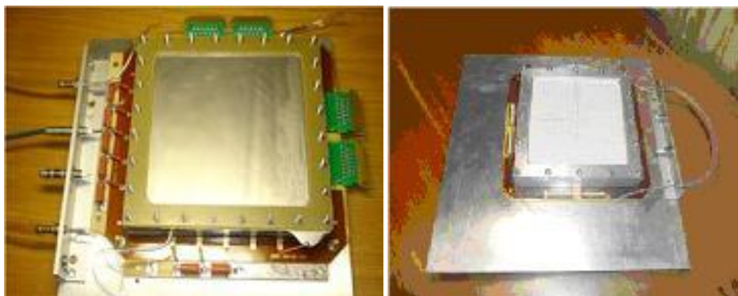
Рис. 3.22 Фотографии двух прототипов GEM детекторов
