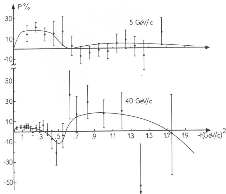
Рис. 5.3 Модель оддерона [131] в применении к описанию поляризации в реакции \pi^- p^\uparrow \rightarrow \pi^0 n при импульсах 5 и 40 ГэВ/с [53]
