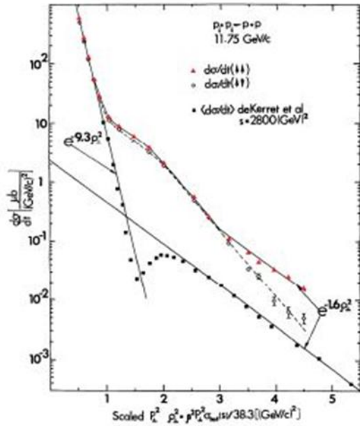
Рис. 5.1 Сечение протон-протонного упругого рассеяния в зависимости от скейлинговой переменной p_{\perp}^2 = \beta^2 P_{\perp}^2 \sigma_{tot}(s)/38.3 [128].
