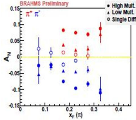
Рис. 5.8 Зависимость A_N(x_F) для реакции p \uparrow p \rightarrow \pi^\pm + X в эксперименте BRAHMS [30]
