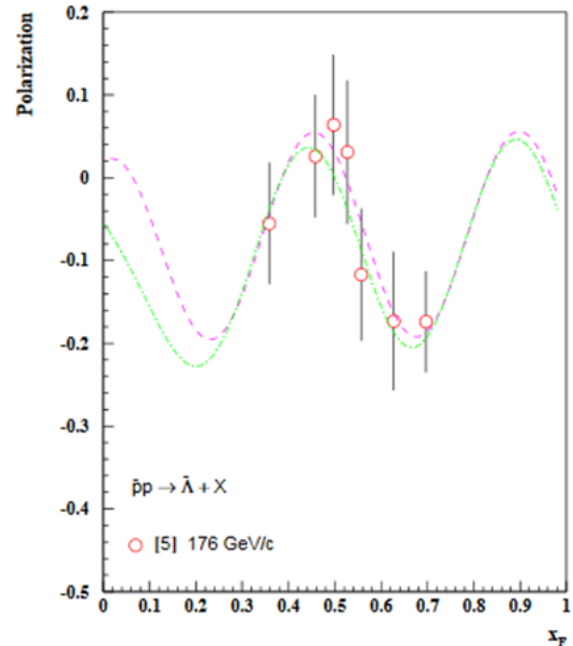
Рис. 5.14 P_N в реакции \bar{p}p \rightarrow \bar{\Lambda} + X
