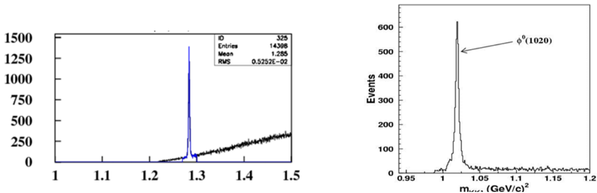
Рис. 1.8 Ожидаемые массовые спектры образования \Xi^- \rightarrow \Lambda \pi^- (слева) и \phi -мезона (справа)
