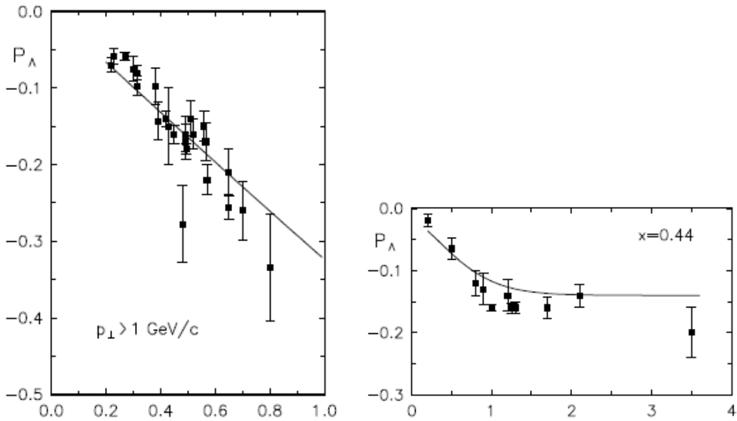
Рис. 5.24 P_N(x_F) для pp \rightarrow L^1 X (слева) и P_N(p_T) для pp(A) \rightarrow L^1 X (справа) из работы [183]
