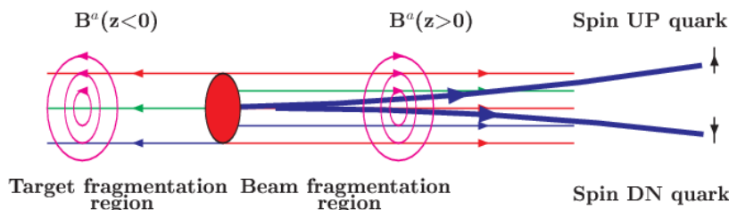
Рис. 5.27 Механизм хромагнитной поляризации кварков (микроскопический аппарат Штерна-Герлаха). Кварк-пробник отклоняется влево или вправо в неоднородном поле B^a
