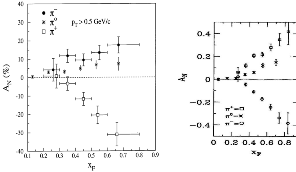
Рис. 1.7 Слева A_N в p\bar{p} -взаимодействии в рождении заряженных [30] и нейтральных [29] мезонов, справа — аналогичный результат для pp -взаимодействии [23, 29]
