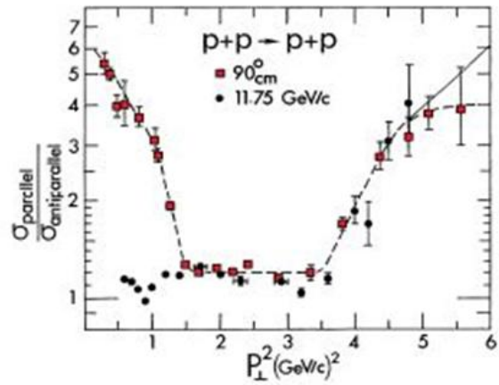
Рис. 5.2 Отношение упругих сечений \sigma^{\uparrow\uparrow}/\sigma^{\downarrow\downarrow} в зависимости от P_{\perp}^2 [129]
