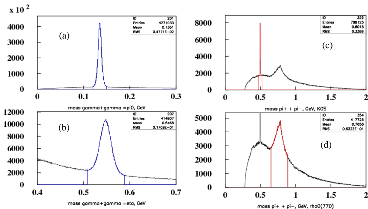
Рис. 6.4. Эффективная масса продуктов распада в процессе \pi^- p \rightarrow h + X , где h = \pi^0 \rightarrow \gamma\gamma (a); h = \eta \rightarrow \gamma\gamma (b); h = K^0_S \rightarrow \pi^+ \pi^- (c); h = \rho^0(770) \rightarrow \pi^+ \pi^- (d)
