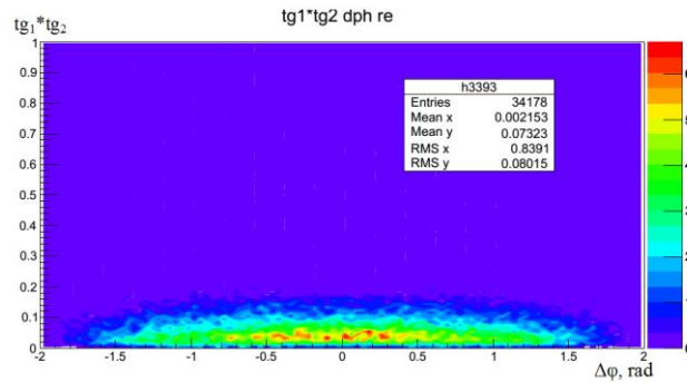
Рис. 2.24 То же, что и на предыдущем рисунке, но только для дифракционных процессов
