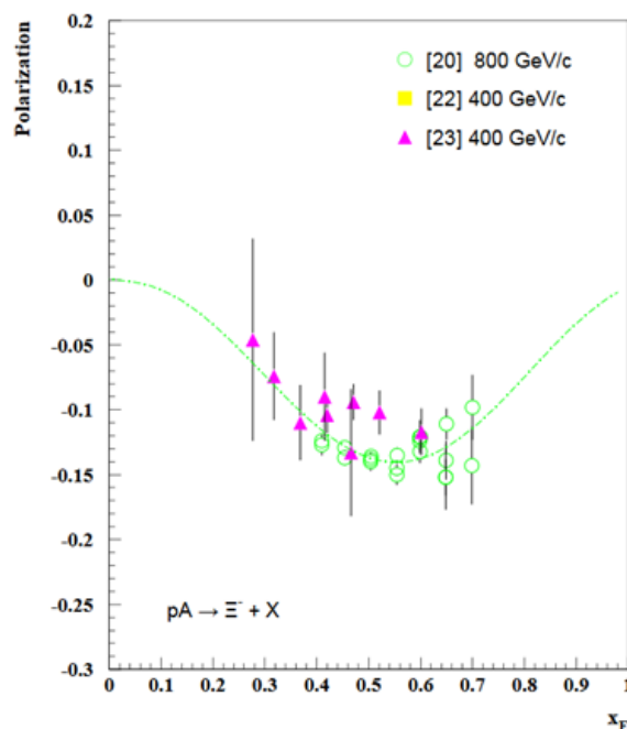
Рис. 5.10 P_N в реакции pA \rightarrow \Xi + X
