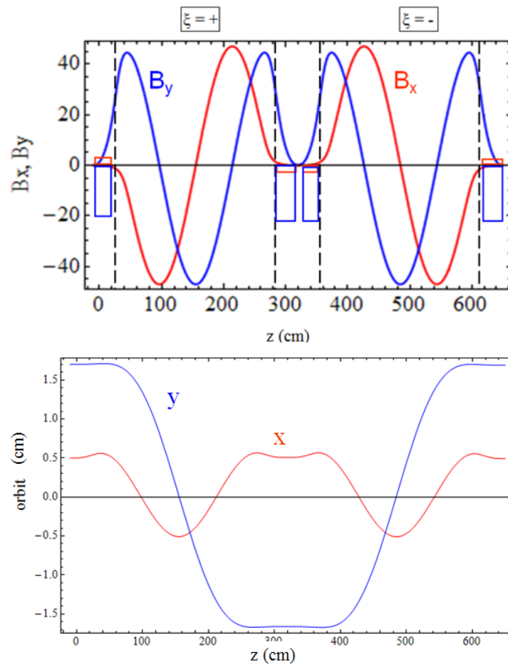
Рис. 2.27 Магнитное поле двух геликоидальных магнитов и траектория частиц внутри змейки при единичной матрице
