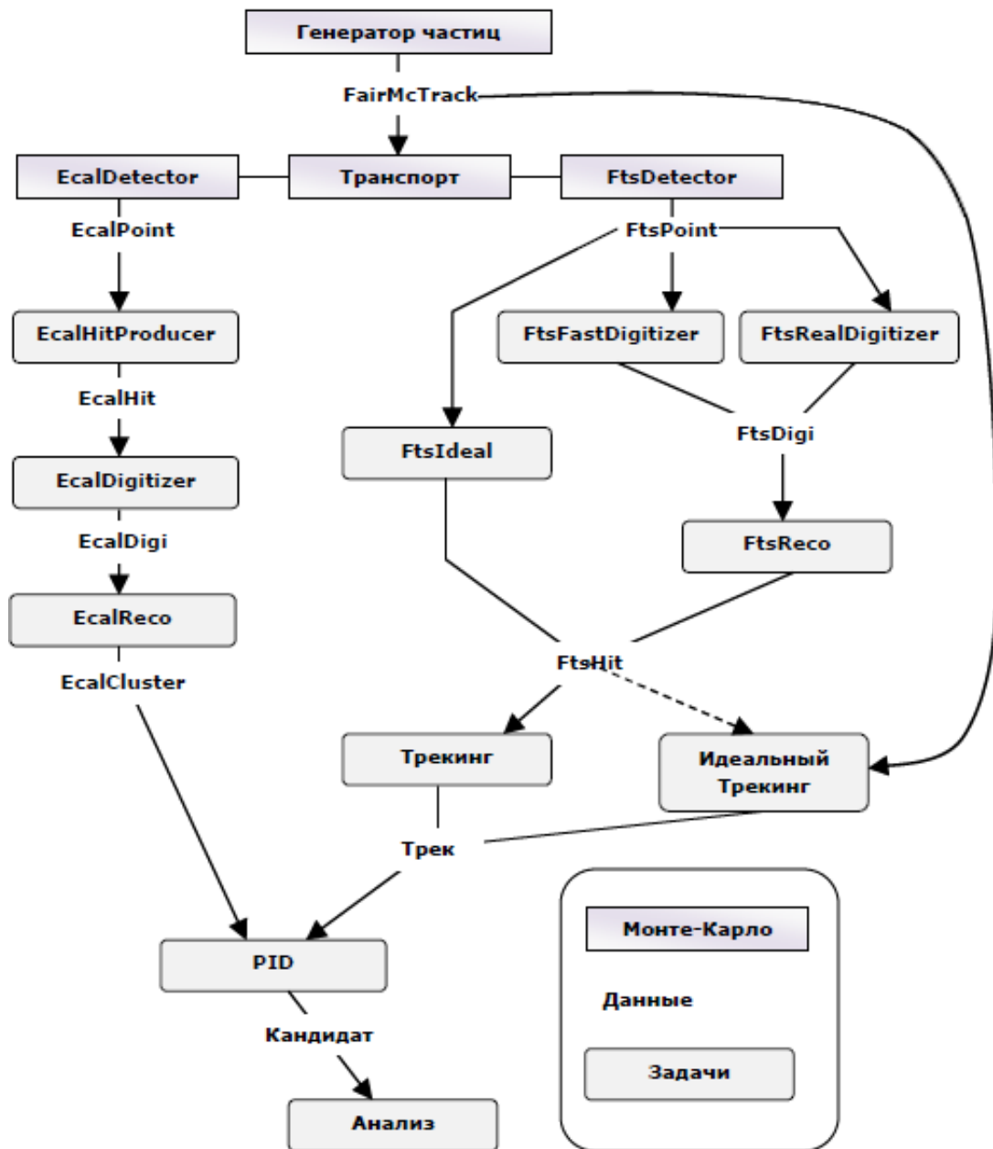
Рис. 3.52 Последовательность выполнения задач TTask при моделировании в среде SpascharmRoot, на примере детектора, идентифицирующего частицы (калориметр или ECAL), и трекового детектора (система станций дрейфовых трубок или FTS). Модульная архитектура программной среды позволяет подключать компоненты, необходимые для конкретного случая
