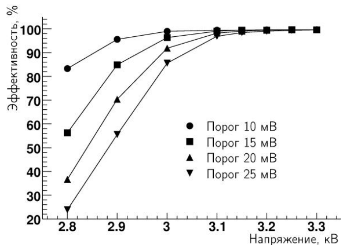
Рис. 3.4 Зависимость эффективности пропорциональной камеры от напряжения на потенциальных плоскостях при различных порогах дискриминации
