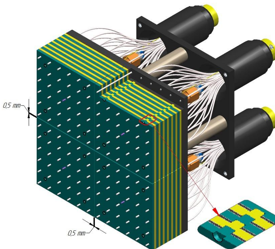
Рис. 3.32 Часть модуля калориметра в разрезе
