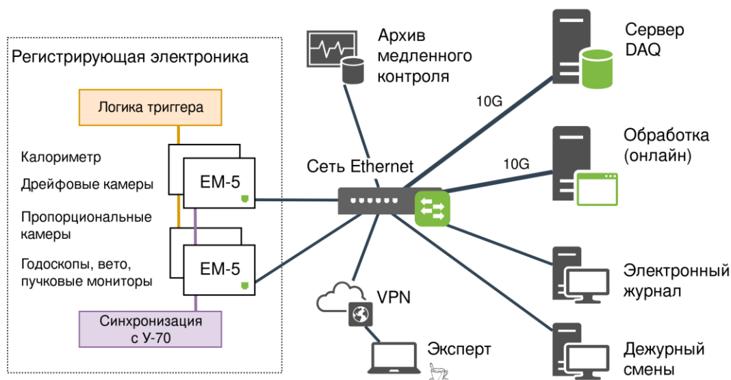
Рис. 3.42 Сеть системы сбора данных установки
