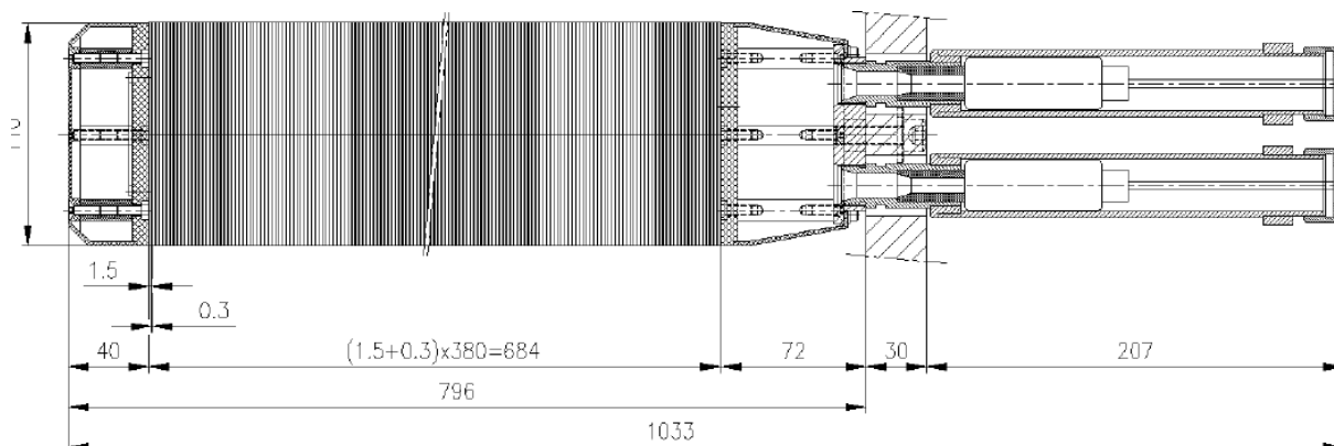
Рис. 3.31 Чертеж супермодуля калориметра
