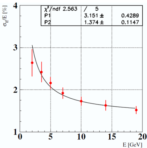
Рис. 3.34 Результаты измерения прототипа калориметра в ИФВЭ
