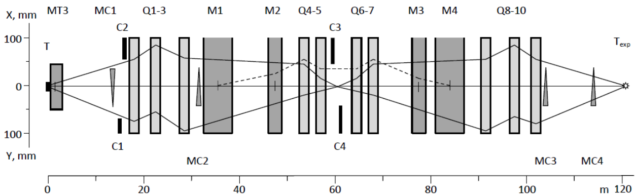
Рис. 2.5 Базовая оптическая схема канала 24А, предназначенная для формирования пучков поляризованных протонов и антипротонов от распада \Lambda(\bar{\Lambda}) -гиперонов: Q — квадрупольные линзы, M — дипольные магниты, C — коллиматоры, MC — магниты-корректоры, T и T_{\text{exp}} — мишени канала и экспериментальной установки. Сплошными линиями показана фокусировка пучка в обеих поперечных плоскостях, пунктиром — дисперсия в горизонтальной плоскости для \Delta p/p = 5\%
