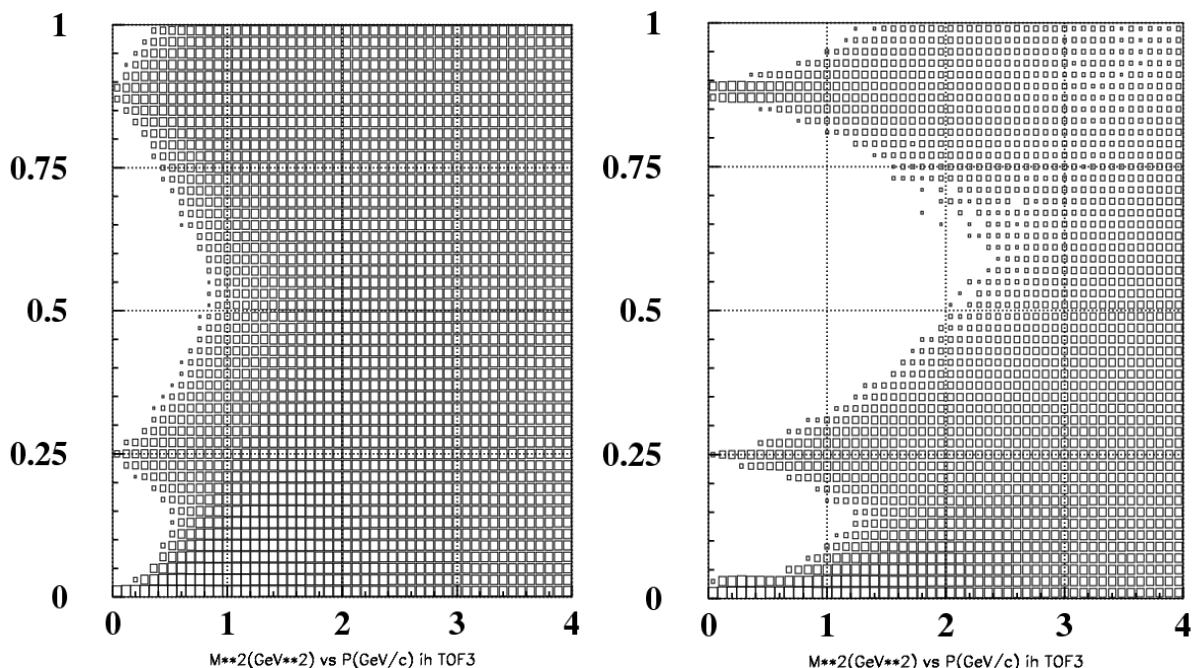
Рис. 3.39 Распределение по квадрату массы M^2 (ГэВ/ c^2 ) в зависимости от импульса частицы при расстоянии 7.6 м от мишени
