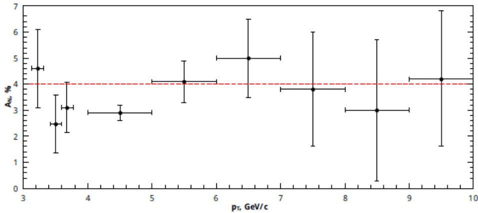
Рис. 5.22 Зависимость A_N(x_F) для p^\uparrow p \rightarrow \pi^0 X , из [178]. Угол изоляции пиона 70 мрад, \sqrt{s} = 500 ГэВ и 0.32 < x_F < 0.40 . Данные STAR из [179, 180]
