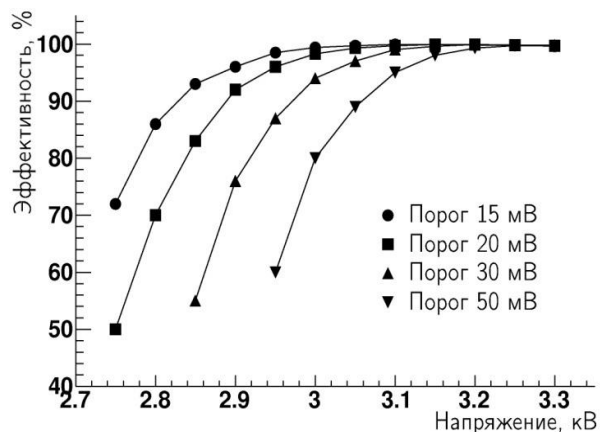
Рис. 3.29 Зависимость эффективности дрейфовой камеры от питающего напряжения при различных порогах дискриминации
