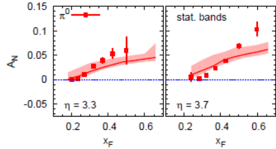
Рис. 5.16 Зависимость A_N(x_F) для p^\uparrow p \rightarrow \pi^0 X , из работы [166].
