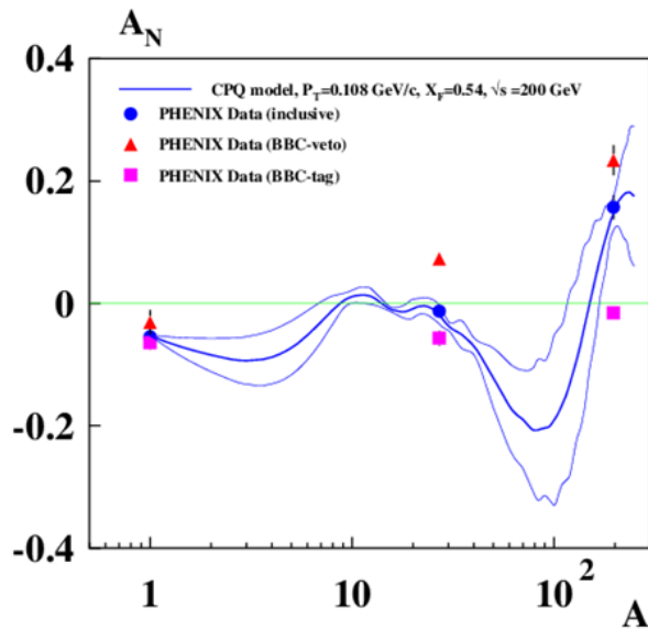
Рис. 1.9 Зависимость A_N(A) для реакции p^+A \rightarrow n+X в эксперименте ФЕНИКС [29]
