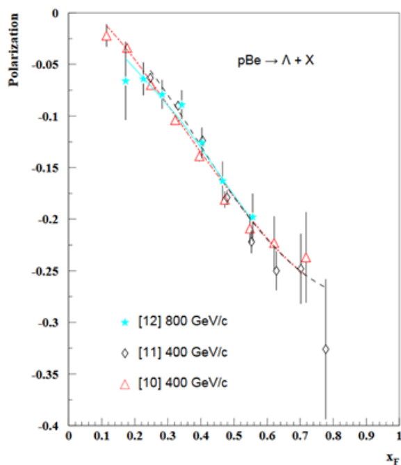
Рис. 5.9 P_N в реакции pBe \rightarrow \Lambda + X
