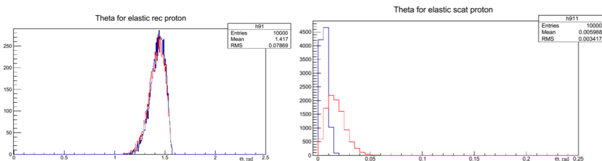
Рис. 2.21 Угловые распределения протонов отдачи (слева) и рассеяния справа для энергий 45 (синий) и 16 ГэВ
