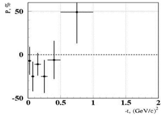
Рис. 1.15 Асимметрия в реакции \pi p^+ \rightarrow \eta'(958)n при энергии 40 ГэВ [132], когда \eta'(958) -мезон регистрировался в режиме распада на два \gamma -кванта
