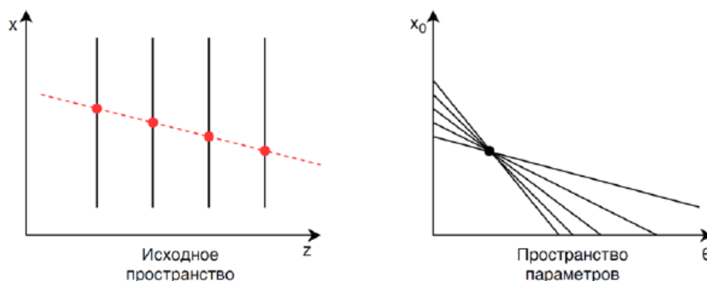
Рис. 3.55 Иллюстрация основного принципа преобразования Хафа для одного трека
