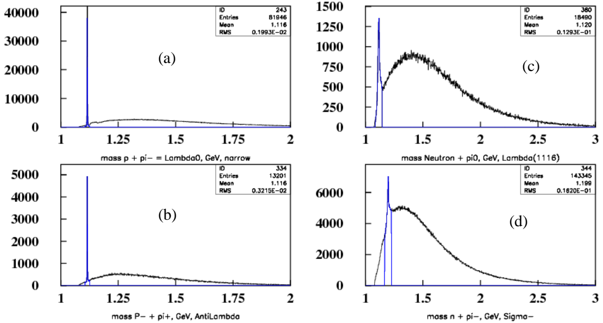
Рис. 6.5 Эффективная масса продуктов распада в процессе K^-p \rightarrow h + X : h = \Lambda \rightarrow p \pi^- (a); h = \tilde{\Lambda} \rightarrow \tilde{p} \pi^+ (b); h = \Lambda \rightarrow n \pi^0 (c); h = \Sigma^- \rightarrow n \pi^- (d)
