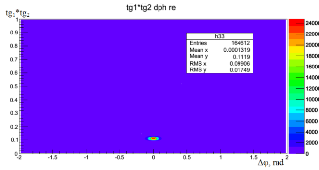
Рис. 2.23 Произведения тангенсов от разницы азимутальных углов (только для упругих процессов с учетом размеров детекторов H3 и H5)
