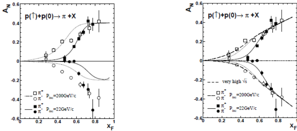
Рис. 5.19 A_N(x_F) для p^\uparrow p \rightarrow \pi^\pm X для разных значений параметров Берлинской модели [172]
