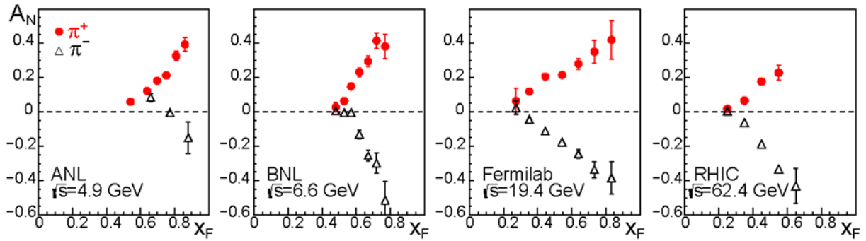
Рис. 1.6 A_N для реакций p^\uparrow p \rightarrow \pi^\pm + X . Данные ZGS [21], AGS [22], FNAL [23], RHIC [24]. Компиляция экспериментальных данных из публикации [28]
