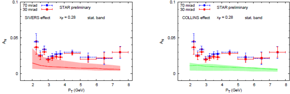
Рис. 5.18 Зависимость A_N(p_T) для реакции p^+p^- \rightarrow \pi^0 X , из работы [166], и предсказания в рамках моделей Сиверса (слева) и Коллинза (справа)
