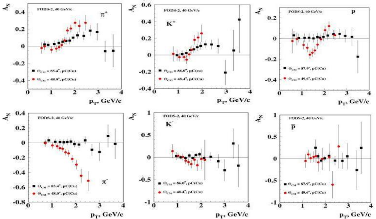
Рис. 5.7 Зависимость A_N(p_T) для процессов инклюзивного образования \pi^\pm , K^\pm , p и \bar{p} в p^+A -соударениях при двух углах рождения адронов и импульсе 40 ГэВ/с
