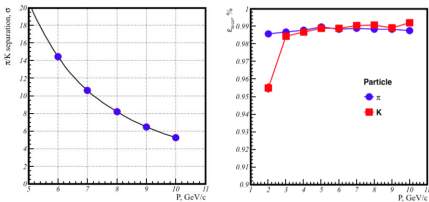
Рис. 3.38 Моделирование разделения мезонов и эффективность их регистрации для детектора ПАНДА
