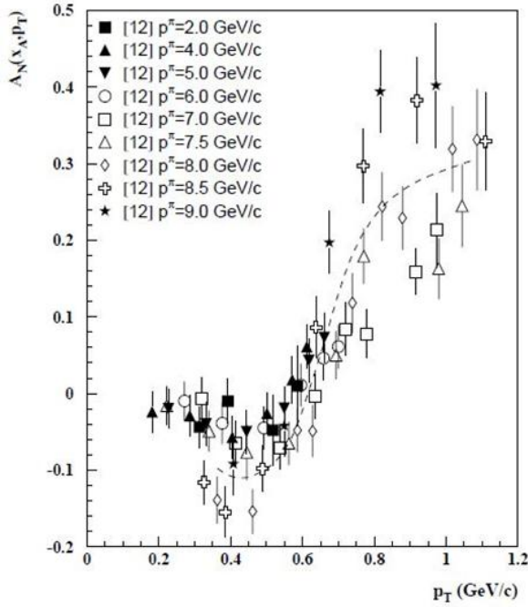
Рис. 5.5 A_N(p_T) для реакции p^+p^- \rightarrow \pi^+ + X
