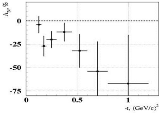
Рис. 1.14 Асимметрия в реакции \pi p^+ \rightarrow \omega(782)n при энергии 40 ГэВ [55], когда \omega(782) -мезон регистрировался в режиме распада на \pi^0 и \gamma
