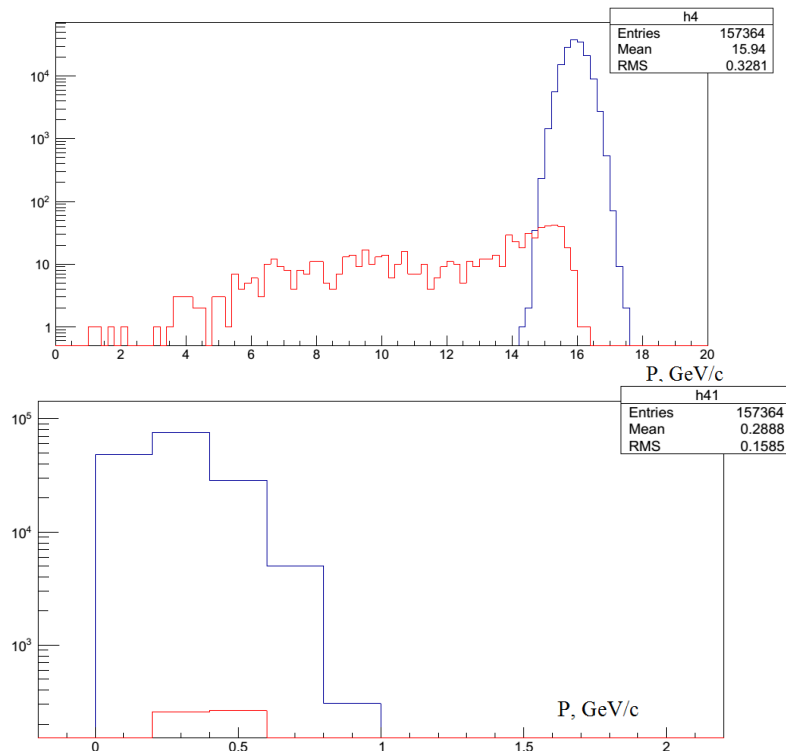
Рис. 2.25 Распределение по импульсу рассеянных частиц (слева) и частиц отдачи (справа) для упругих (синий) и дифракционных (красный) процессов
