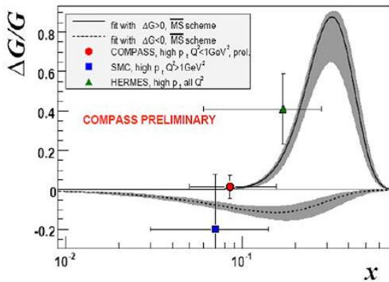
Рис. 1.1 Результат глобального анализа данных [13]
