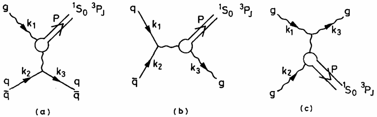
Рис. 1.3 Типичные диаграммы образования кваркония
