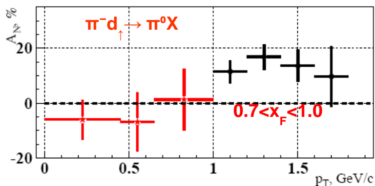
Рис. 1.13 Зависимость A_N(p_T) для реакции \pi^- d \rightarrow \pi^0 X при энергии пучка 40 ГэВ в области фрагментации \pi^- -пучка [50] (значение x_F лежит в интервале 0.7 < x_F < 1.0 )
