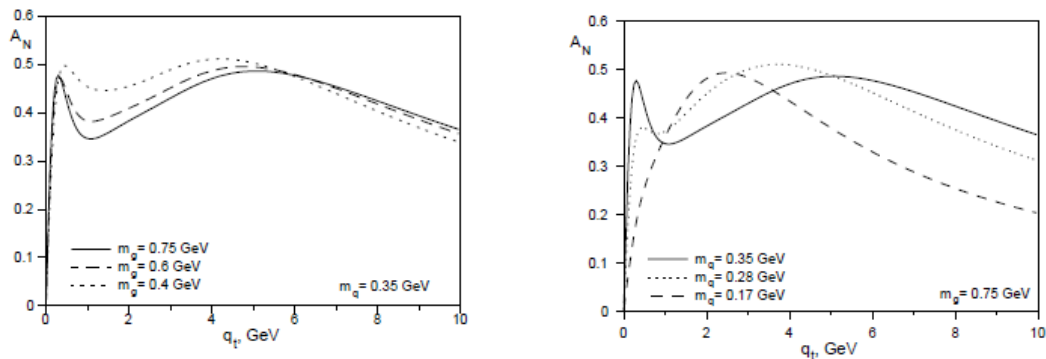
Рис. 5.21 A_N(q_T) для рассеяния кварков, при разных параметрах m_g инфракрасного обрезания (слева) и разных динамических массах кварка (справа) из модели [176]
