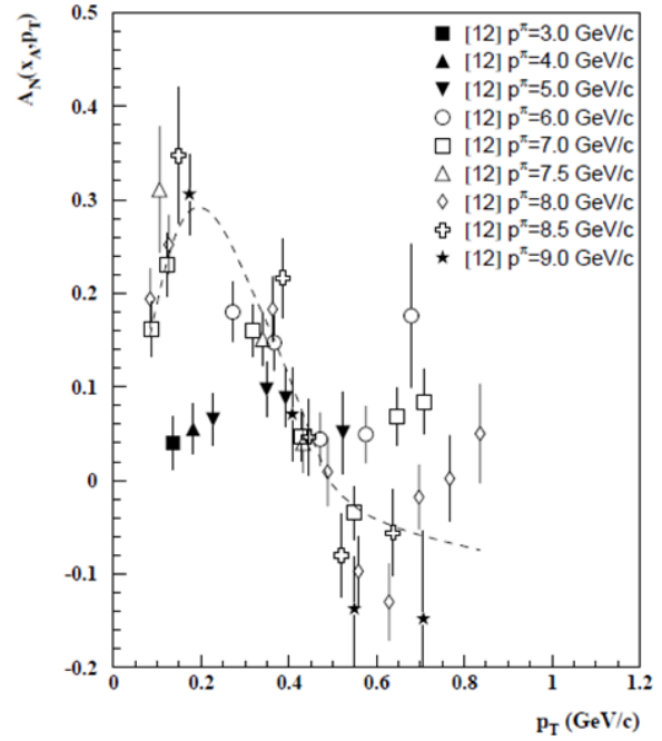
Рис. 5.6 A_N(p_T) для реакции p^+p^- \rightarrow \pi^- + X
