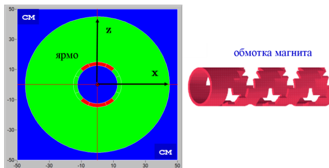
Рис. 2.26 Проект дизайна ярма и обмотки одного геликоидального магнита (на данном рисунке ось z соответствует вертикальному направлению)
