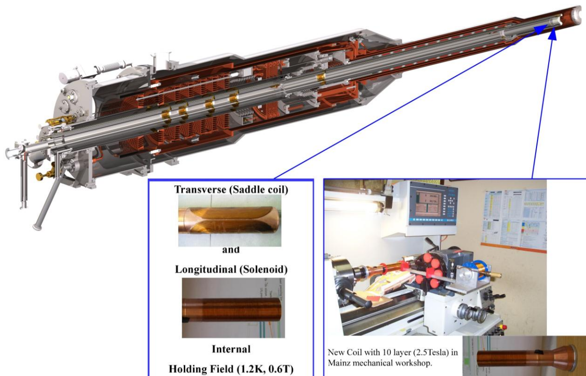
Рис. 3.14 Криостат поляризованной мишени с поляризующей (Saddle coil) и удерживающей поляризацию (Solenoid) сверхпроводящими катушками
