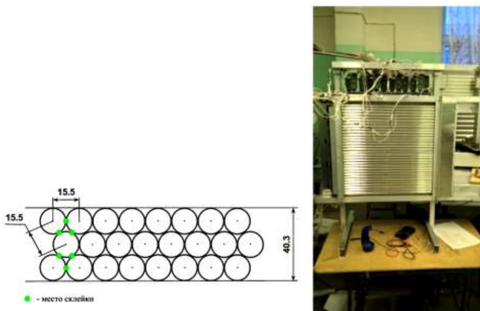
Рис. 3.22 Схема расположения трубок (левая панель) и фото камеры перед установкой на штатное место (правая панель)
