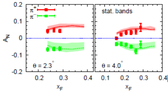
Рис. 5.15 Зависимость A_N(x_F) для p^+p \rightarrow \pi^+X , из работы [166].
