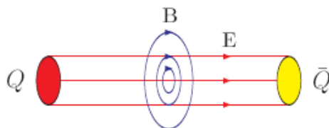
Рис. 5.25 Схематическая картина трубки цветового потока между кварком и антикварком. Продольные линии показывают направление хромоэлектрического поля E , а круговые направление хромомагнитного поля B
