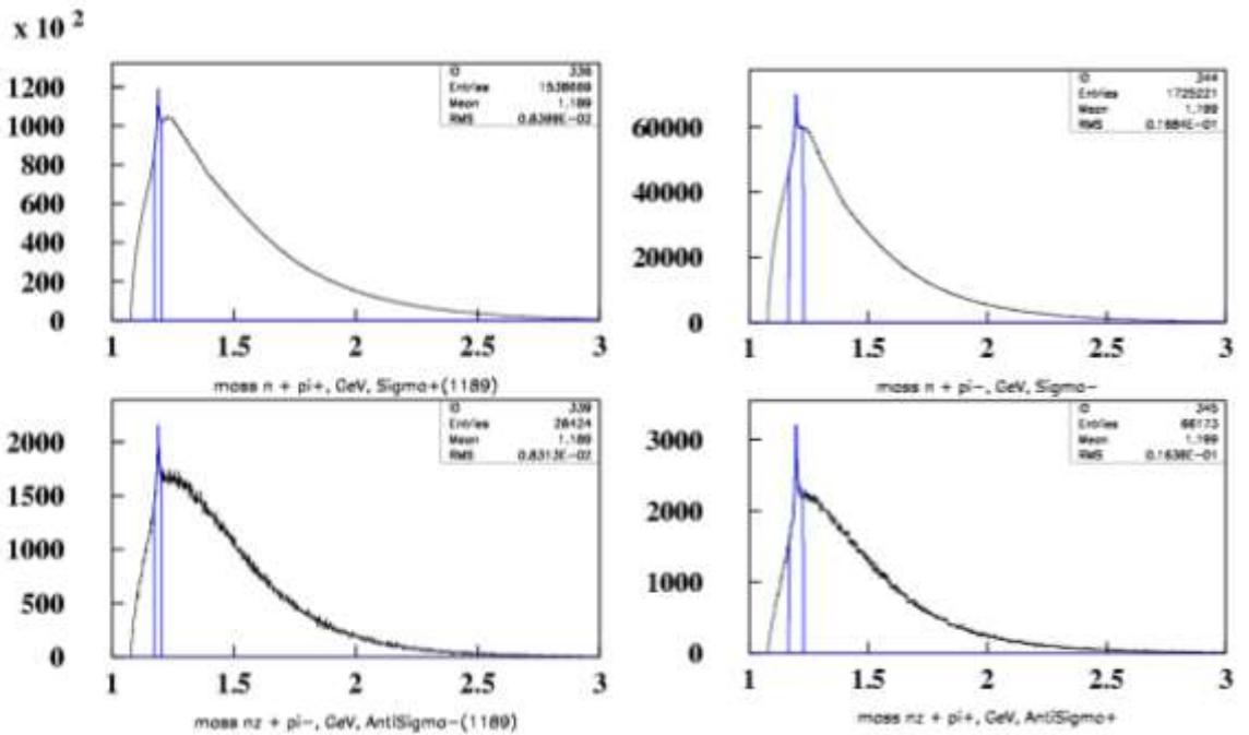
Рис. 6.3 Эффективная масса продуктов распада в процессе pp \rightarrow h + X : где h = \Sigma^+ \rightarrow n \pi^+ (a); h = \Sigma^- \rightarrow n \pi^- (b); h = \Sigma^- \rightarrow n \pi^- (c); h = \Sigma^+ \rightarrow n \pi^+ (d)
