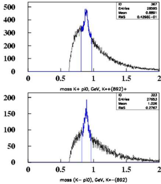
Рис. 6.2 Эффективная масса продуктов распада в процессах типа pp \rightarrow h + X : где h = K^{*+}(892) \rightarrow K^+ \pi^0 (вверху) и h = \tilde{K}^{*0}(892) \rightarrow K^- \pi^0 (внизу)
