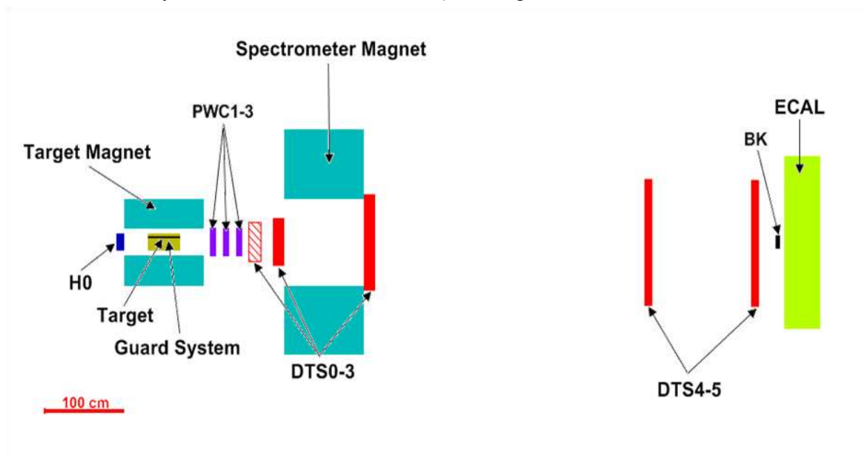
Рис. 3.2 Схема установки СПАСЧАРМ, детекторы показаны не в масштабе (детекторы DTS0-1 соответствуют детекторам DT1-2 при работе на канале 24)
