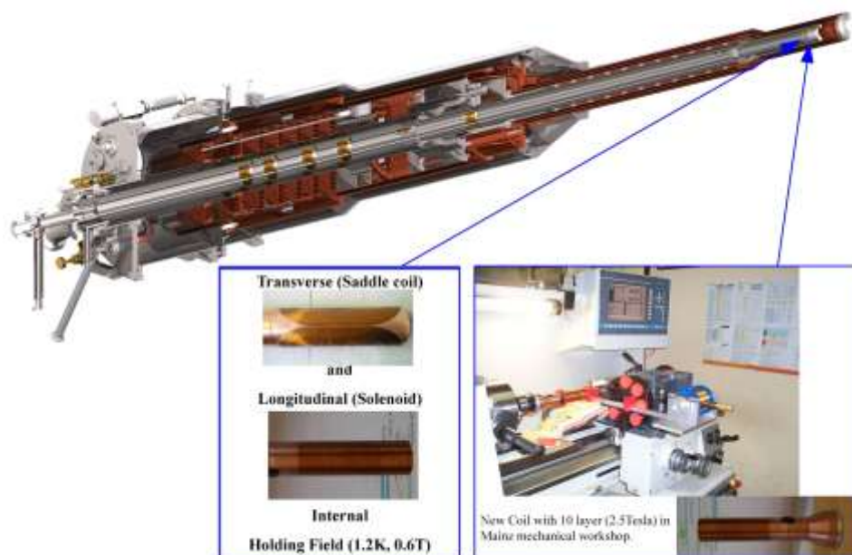
Рис. 3.12 Криостат поляризованной мишени с поляризирующей и удерживающей поляризацию сверхпроводящими катушками
