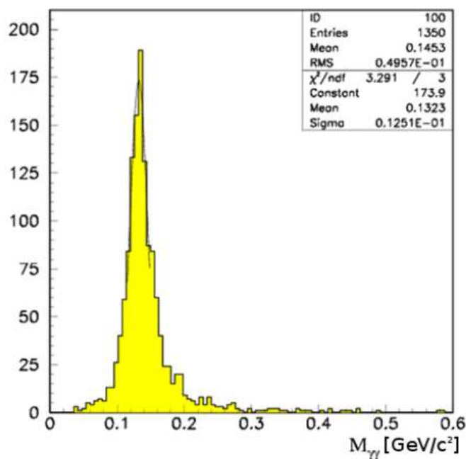
Рис. 3.34 Массовый спектр \pi^0 -мезонов с энергией от 1 до 2 ГэВ (детектор располагался на расстоянии 1,5 м от мишени)
