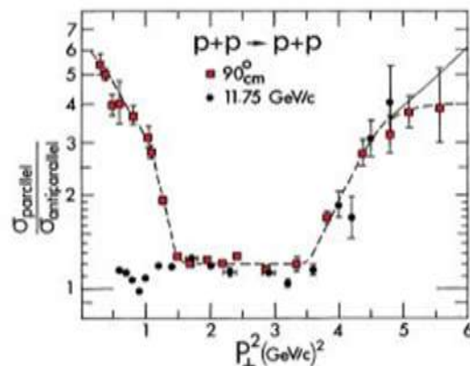
Рис. 5.2 Отношение упругих сечений \sigma_{\uparrow\uparrow}/\sigma_{\uparrow\downarrow} в зависимости от P_t^2 [129]
