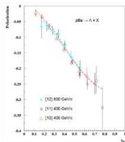
Рис. 5.9 P_N в реакции pBe \rightarrow \Lambda + X
