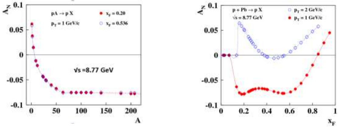
Рис. 1.10 Предсказания A_N в рамках модели хромомангнитной поляризации кварков
