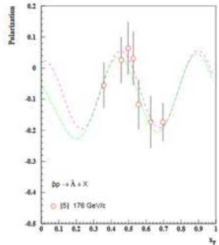
Рис. 5.14 P_N в реакции p\bar{p} \rightarrow \Lambda + X
