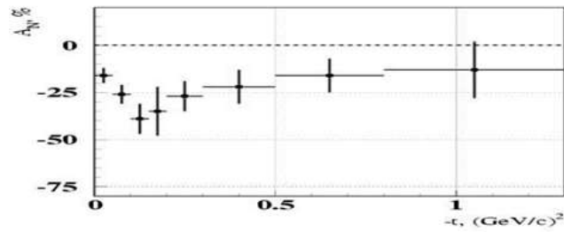
Рис. 5.4. Асимметрия в реакции \pi p \rightarrow f_2(1270) n при энергии 40 ГэВ [132], когда f_2(1270) -мезон регистрировался в режиме распада на два \pi^0 -мезона
