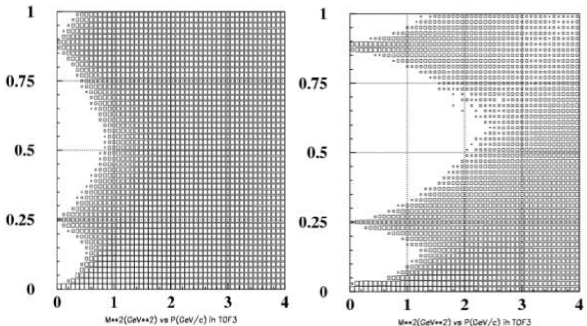
Рис. 3.38 Распределение по квадрату массы M^2 (ГэВ 2 /с 2 ) в зависимости от импульса частицы при расстоянии 7.6 м от мишени
