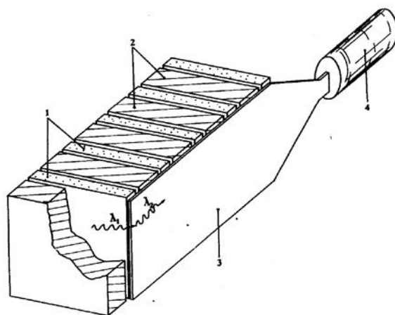
Рис. 3.35 Схематическое изображение модуля адронного калориметра: 1. сцинтилляционные пластины; 2 – свинцовый поглотитель; 3- спектроместитель (WLS); 4 – фотоумножитель
