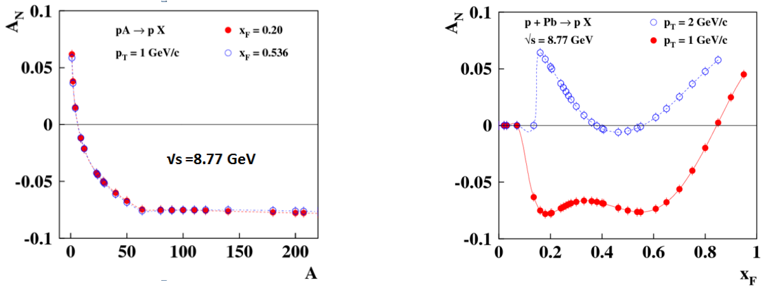
Рис. 1.10 Предсказания A_N в рамках модели хромагнитной поляризации кварков
