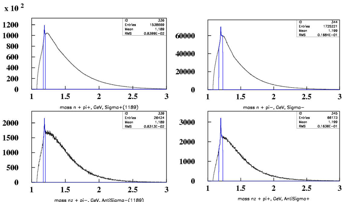
Рис. 6.3 Эффективная масса продуктов распада в процессе pp \rightarrow h + X : где h = \Sigma^+ \rightarrow n \pi^+ (a); h = \Sigma^- \rightarrow n \pi^- (b); h = \tilde{\Sigma}^- \rightarrow \tilde{n} \pi^- (c); h = \tilde{\Sigma}^+ \rightarrow \tilde{n} \pi^+ (d)
