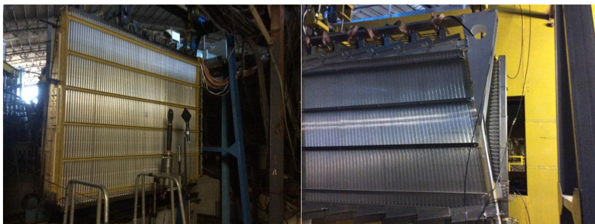
Рис. 3.24 Четвертая станция камер на рабочем месте с установленным перед ней триггерным счетчиком на взаимодействие, справа – третья станция, расположенная сразу после магнита.
