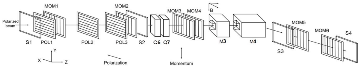
Рис. 2.11 Схема размещения детекторов мечения пучка. Импульс частицы измеряется в горизонтальной плоскости с помощью импульсных годоскопов MOM1-MOM6 и магнитов M3 + M4 . Поляризация частицы определяется путем измерения ее импульса и вертикальной y координаты поляризационными годоскопами POL1-POL3 . S1-S4 – сцинтилляционные счетчики полного потока. Промежуточный фокус по вертикали для центрального импульса находится в плоскости размещения годоскопа POL2 .
