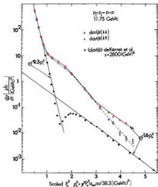
Рис. 6.1 Сечение протон-протонного упругого рассеяния в зависимости от скейлинговой переменной \rho^2_t = \beta^2 P^2_t \sigma_{tot}(s) / 38.3 [101].
