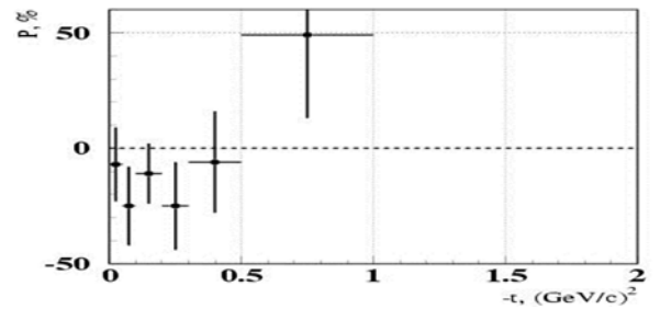
Рис. 1.15 Асимметрия в реакции \pi^+ p \rightarrow \eta'(958)n при энергии 40 ГэВ [105], когда \eta'(958) -мезон регистрировался в моде распада на два \gamma -кванта
