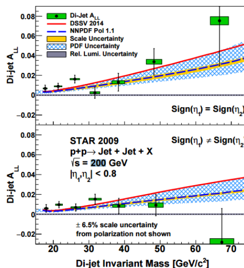
Рис. 1.2 Измерение двухспиновой асимметрии в эксперименте СТАР [14]
