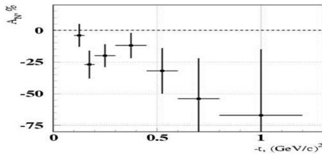
Рис. 1.14 Асимметрия в реакции \pi^+ p \rightarrow \omega(782)n при энергии 40 ГэВ [53], когда \omega(782) -мезон регистрировался в моде распада на \pi^0 и \gamma .
