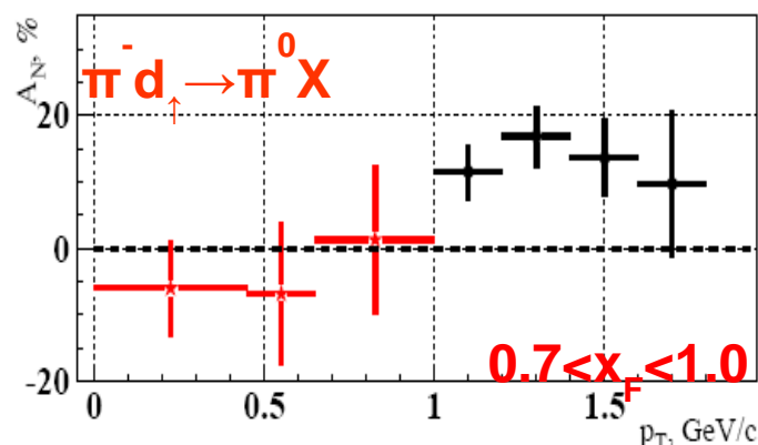
Рис. 1.13 Зависимость A_N(p_T) для реакции \pi^- d \rightarrow \pi^0 X при энергии пучка 40 ГэВ, в области фрагментации \pi^- пучка [48]. Значение x_F лежит в интервале 0.7 < x_F < 1.0 .
