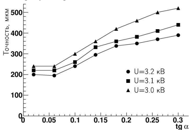
Рис. 3.29 Зависимость точности дрейфовых камер от тангенса угла наклона трека при различных напряжениях на потенциальных проволочках и фиксированном пороге дискриминации. Угол отсчитывается от нормали к плоскости камеры в плоскости, перпендикулярной направлению проволочек.
