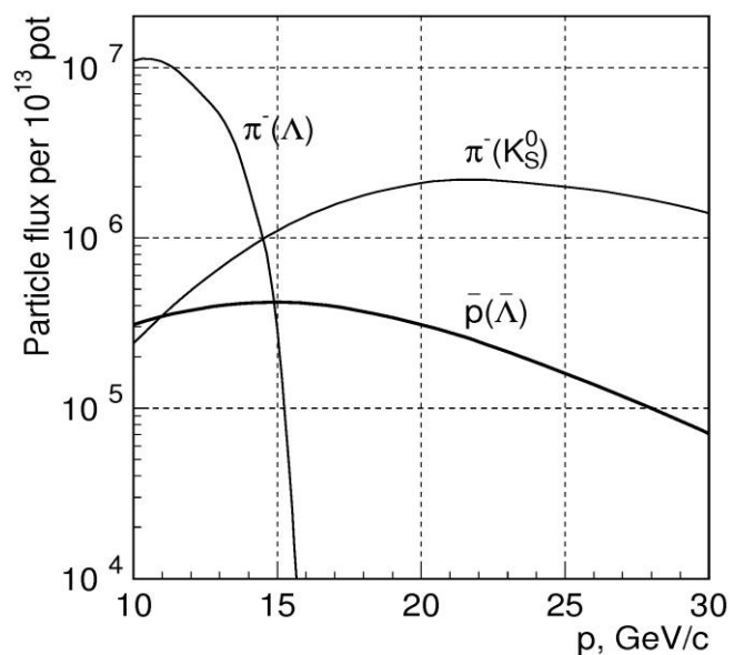
Рис. 2.10 Интенсивность пучка поляризованных антипротонов и фоновых \pi^- -мезонов в конце канала при максимальном \Delta p/p , рассчитанная на 10^{13} падающих на мишень протонов с энергией 60 ГэВ.
