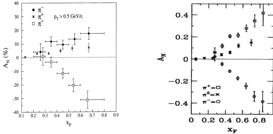
Рис. 1.7 Слева A_N в \bar{p}_1 -взаимодействии в рождении заряженных [30] и нейтральных [29] мезонов, справа – аналогичный результат для pp -взаимодействии [23, 29].
