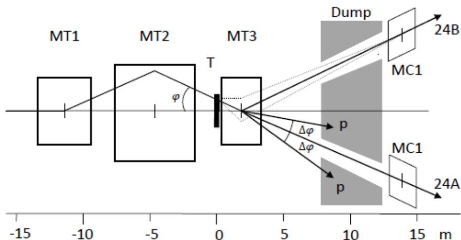
Рис. 2.3 Схема мишенной станции каналов 24А и 24В. Т – мишень канала, MT1÷MT3 – дипольные магниты, MC – магниты-корректоры, Dump – стальной поглотитель длиной 5 м. Приведенный на схеме мишенной станции вариант наведения протонного пучка на мишень соответствует отбору нейтральных вторичных частиц в канал 24А и положительно (отрицательно) заряженных частиц в канал 24В. Пунктирными линиями показаны траектории вторичных заряженных частиц, отбираемых с канал 24В с ненулевыми углами рождения в мишени.
