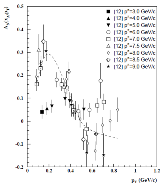
Рис. 5.6 A_N(p_T) для реакции p^+ p \rightarrow \pi^- + X
