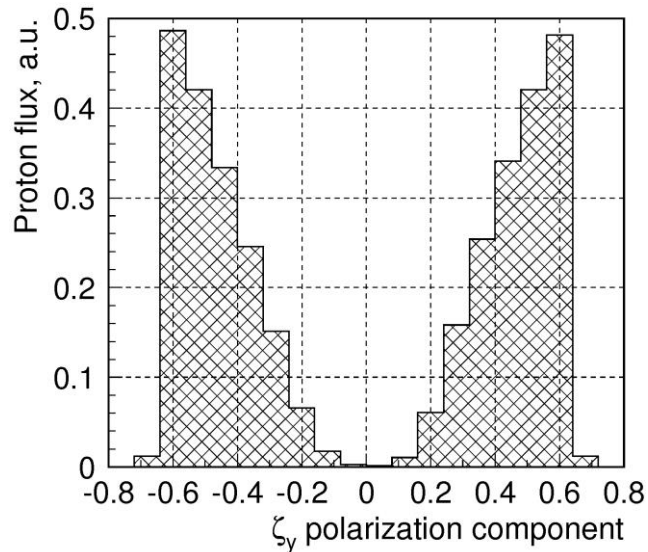
Рис. 2.9 Поляризация протонного пучка с импульсом 45 ГэВ/с на мишени установки для режимов корректора МС2, равных +0.12 Тл×м (слева) и -0.12 Тл×м (справа) при C4 = \pm 15 мм.
