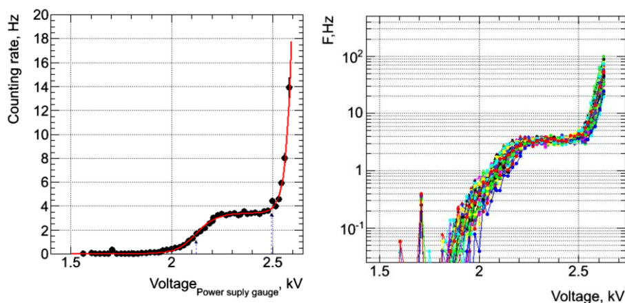
Рис. 3.23 Счетные характеристики всех трубок(правая панель) и усредненная характеристика всей камеры (левая панель)
