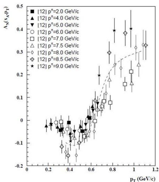
Рис. 5.5 A_N(p_T) для реакции p^+ p \rightarrow \pi^+ + X
