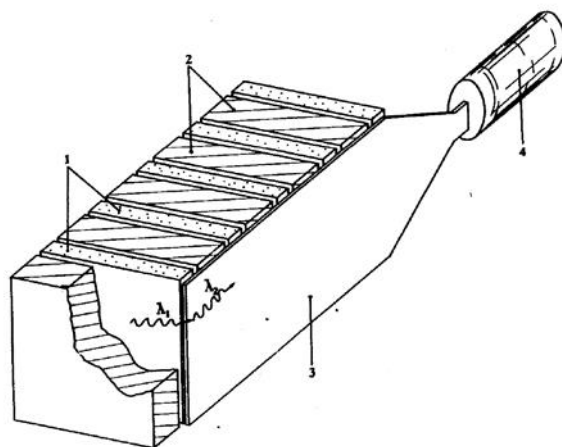
Рис. 3.35 Схематическое изображение модуля адронного калориметра: 1. сцинтилляционные пластины; 2 – свинцовый поглотитель; 3- спектростемитель (WLS); 4 – фотоумножитель
