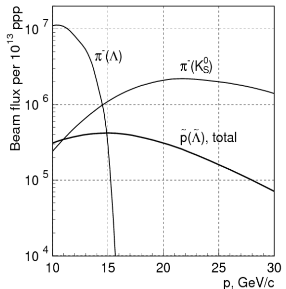
Рис. 2.10 Интенсивность пучка поляризованных антипротонов и фоновых \pi^- -мезонов в конце канала при максимальном \Delta p/p , рассчитанная на 10^{13} падающих на мишень протонов с энергией 60 ГэВ
