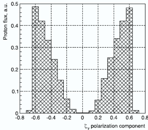
Рис. 2.9 Поляризация протонного пучка с импульсом 45 ГэВ/с на мишени установки для режимов корректора МС2, равных +0.12 Тл×м (слева) и -0.15 Тл×м (справа) при C4 = \pm 15 мм
