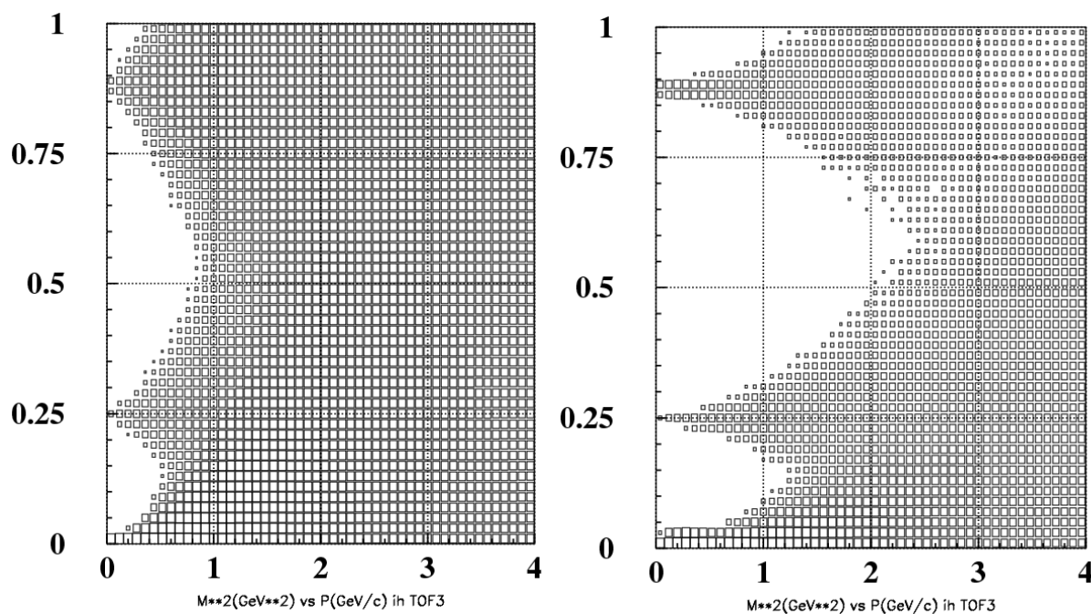
Рис. 3.38 Распределение по квадрату массы M^2 (ГэВ/с 2 ) в зависимости от импульса частицы при расстоянии 7.6 м от мишени
