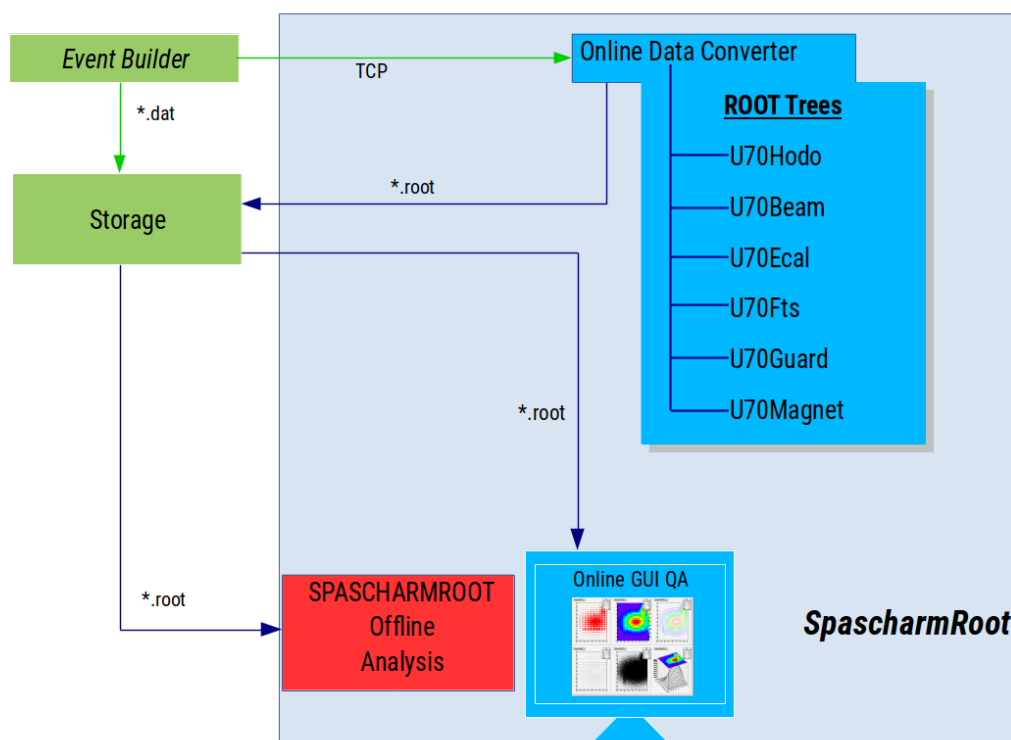
Рис. 3.52. Блок-схема программы обработки онлайн эксперимента СПАСЧАРМ.
