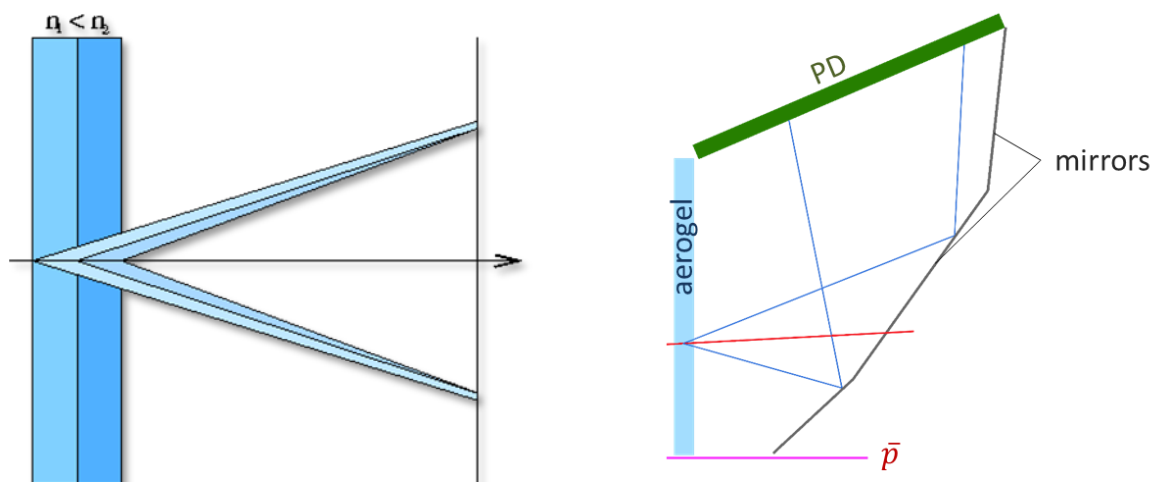
Рис. 3.36 Принцип фокусирования (слева) и принципиальная схема детектора на основе аэрогеля
