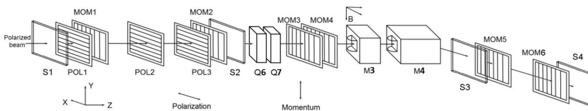
Рис. 2.12 Схема размещения детекторов мечения пучка. Импульс частицы измеряется в горизонтальной плоскости с помощью импульсных годоскопов MOM1-MOM6 и магнитов M3 + M4 . Поляризация частицы определяется путем измерения ее импульса и вертикальной y координаты поляризационными годоскопами POL1-POL3 . S1-S4 – сцинтилляционные счетчики полного потока. Промежуточный фокус по вертикали для центрального импульса находится в плоскости размещения годоскопа POL2 .
