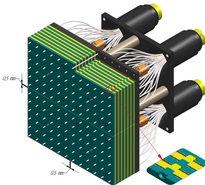
Рис. 3.31 Часть модуля калориметра в разрезе
