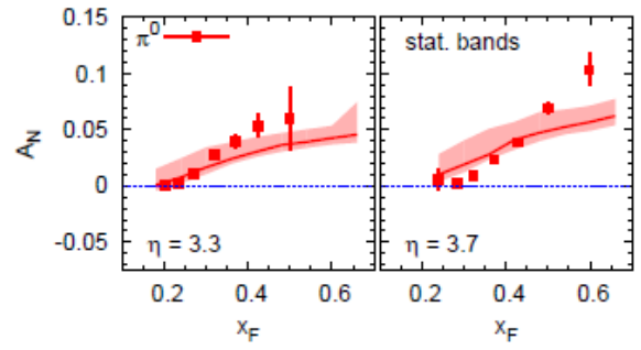
Рис. 5.16 Зависимость A_N(x_F) для p^+p^- \rightarrow \pi^0 X , из работы [166].
