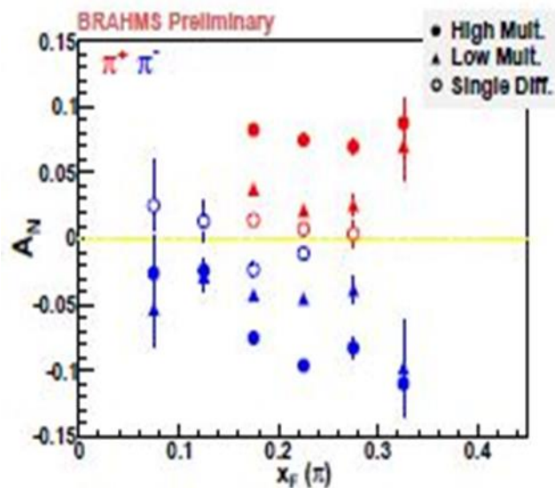
Рис. 5.8 Зависимость A_N(x_F) для реакции p \uparrow p \rightarrow \pi^\pm + X в эксперименте BRAHMS [30].
