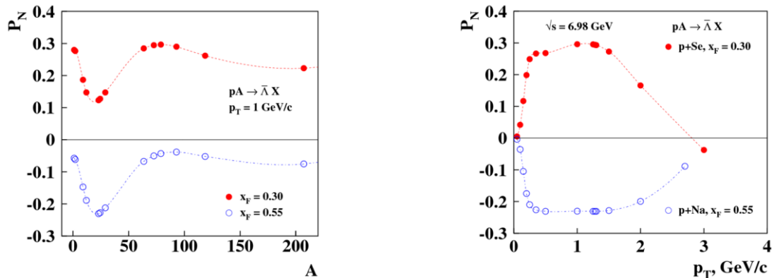
Рис. 1.12 Предсказания поляризации анти-лямбда гиперонов в pA -взаимодействии в рамках модели хромагнитной поляризации кварков
