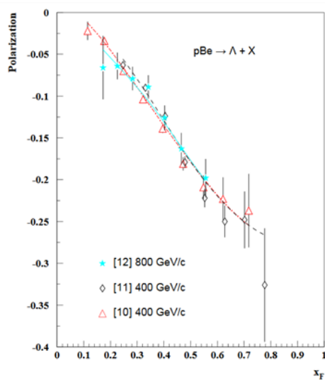
Рис. 5.9 P_N в реакции pBe \rightarrow \Lambda + X
