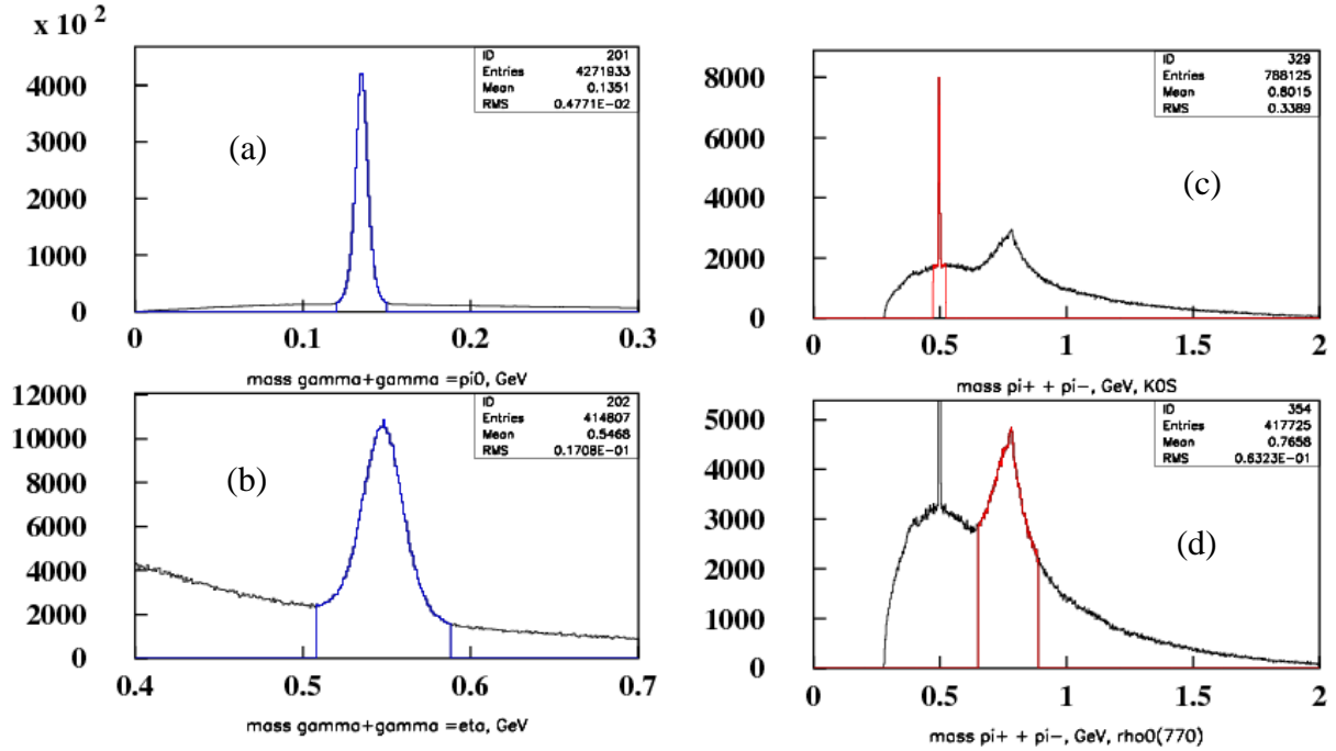
Рис. 6.4. Эффективная масса продуктов распада в процессе \pi^- p \rightarrow h + X , где h = \pi^0 \rightarrow \gamma\gamma (a); h = \eta \rightarrow \gamma\gamma (b); h = K_S^0 \rightarrow \pi^+ \pi^- (c); h = \rho^0(770) \rightarrow \pi^+ \pi^- (d).
