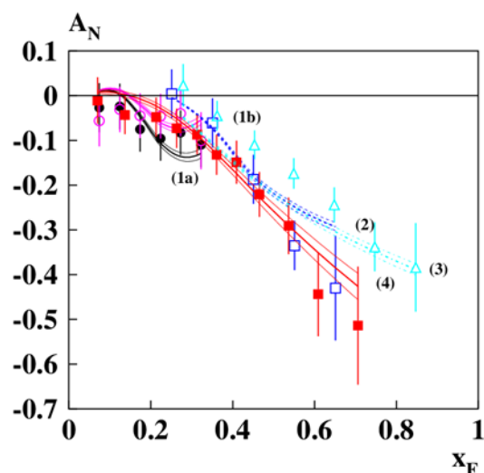
Рис. 5.29 A_N(x_F) для реакции p^\uparrow p(A) \rightarrow \pi^- + X
