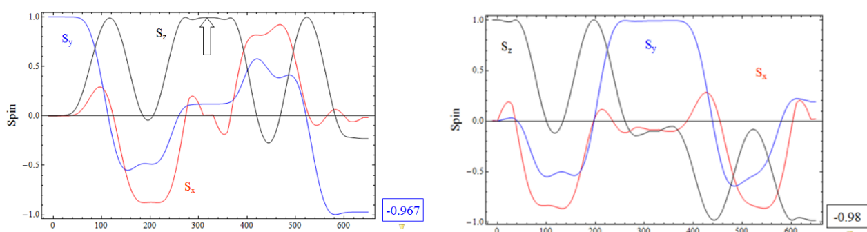
Рис. 2.28 Спиновые траектории для поперечной (слева) и продольной (справа) поляризаций
