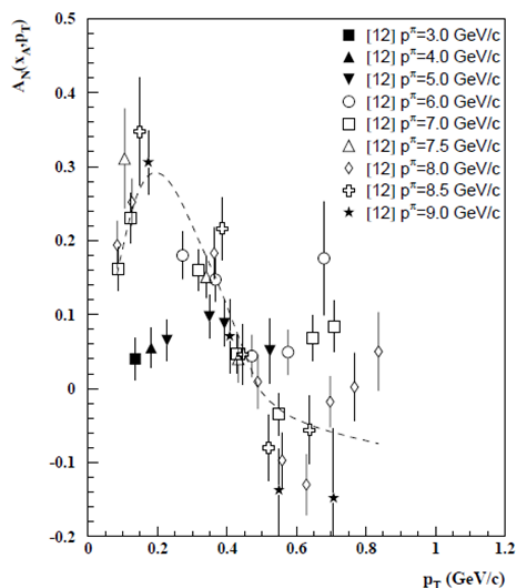
Рис. 5.6 A_N(p_T) для реакции p^\dagger p \rightarrow \pi^- + X
