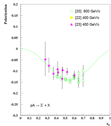
Рис. 5.10 P_N в реакции pA \rightarrow \Xi + X
