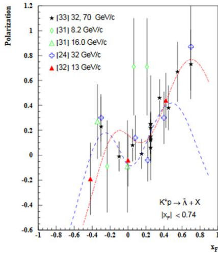
Рис. 5.13 P_N в реакции K^+p \rightarrow \Lambda + X
