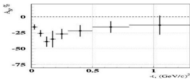
Рис. 5.4. Асимметрия в реакции \pi p \rightarrow f_2(1270) n при энергии 40 ГэВ [132], когда f_2(1270) -мезон регистрировался в моде распада на два \pi^0 -мезона
