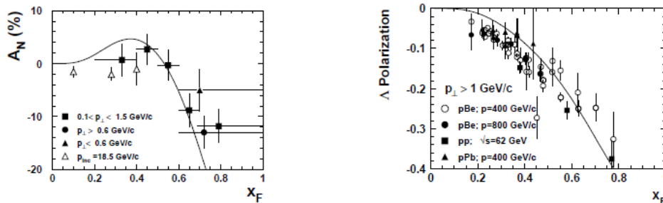
Рис. 5.20 A_N(x_F) (слева) для реакции p^\uparrow p \rightarrow \Lambda X и P_N(x_F) для pp(A) \rightarrow \Lambda X
