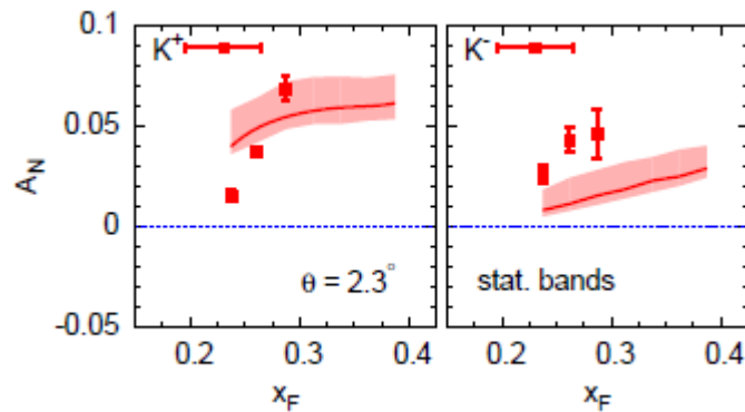
Рис. 5.17 Зависимость A_N(x_F) для K^\pm , из работы [165]
