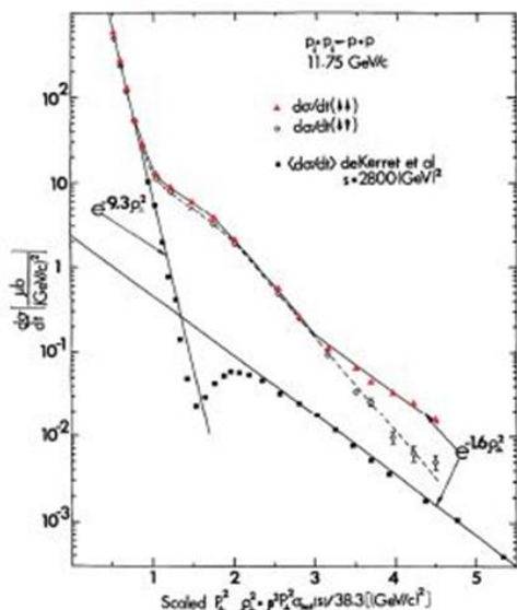
Рис. 5.1 Сечение протон-протонного упругого рассеяния в зависимости от скейлинговой переменной \rho_t^2 = \beta^2 P_t^2 \sigma_{tot}(s) / 38.3 [128].
