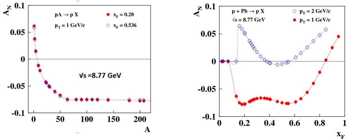
Рис. 1.10 Предсказания A_N в рамках модели хромагнитной поляризации кварков
