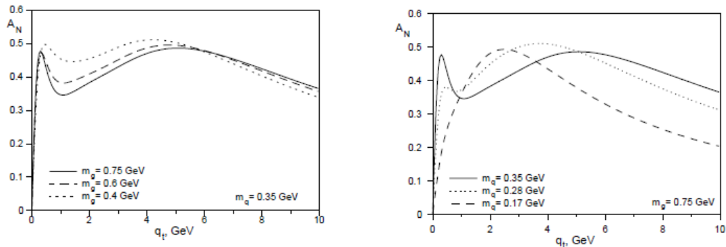
Рис. 5.21 A_N(q_t) для рассеяния кварков, при разных параметрах m_g инфракрасного обрезания (слева) и разных динамических массах кварка (справа) из модели [176]
