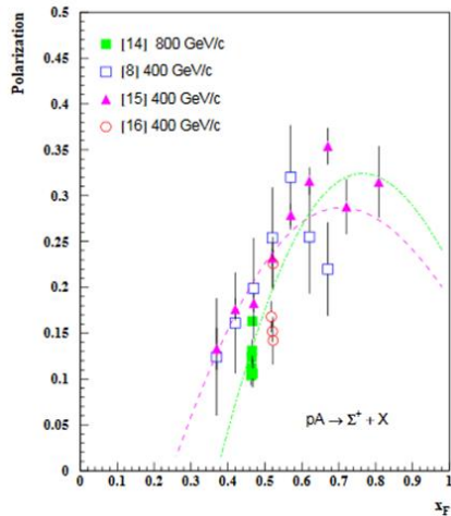
Рис. 5.11 P_N в реакции pA \rightarrow \Sigma^+ + X
