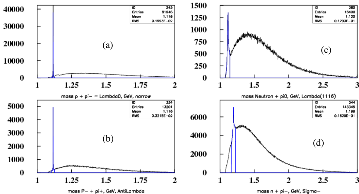
Рис. 6.5 Эффективная масса продуктов распада в процессе K^- p \rightarrow h + X : h = \Lambda \rightarrow p \pi^- (a); h = \tilde{\Lambda} \rightarrow \tilde{p} \pi^+ (b); h = \Lambda \rightarrow n \pi^0 (c); h = \Sigma^- \rightarrow n \pi^- (d).
