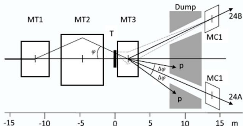
Рис. 2.3 Схема мишенной станции каналов 24А и 24В. Т – мишень канала, МТ1÷МТ3 – дипольные магниты, МС – магниты-корректоры, Dump – стальной поглотитель длиной 5 м. Приведенный на схеме мишенной станции вариант наведения протонного пучка на мишень соответствует отбору нейтральных вторичных частиц в канал 24А и положительно (отрицательно) заряженных частиц в канал 24В. Пунктирными линиями показаны траектории вторичных заряженных частиц, отбираемых с канал 24В с ненулевыми углами рождения в мишени.
