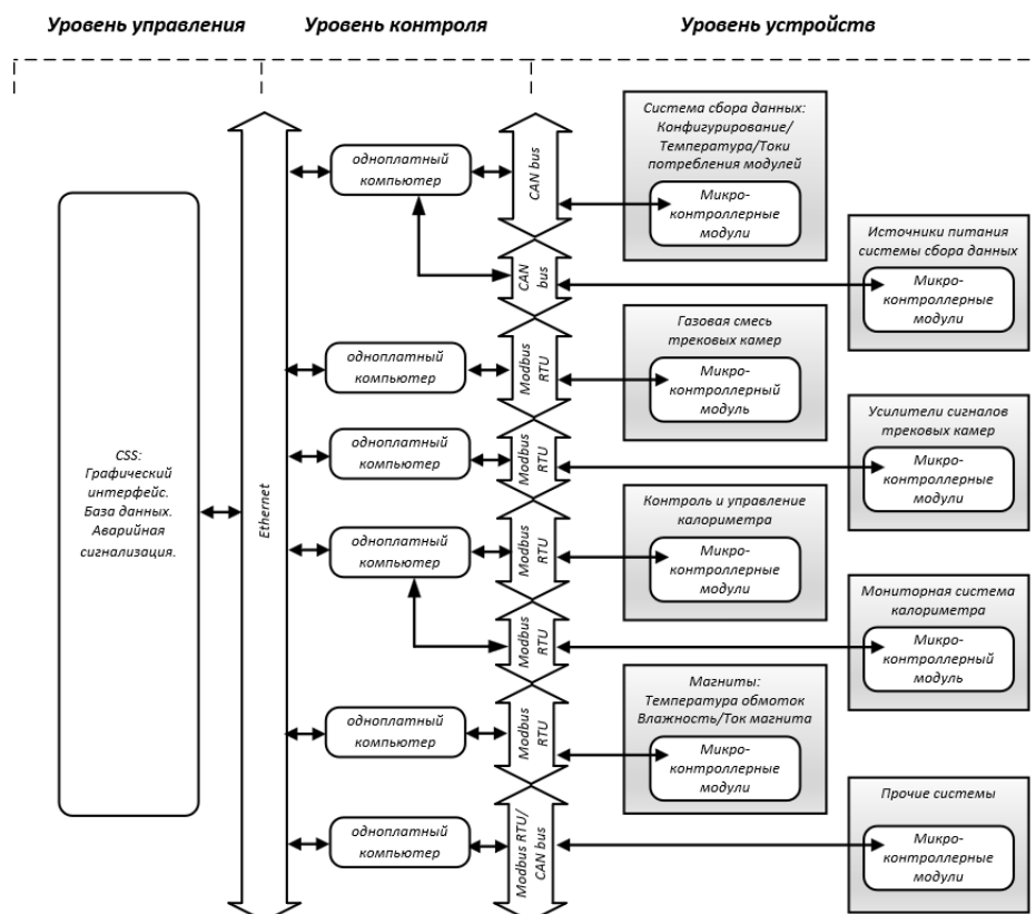
Рис. 3.42 Архитектура системы управления экспериментальной установки СПАСЧАРМ: Control System Studio.
