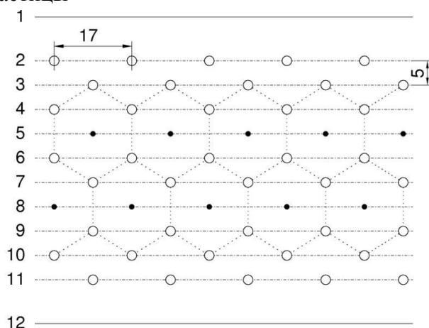
Рис. 3.27 Часть периодической структуры проволочных дрейфовых камер ЭПЕКУР (не в масштабе): 2,3,4,6,7,9,10,11 – плоскости потенциальных проволочек, 5,8 – плоскости сигнальных проволочек, 1,12 – майларовые окна, ограничивающие газовый объем
