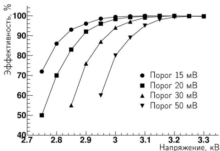
Рис. 3.28. Зависимость эффективности дрейфовой камеры от питающего напряжения при различных порогах дискриминации
