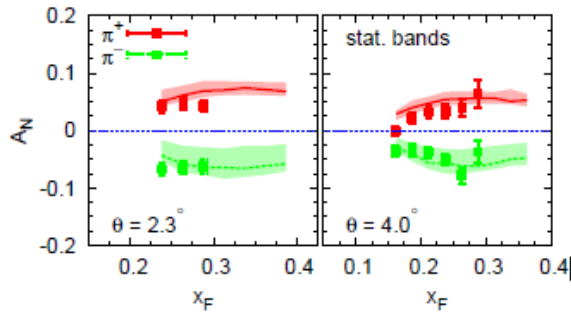
Рис. 5.15 Зависимость A_N(x_F) для p^+p^- \rightarrow \pi^\pm X , из работы [166].
