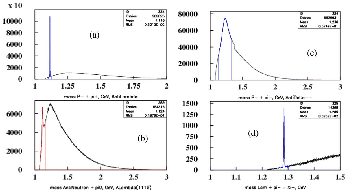
Рис. 6.1 Эффективная масса продуктов распада в процессе \tilde{p} p \rightarrow h + X : h = \tilde{\Lambda} \rightarrow \tilde{p} \pi^+ (a); h = \tilde{\Lambda} \rightarrow \tilde{n} \pi^0 (b); h = \tilde{\Delta}^{--} \rightarrow \tilde{p} \pi^- (c); h = \Xi^- \rightarrow \Lambda \pi^- (d).
