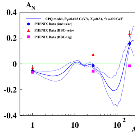
Рис. 1.9 Зависимость A_N(A) для реакции p^+A \rightarrow n + X в эксперименте PHENIX [29].
