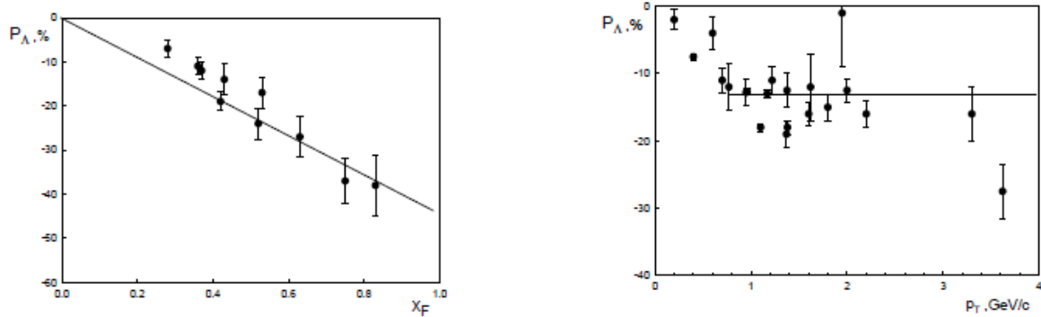
Рис. 5.23 P_N(x_F) (слева) и P_N(p_T) (справа) для реакции pp(A) \rightarrow \Lambda^1 X , сплошные линии – предсказания по модели фильтрации спина [181]
