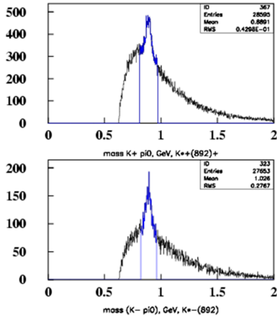
Рис. 6.2 Эффективная масса продуктов распада в процессах pp \rightarrow h + X : где h = K^{*+}(892) \rightarrow K^+ \pi^0 (вверху) и h = \tilde{K}^{*-}(892) \rightarrow K^- \pi^0 (внизу)
