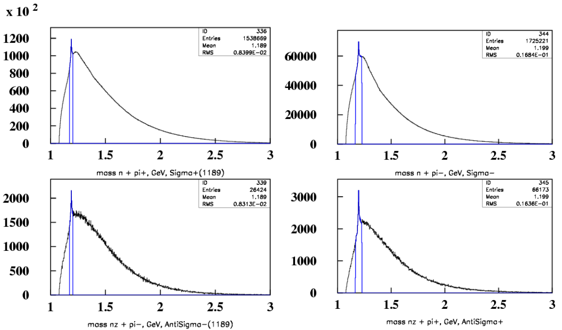
Рис. 6.3 Эффективная масса продуктов распада в процессе pp \rightarrow h + X : где h = \Sigma^+ \rightarrow n \pi^+ (a); h = \tilde{\Sigma}^- \rightarrow \tilde{n} \pi^- (b); h = \Sigma^- \rightarrow n \pi^- (c); h = \Sigma^+ \rightarrow \tilde{n} \pi^+ (d).
