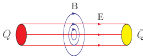
Рис. 5.25 Схематическая картина трубки цветового потока между кварком и антикварком. Продольные линии показывают направление хромозлектрического поля E , а круговые направление хромомангнитного поля B .
