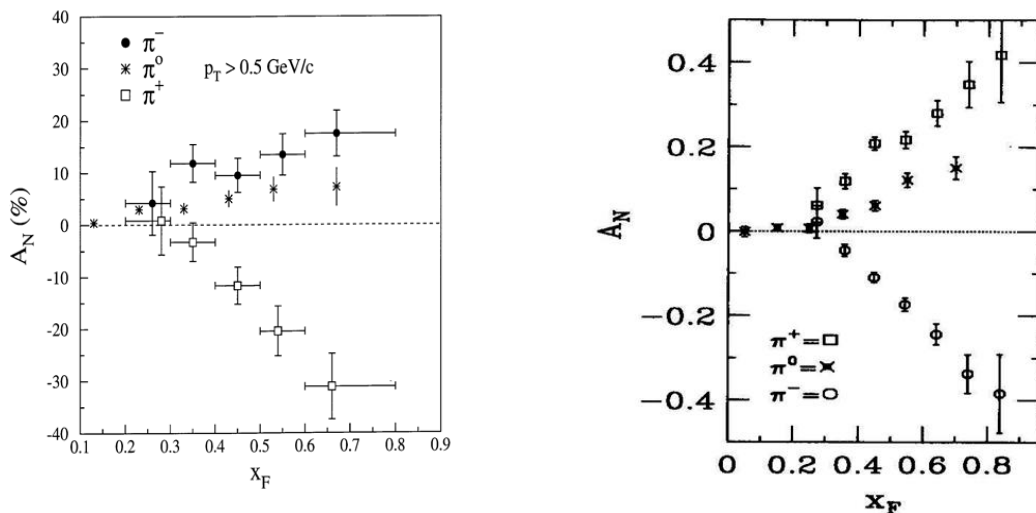
Рис. 1.7 Слева A_N в \bar{p}p -взаимодействии в рождении заряженных [30] и нейтральных [29] мезонов, справа – аналогичный результат для pp -взаимодействии [23, 29].
