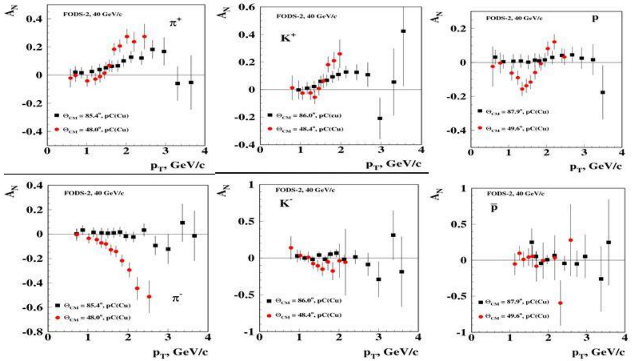
Рис. 5.7 Зависимость A_N(p_T) для процессов инклюзивного образования \pi^\pm , \pi^\pm , p и \bar{p} в p^\uparrow A соударениях, при двух углах рождения адронов и импульсе 40 ГэВ/с.
