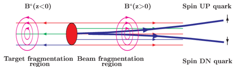
Рис. 5.27 Механизм хромомагнитной поляризации кварков (микроскопический аппарат Штерна-Герлаха). Кварк-пробник отклоняется влево или вправо в неоднородном поле B^a .
