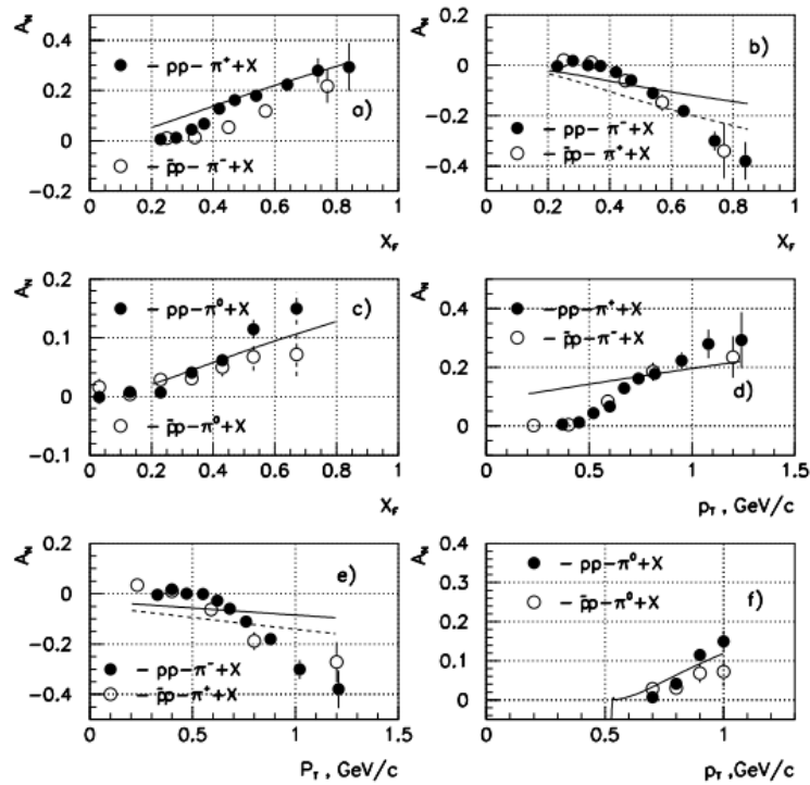
Рис. 5.26 Сравнение данных E704 для p^\uparrow p (черные кружочки) [23] и p^\uparrow \bar{p} (открытые кружочки) [190], из работы [188].
