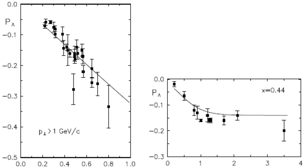
Рис. 5.24 P_N(x_F) для pp \rightarrow \Lambda^+ X (слева) и P_N(p_T) для pp(A) \rightarrow \Lambda^+ X (справа) из работы [183]
