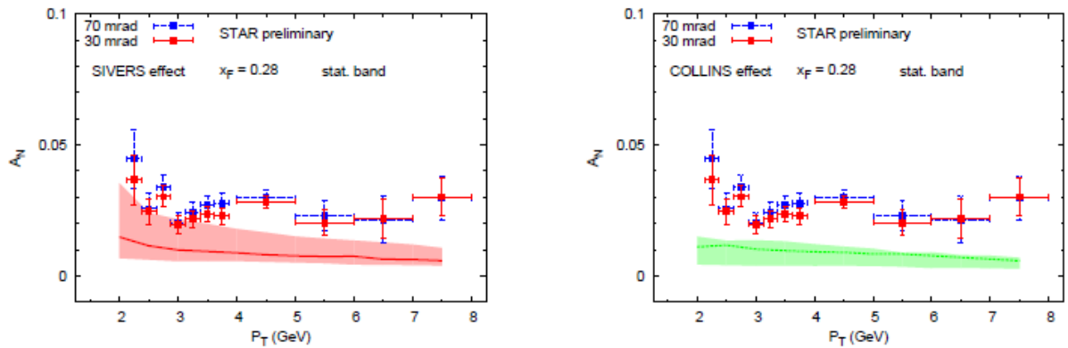
Рис. 5.18 Зависимость A_N(p_T) для реакции p^+p^- \rightarrow \pi^0 X , из работы [166] и предсказания в рамках моделей Сиверса (слева) и Коллинза (справа)
