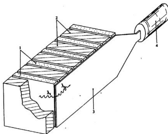
Рис. 3.35 Схематическое изображение модуля адронного калориметра: 1 - сцинтилляционные пластины; 2 - свинцовый поглотитель; 3 - спектроместитель (WLS); 4 - фотоумножитель
