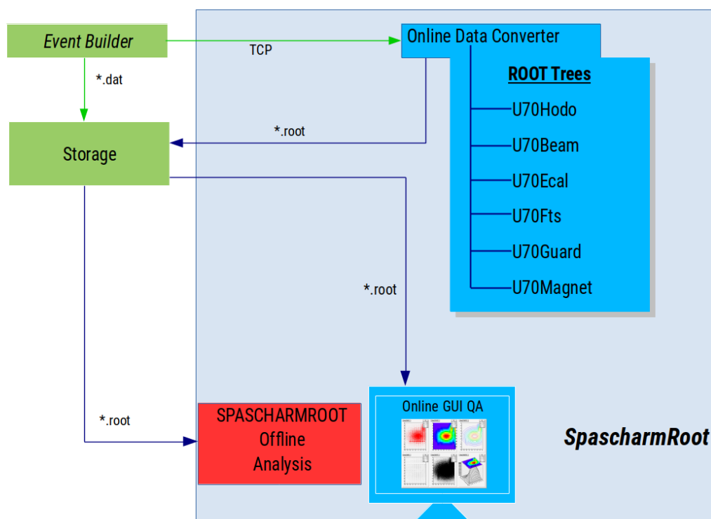
Рис. 3.52. Блок-схема программы обработки онлайн эксперимента СПАСЧАРМ.
