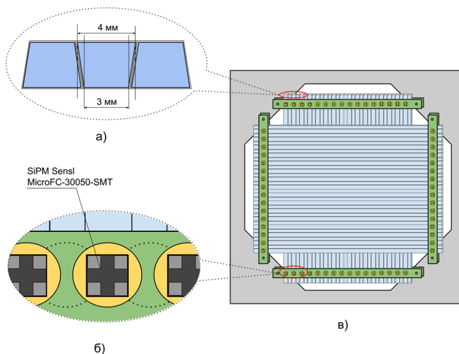
Рис. 2.14. Вариант конструкции однослойного годоскопа системы мечения. а) Вид с торца на сегменты сцинтиллятора. Трапецевидная форма позволяет улучшить эффективность регистрации на границе сегментов. б) Крепление фотодетекторов (кремниевых фотоумножителей) к сегментам сцинтиллятора. в) Общий вид двухкоординатного годоскопа
