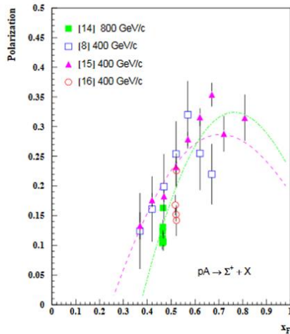
Рис. 5.11 P_N в реакции pA \rightarrow \Sigma^+ + X
