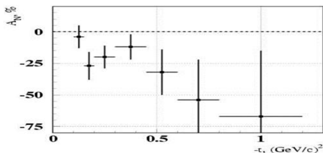
Рис. 1.14 Асимметрия в реакции \bar{\pi}p \rightarrow \omega(782)n при энергии 40 ГэВ [55], когда \omega(782) -мезон регистрировался в моде распада на \pi^0 и \gamma .
