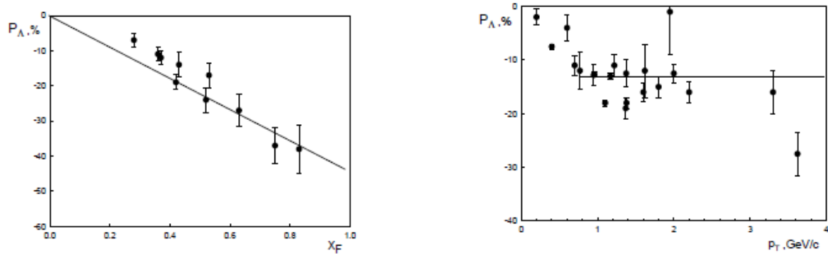
Рис. 5.23 P_N(x_F) (слева) и P_N(p_T) (справа) для реакции pp(A) \rightarrow \Lambda^{\uparrow}X , сплошные линии – предсказания по модели фильтрации спина [181]
