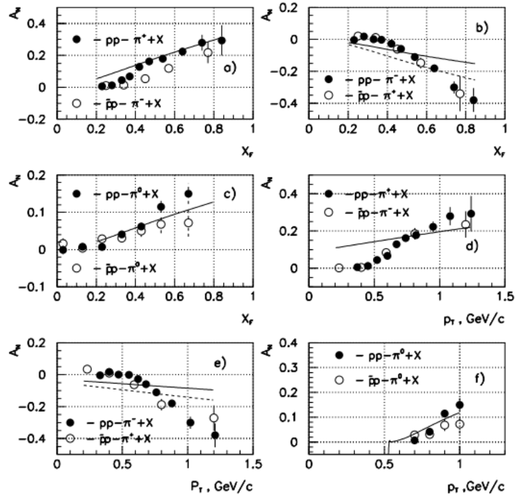
Рис. 5.26 Сравнение данных E704 для p^{\uparrow}p (черные кружочки) [23] и p^{\downarrow}p (открытые кружочки) [190], из работы [188].
