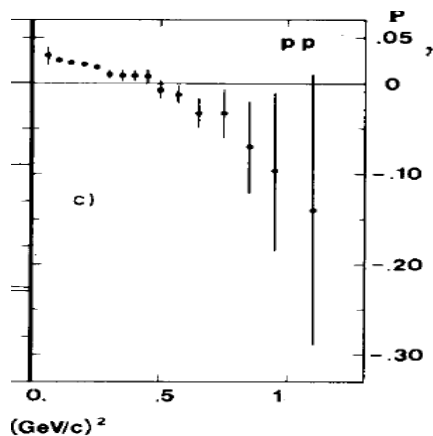
Рис. 2.20 Поляризация в упругом pp-рассеянии при импульсе 45 ГэВ/с
