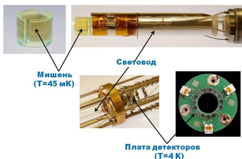
Рис. 3.13 Основные внутренние узлы, созданной совместными усилиями (Майнц-Бонн-Бохум-ОИЯИ) мишени-сцинтиллятора
