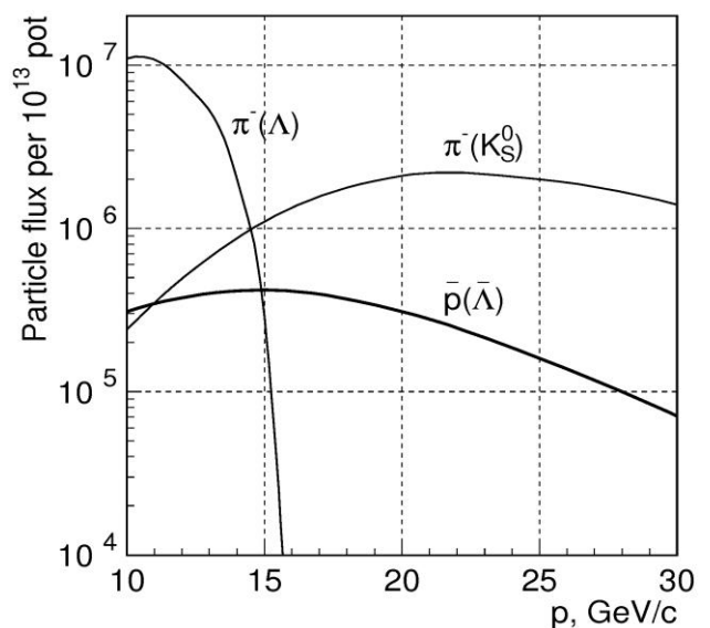
Рис. 2.10 Интенсивность пучка поляризованных антипротонов и фоновых \pi^- -мезонов в конце канала при максимальном \Delta p/p , рассчитанная на 10^{13} падающих на мишень протонов с энергией 60 ГэВ.
