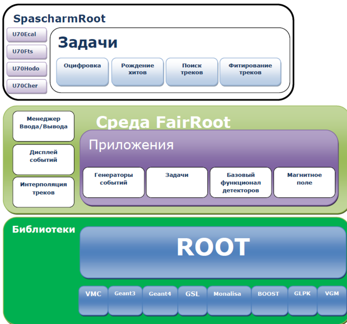
Рис. 3.48. Схематическая структура программной среды эксперимента СПАСЧАРМ: внизу – библиотеки сторонних разработчиков, в центре – среда FairRoot, сверху – конкретная реализация SpascharmRoot
