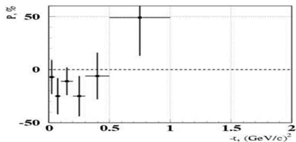
Рис. 1.15 Асимметрия в реакции \bar{\pi}p \rightarrow \eta'(958)n при энергии 40 ГэВ [132], когда \eta'(958) -мезон регистрировался в моде распада на два \gamma -кванта
