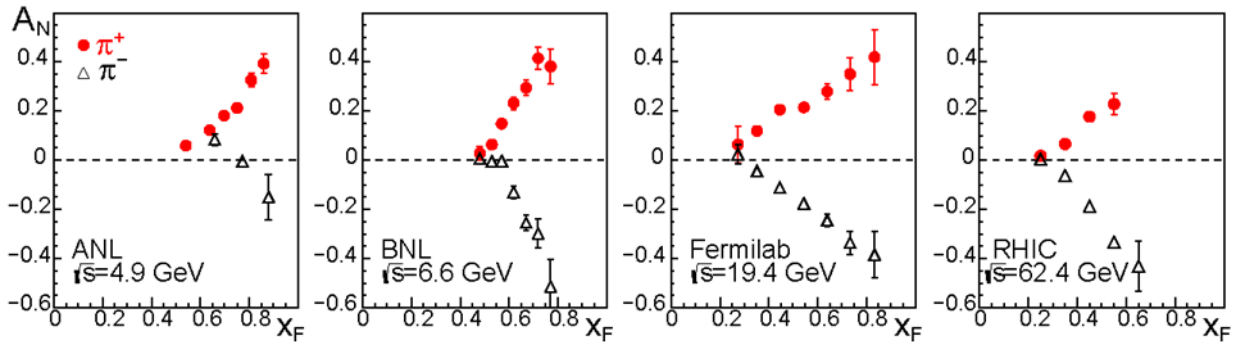
Рис. 1.6 A_N для реакций p^\uparrow p \rightarrow \pi^\pm + X . Данные ZGS [21], AGS [22], FNAL [23], RHIC [24]. Компильация экспериментальных данных из публикации [28]
