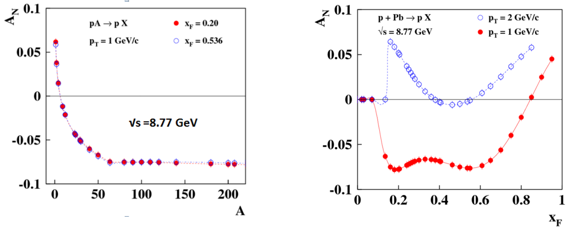
Рис. 1.10 Предсказания A_N в рамках модели хромоманнитной поляризации кварков
