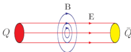
Рис. 5.25 Схематическая картина трубки цветового потока между кварком и антикварком. Продольные линии показывают направление хромоэлектрического поля E , а круговые направление хромагнитного поля B .
