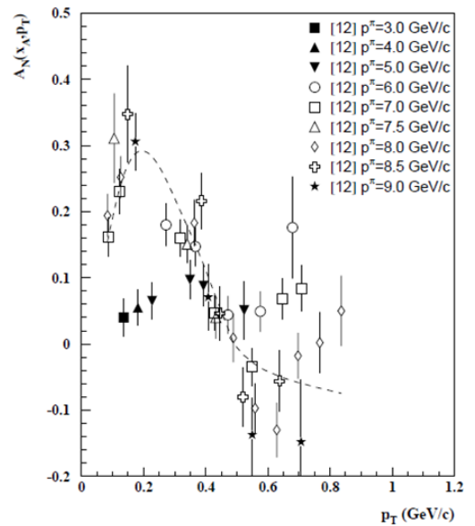
Рис. 5.6 A_N(p_T) для реакции p^+ p \rightarrow \pi^- + X
