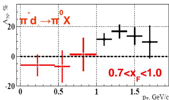
Рис. 1.13 Зависимость A_N(p_T) для реакции \pi^- d \rightarrow \pi^0 X при энергии пучка 40 ГэВ, в области фрагментации \pi^- пучка [50]. Значение x_F лежит в интервале 0.7 < x_F < 1.0 .
