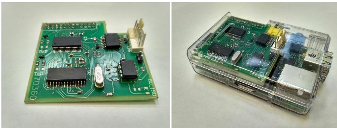
Рис. 3.43 Адаптер шин для Modbus RTU и CAN
