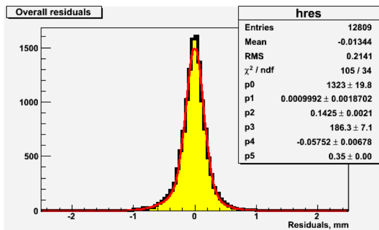
Рис. 3.26 Разность между восстановленной координатой трека и координатой в данной подплоскости
