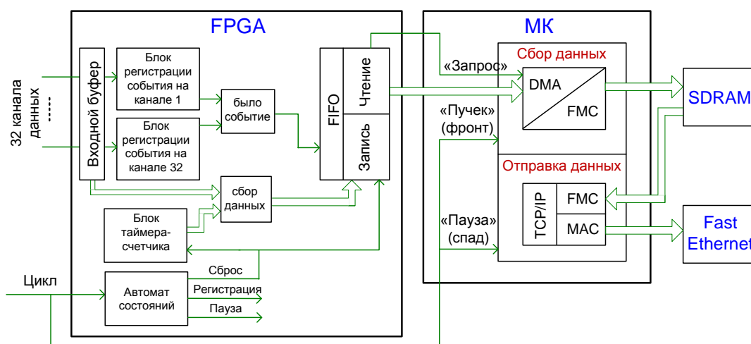
Рис. 2.18 Общий алгоритм взаимодействия двух плат прототипа
