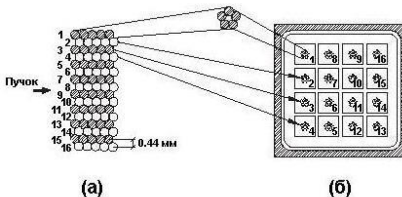
Рис. 3.5 Схематическое изображение части сцинтиляционной волоконной кассеты (а) и расположение волокон на фотокатоде 16-анодного ФЭУ Hamamatsu R7600-200-M16 (б).
