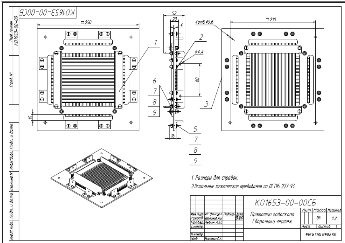
Рис. 2.15 Рама двухкоординатного годоскопа на 32 канала по каждой координате
