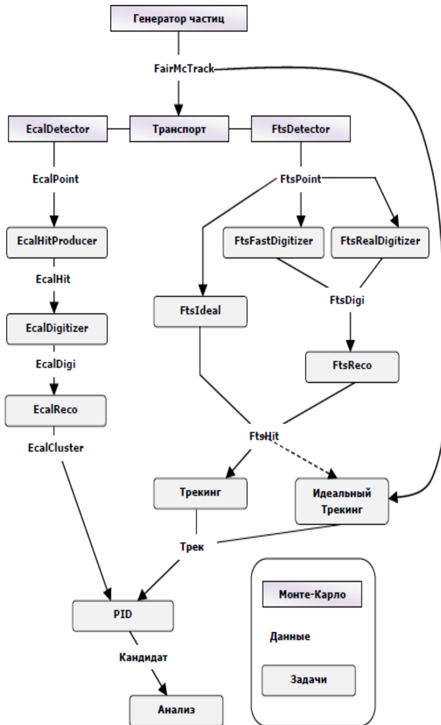
Рис. 3.51. Последовательность выполнения «задач» в среде SpascharmRoot на примере детектора идентифицирующего частицы (калориметр или ECAL) и трекового детектора (система станций дрейфовых трубок или FTS) при моделировании. Модульная архитектура программной среды позволяет подключать компоненты, необходимые для конкретного случая.
