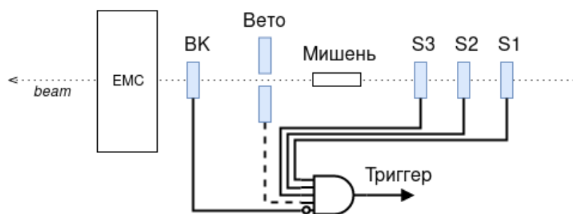
Рис. 3.40 Схема триггера установки
