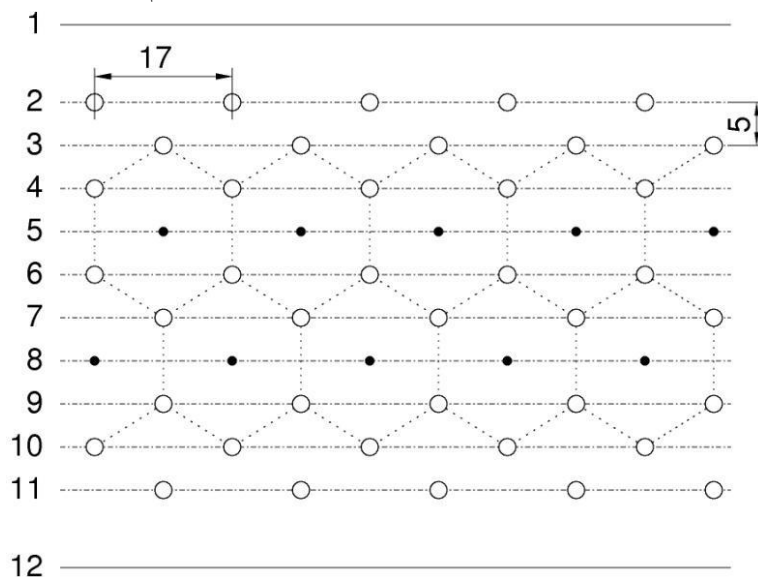
Рис. 3.27 Часть периодической структуры проволоочных дрейфовых камер ЭПЕКУР (не в масштабе): 2,3,4,6,7,9,10,11 – плоскости потенциальных проволоочек, 5,8 – плоскости сигнальных проволоочек, 1,12 – майларовые окна, ограничивающие газовый объем
