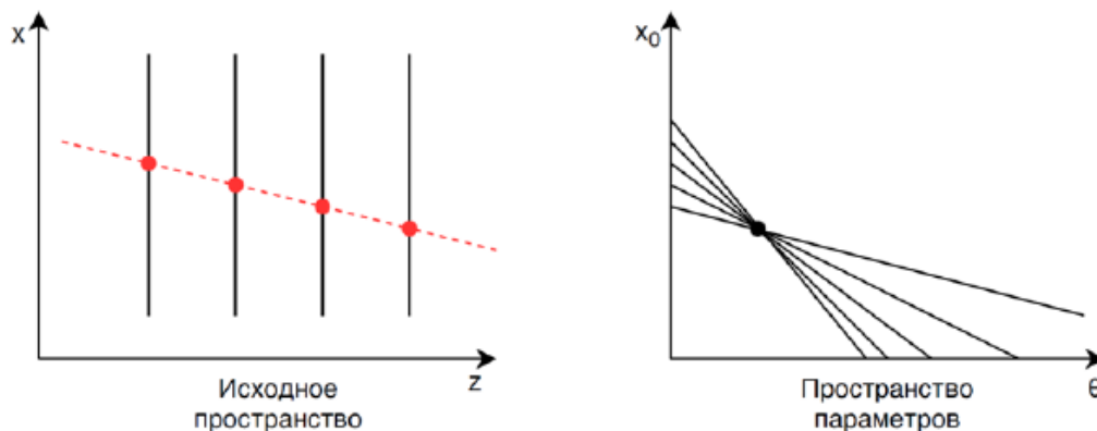
Рис. 3.54 Иллюстрация основного принципа преобразования Хафа для одного трека
