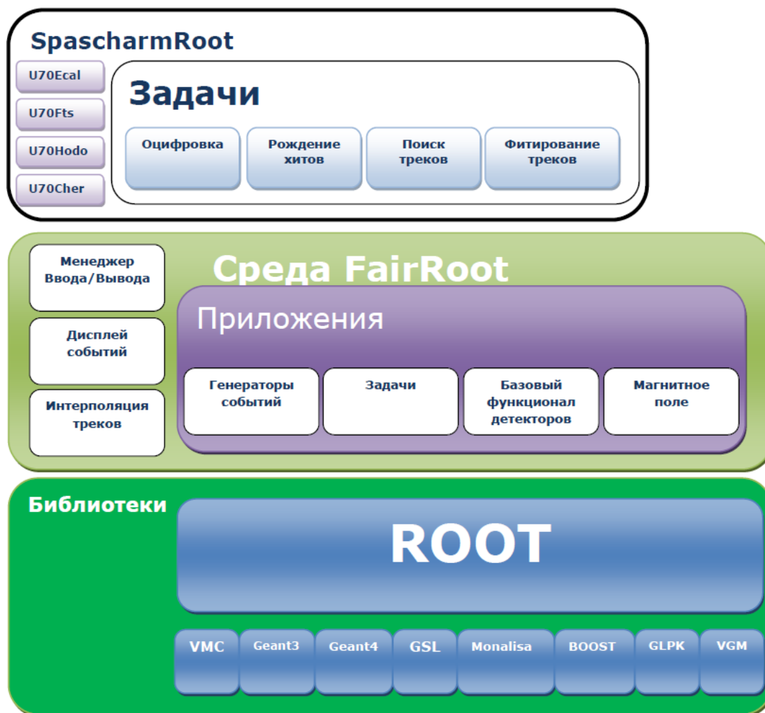
Рис. 3.48. Схематическая структура программной среды эксперименте СПАСЧАРМ: внизу – библиотеки сторонних разработчиков, в центре – среда FairRoot, сверху – конкретная реализация SpascharmRoot
