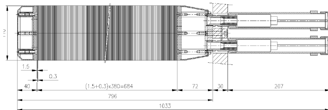
Рис. 3.30 Чертеж супермодуля калориметра
