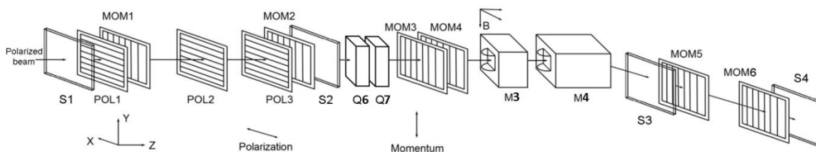
Рис. 2.12 Схема размещения детекторов мечения пучка. Импульс частицы измеряется в горизонтальной плоскости с помощью импульсных годоскопов MOM1-MOM6 и магнитов M3 + M4 . Поляризация частицы определяется путем измерения ее импульса и вертикальной y координаты поляризационными годоскопами POL1-POL3 . S1-S4 – сцинтилляционные счетчики полного потока. Промежуточный фокус по вертикали для центрального импульса находится в плоскости размещения годоскопа POL2 .
