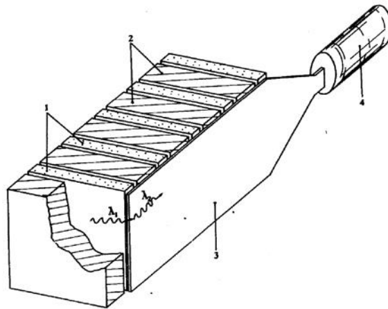
Рис. 3.35 Схематическое изображение модуля адронного калориметра: 1. сцинтилляционные пластины; 2 – свинцовый поглотитель; 3- спектрсмещитель (WLS); 4 – фотоумножитель
