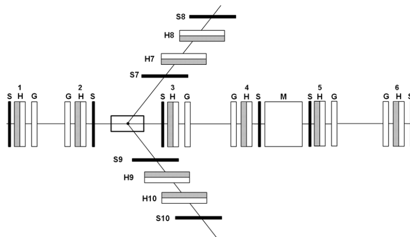
Рис. 2.19 Схема комбинированного поляриметра. G - GEM детекторы; H – сцинтилляционные годоскопы; S – сцинтилляционные счётчики
