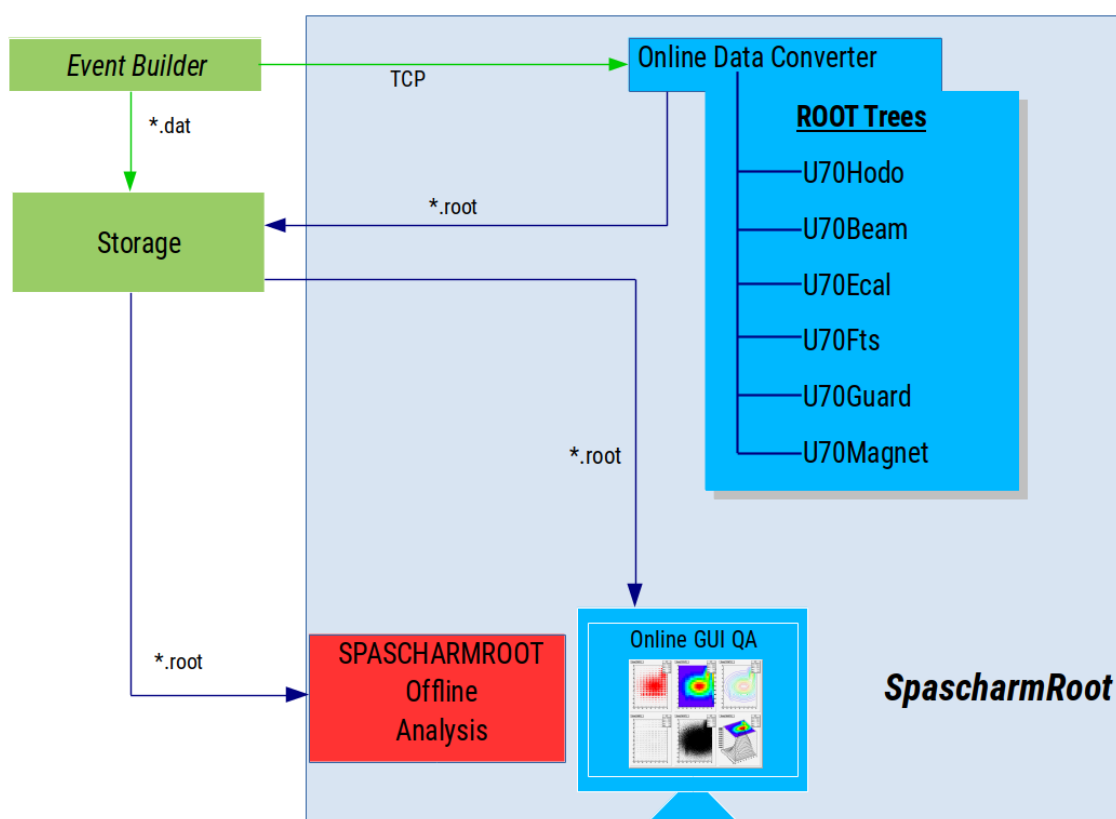
Рис. 3.52. Блок-схема программы обработки онлайн эксперимента СПАСЧАРМ.
