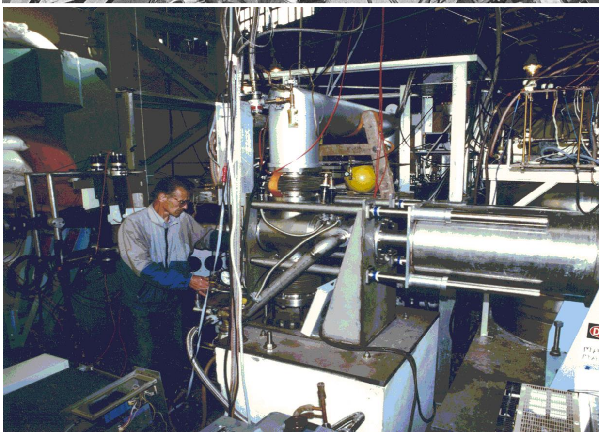
Рис. 3.11 Фотографии комплекса продольной поляризованной мишени сверху и сбоку
