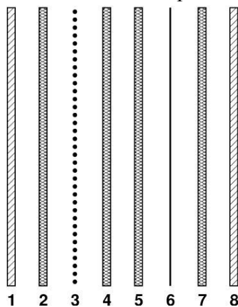
Рис. 3.3 Устройство двухкоординатных пропорциональных камер с шагом 1 мм (не в масштабе): 3,6 – плоскости сигнальных проволочек, 2,4,5,7 – высоковольтные электроды, 1,8 – майларовые окна, ограничивающие газовый объем
