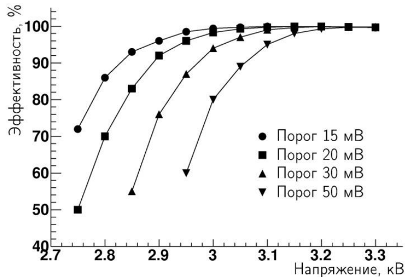
Рис. 3.28. Зависимость эффективности дрейфовой камеры от питающего напряжения при различных порогах дискриминации
