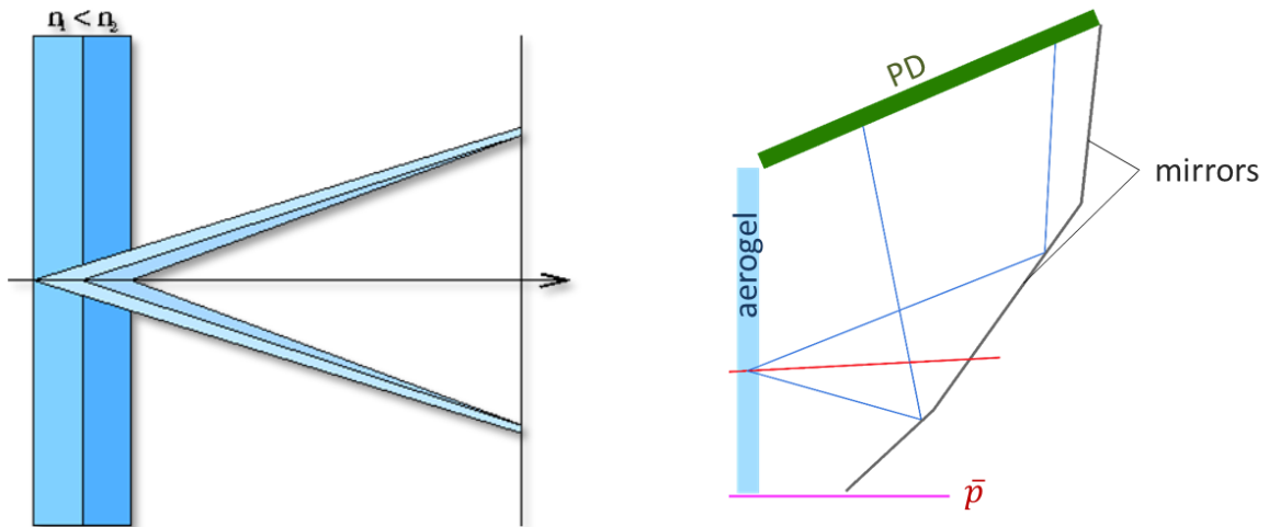
Рис. 3.36 Принцип фокусирования (слева) и принципиальная схема детектора на основе аэрогеля
