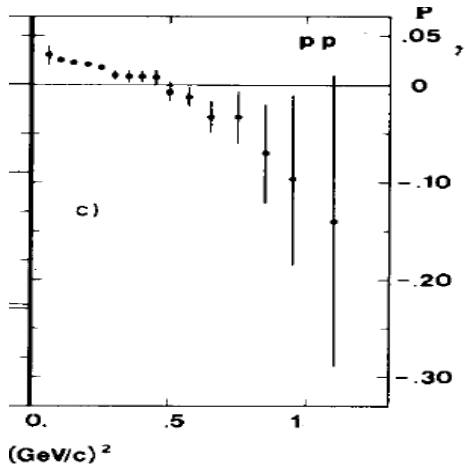
Рис. 2.20 Поляризация в упругом pp-рассеянии при импульсе 45 ГэВ/с
