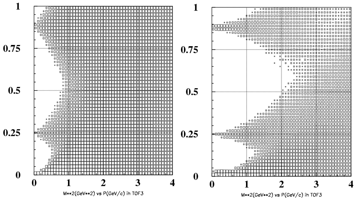
Рис. 3.38 Распределение по квадрату массы M^2 ( \text{ГэВ}/c^2 ) в зависимости от импульса частицы при расстоянии 7.6 м от мишени
