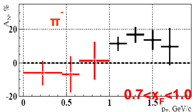
Рис. 1.13 Зависимость A_N(p_T) для реакции \pi^- d_1 \rightarrow \pi^0 X при энергии пучка 40 ГэВ, в области фрагментации \pi^- пучка [50]. Значение x_F лежит в интервале 0.7 < x_F < 1.0 .
