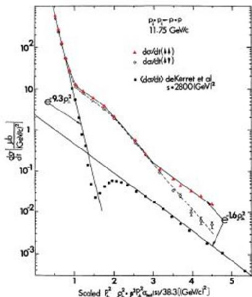
Рис. 6.1 Сечение протон-протонного упругого рассеяния в зависимости от скейлинговой переменной \rho_t^2 = \beta^2 P_t^2 \sigma_{tot}(s) / 38.3 [128].
