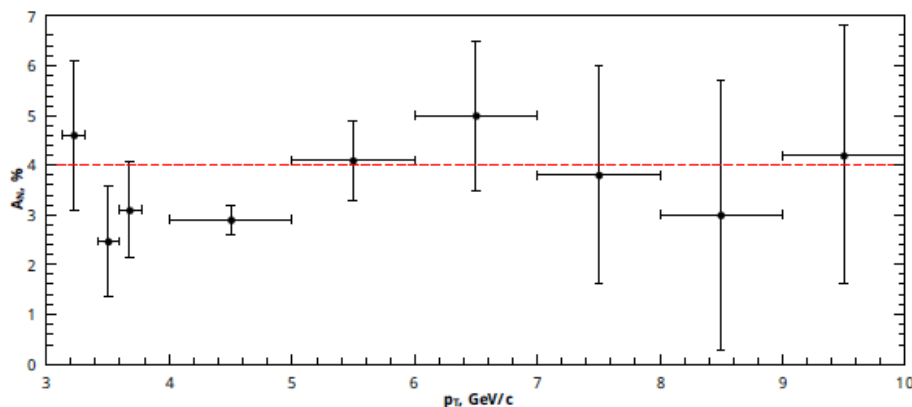
Рис. 6.22 Зависимость A_N(x_F) для p^\uparrow p \rightarrow \pi^0 X , из [178]. Угол изоляции пиона 70 мрад, \sqrt{s} = 500 ГэВ и 0.32 < x_F < 0.40 . Данные STAR из [179, 180].
