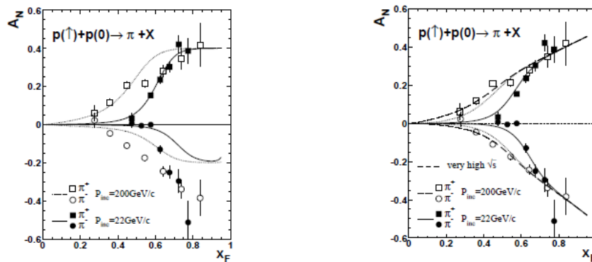
Рис. 6.19 A_N(x_F) для p^\uparrow p \rightarrow \pi^\pm X для разных значений параметров Берлинской модели [172]
