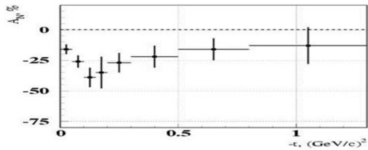
Рис. 6.4. Асимметрия в реакции \pi p \rightarrow f_2(1270)n при энергии 40 ГэВ [132], когда f_2(1270) -мезон регистрировался в моде распада на два \pi^0 -мезона.
