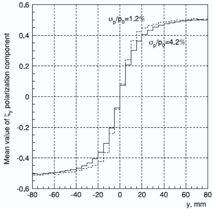
Рис. 2.6 Связь между вертикальными координатами протонов и средними значениями \xi_y компоненты вектора поляризации в промежуточном изображении для пучка с импульсом 45 ГэВ/с.
