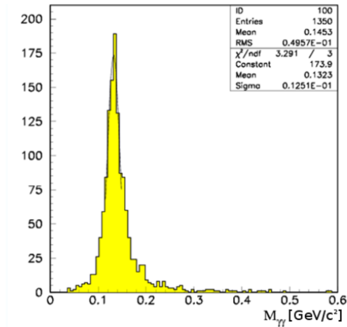
Рис. 3.34 Массовый спектр \pi^0 -мезонов с энергией от 1 до 2 ГэВ (детектор располагался на расстоянии 1,5 м от мишени).
