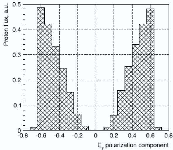
Рис. 2.9 Поляризация протонного пучка с импульсом 45 ГэВ/с на мишени установки для режимов корректора MC2, равных +0.12 Тл·м (слева) и -0.15 Тл·м (справа) при S4 = \pm 15 мм
