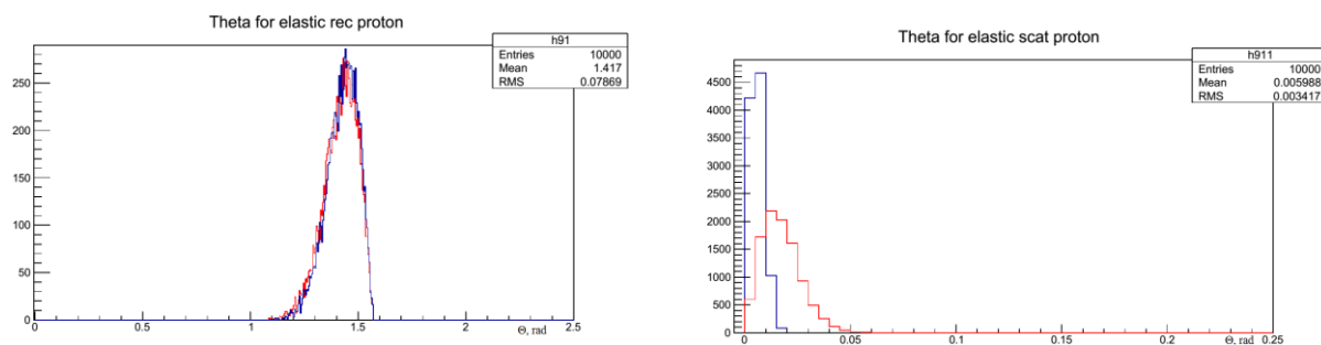
Рис. 2.21 Угловые распределения протонов отдачи (слева) и рассеяния справа для энергий 45 (синий) и 16 ГэВ
