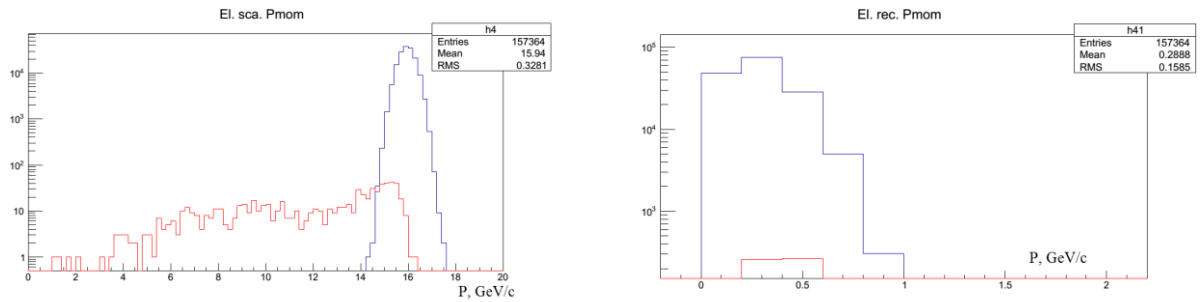
Рис. 2.25 Распределение по импульсу рассеянных частиц (слева) и частиц отдачи (справа) для упругих (синий) и дифракционных процессов
