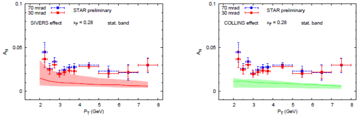
Рис. 6.18 Зависимость A_N(p_T) для реакции p \uparrow p \rightarrow \pi^0 X , из работы [166] и предсказания в рамках моделей Сиверса (слева) и Коллинза (справа)
