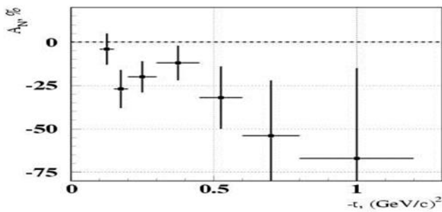
Рис. 1.14 Асимметрия в реакции \pi^- p^+ \rightarrow \omega(782)n при энергии 40 ГэВ [55], когда \omega(782) -мезон регистрировался в моде распада на \pi^0 и \gamma .
