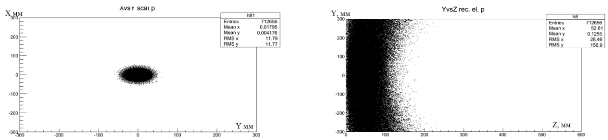
Рис. 2.22 Распределение рассеянных протонов на плоскости где находится детектор рассеянных протонов (слева) и протонов отдачи на плоскости где находится детектор отдачи (справа) для упругих событий.
