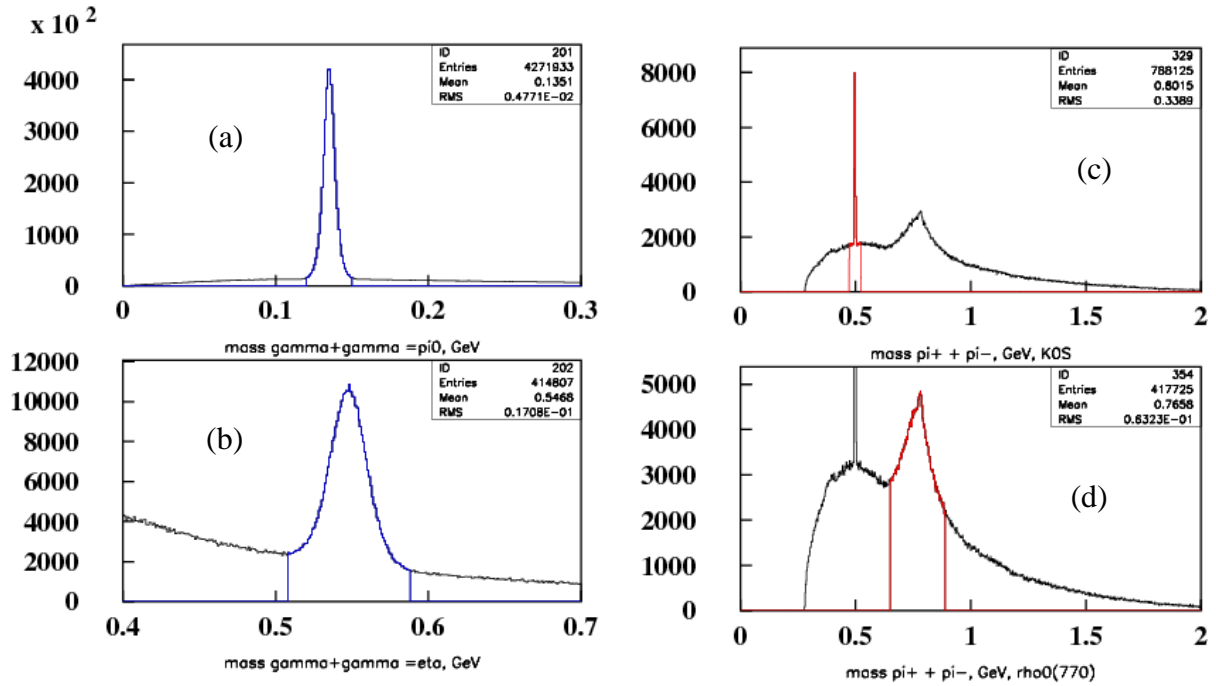
Рис. 7.4. Эффективная масса продуктов распада в процессе \pi^- p \rightarrow h + X , где h = \pi^0 \rightarrow \gamma\gamma (a); h = \eta \rightarrow \gamma\gamma (b); h = K_S^0 \rightarrow \pi^+ \pi^- (c); h = \rho^0(770) \rightarrow \pi^+ \pi^- (d).
