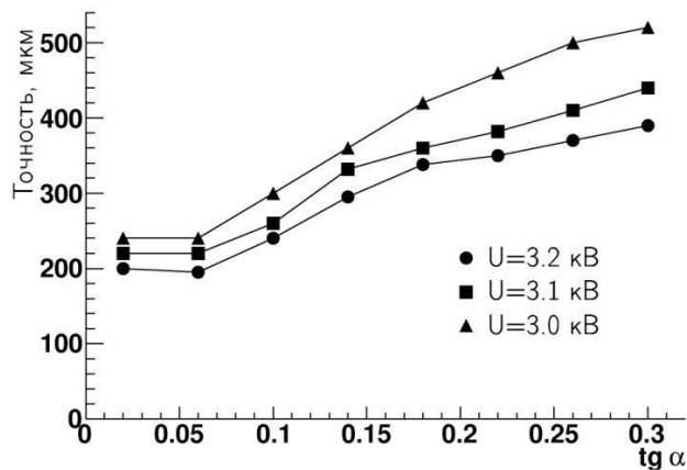
Рис. 3.29 Зависимость точности дрейфовых камер от тангенса угла наклона трека при различных напряжениях на потенциальных проволочках и фиксированном пороге дискриминации. Угол отсчитывается от нормали к плоскости камеры в плоскости, перпендикулярной направлению проволочек.
