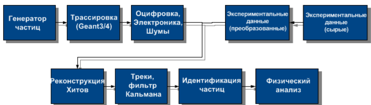
Рис. 3.50. Схематическое представление цепочки выполнения этапов в среде SpascharmRoot.
