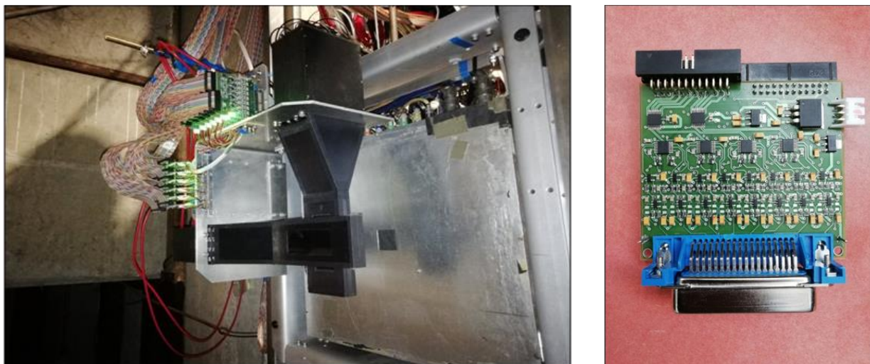
Рис. 3.6 Фотография волоконного годоскопа в зоне экспериментальной (слева) и 16-канального дискриминатора с регулируемым порогом волоконного годоскопа
