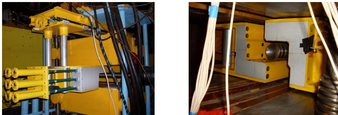
Рис. 3.8 Фотография veto-системы вокруг поляризованной протонной мишени
