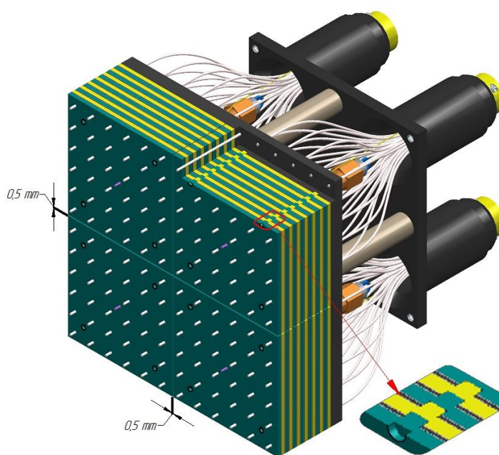
Рис. 3.31 Часть модуля калориметра в разрезе
