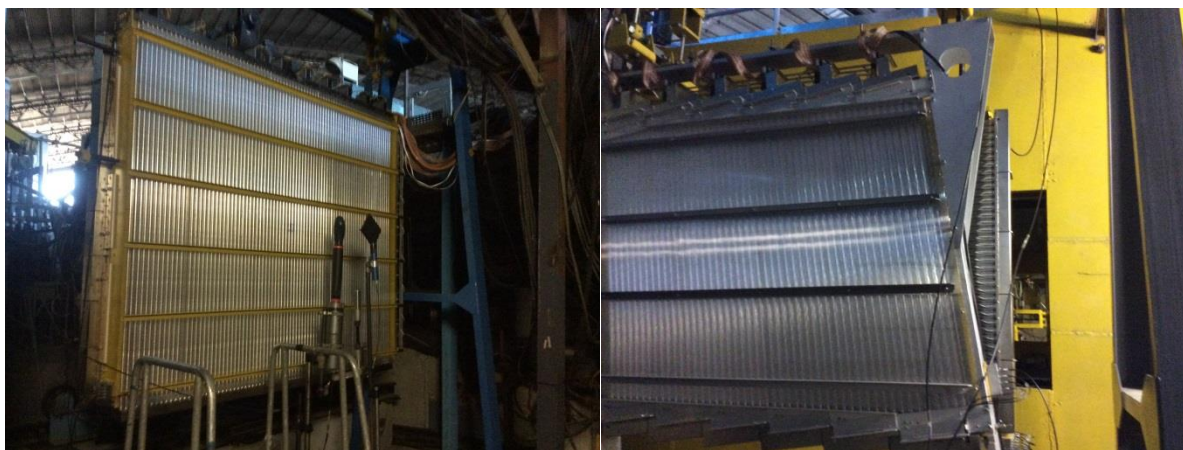
Рис. 3.24 Четвертая станция камер на рабочем месте с установленным перед ней триггерным счетчиком на взаимодействие, справа – третья станция, расположенная сразу после магнита.
