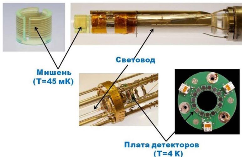
Рис. 3.13 Основные внутренние узлы, созданной совместными усилиями (Майнц-Бонн-Бохум-ОИЯИ) мишени-сцинтиллятора
