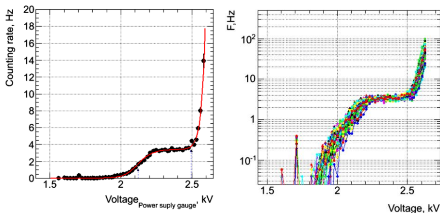
Рис. 3.23 Счетные характеристики всех трубок(правая панель) и усредненная характеристика всей камеры (левая панель)
