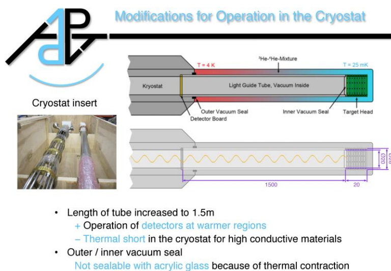
Рис. 3.14 Поляризованная мишень-сцинтиллятор (Майнц)
