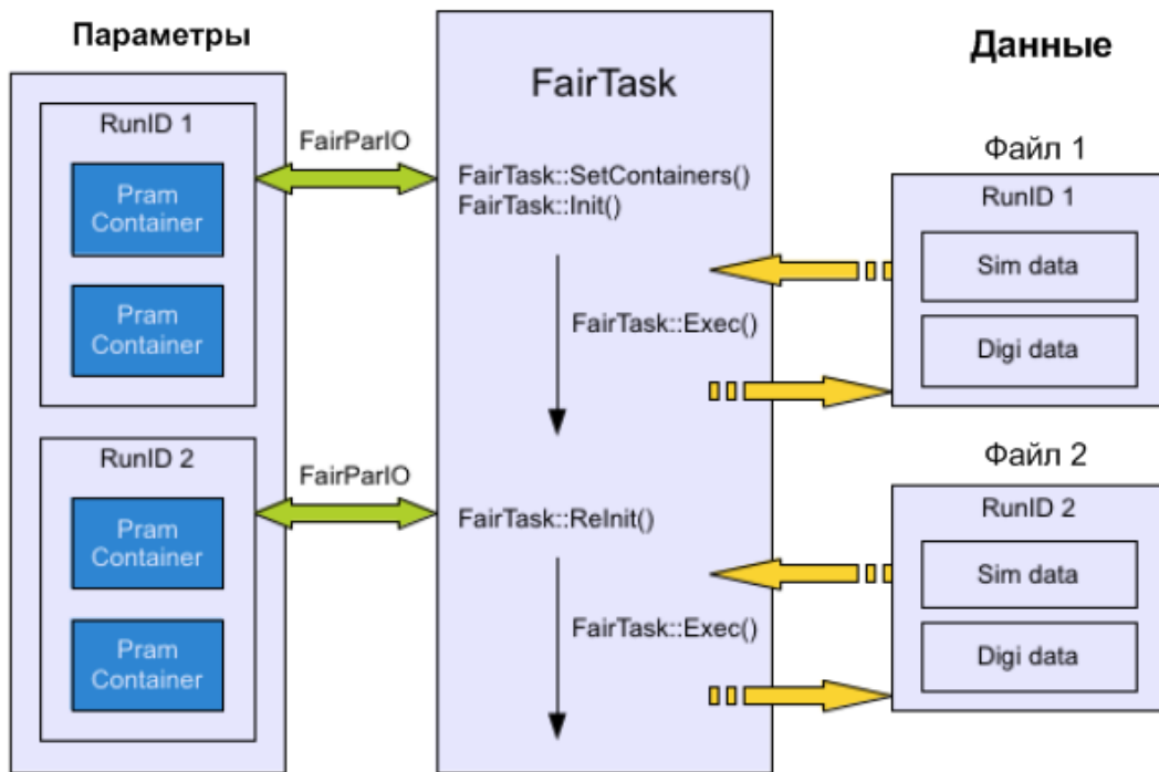
Рис. 3.49 Схематическое представление схемы процессов в FairTask, а также механизма обращения к параметрам и данным. Данные и параметры связаны через уникальный идентификатор “RunID”.
