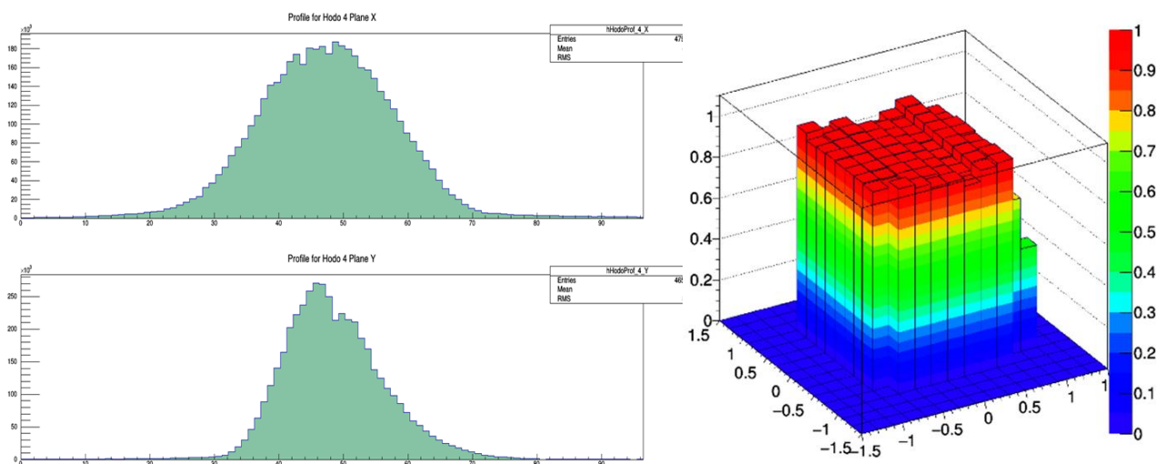
Рис. 3.7 Профили пучка (слева) и зависимость эффективности волоконного годоскопа от координаты
