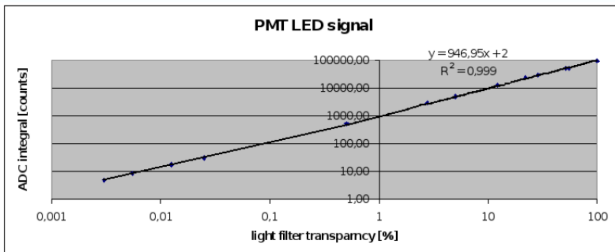
Рис. 3.32 Проверка линейности фотоумножителя
