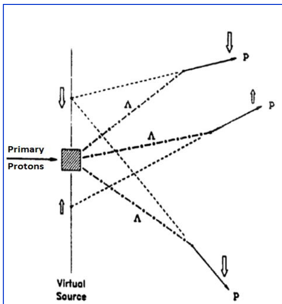
Рис. 2.2. Схема получения пучка поляризованных протонов из распадов \Lambda -гиперонов.
