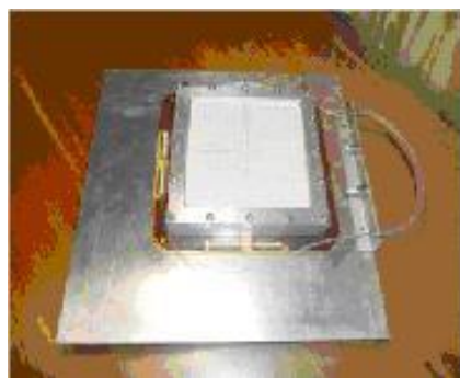
Рис. 3.21 Фотографии двух прототипов GEM детекторов для установки СПАСЧАРМ.
