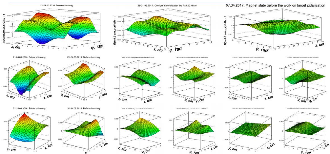
Рис. 3.10 Результаты измерения поля магнита поляризованной мишени в начале измерений (слева), после работы в начале 2017 г. (в центре) и в настоящее время (справа)
