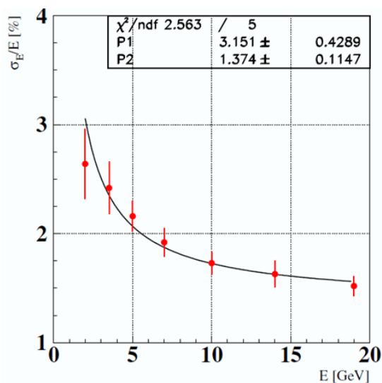
Рис. 3.33 Результаты измерения прототипа калориметра в ИФВЭ
