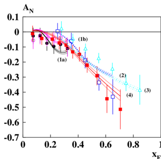
Рис. 6.29 A_N(x_F) для реакции p^\uparrow p(A) \rightarrow \pi^- + X .
