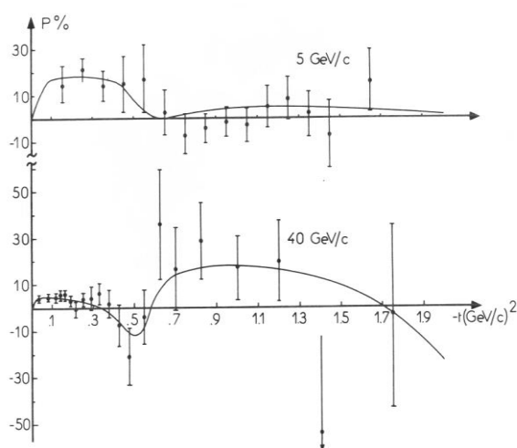
Рис. 6.3 Модель оддерона [131] в применении к описанию поляризации в реакции \pi^- p(\uparrow) \rightarrow \pi^0 n при импульсах 5 и 40 ГэВ/с [53].
