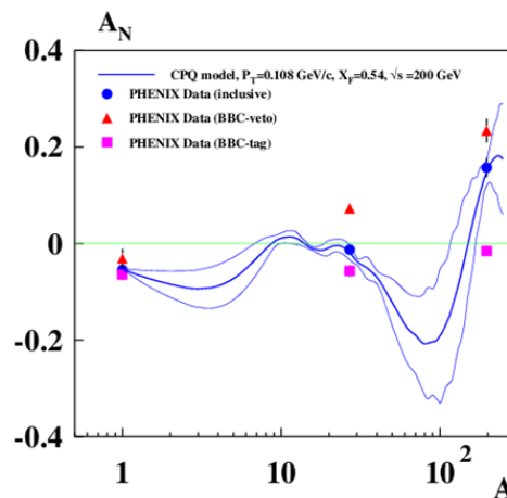
Рис. 1.9 Зависимость A_N(A) для реакции p^\uparrow A \rightarrow n + X в эксперименте PHENIX [29].
