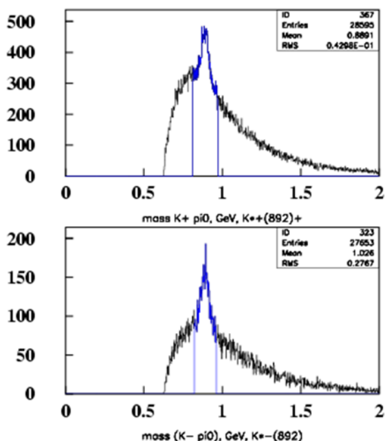
Рис. 7.2 Эффективная масса продуктов распада в процессах типа pp \rightarrow h + X : где h = K^{*+}(892) \rightarrow K^+ \pi^0 (вверху) и h = \tilde{K}^{*-}(892) \rightarrow K^- \pi^0 (внизу)
