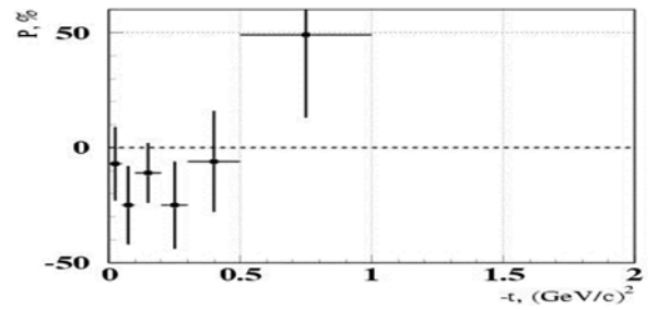
Рис. 1.15 Асимметрия в реакции \pi^- p^+ \rightarrow \eta'(958)n при энергии 40 ГэВ [132], когда \eta'(958) -мезон регистрировался в моде распада на два \gamma -кванта
