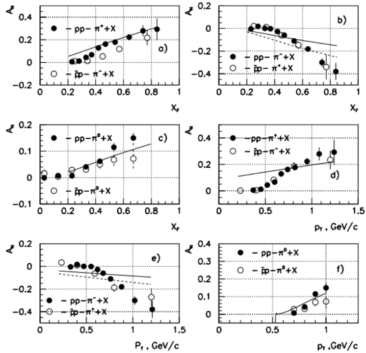
Рис. 6.26 Сравнение данных E704 для p^\uparrow p (черные кружочки) [23] и p^\uparrow p (открытые кружочки) [190], из работы [188].
