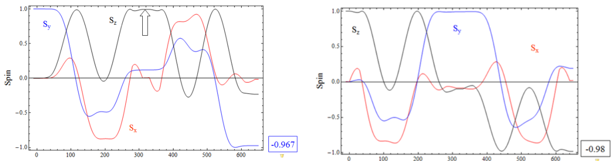
Рис. 2.28 Спиновые траектории для поперечной (слева) и продольной (справа) поляризаций
