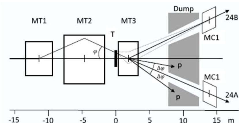
Рис. 2.3 Схема мишенной станции каналов 24А и 24В. Т – первичная мишень, МТ1÷МТ3 – дипольные магниты, МС – магниты-корректоры, Dump – стальной поглотитель длиной 5 м. Приведенный на схеме мишенной станции вариант наведения протонного пучка на мишень соответствует отбору нейтральных вторичных частиц в канал 24А и положительно (отрицательно) заряженных частиц в канал 24В. Пунктирными линиями показаны траектории вторичных заряженных частиц, отбираемых с канал 24В с ненулевыми углами рождения в мишени.
