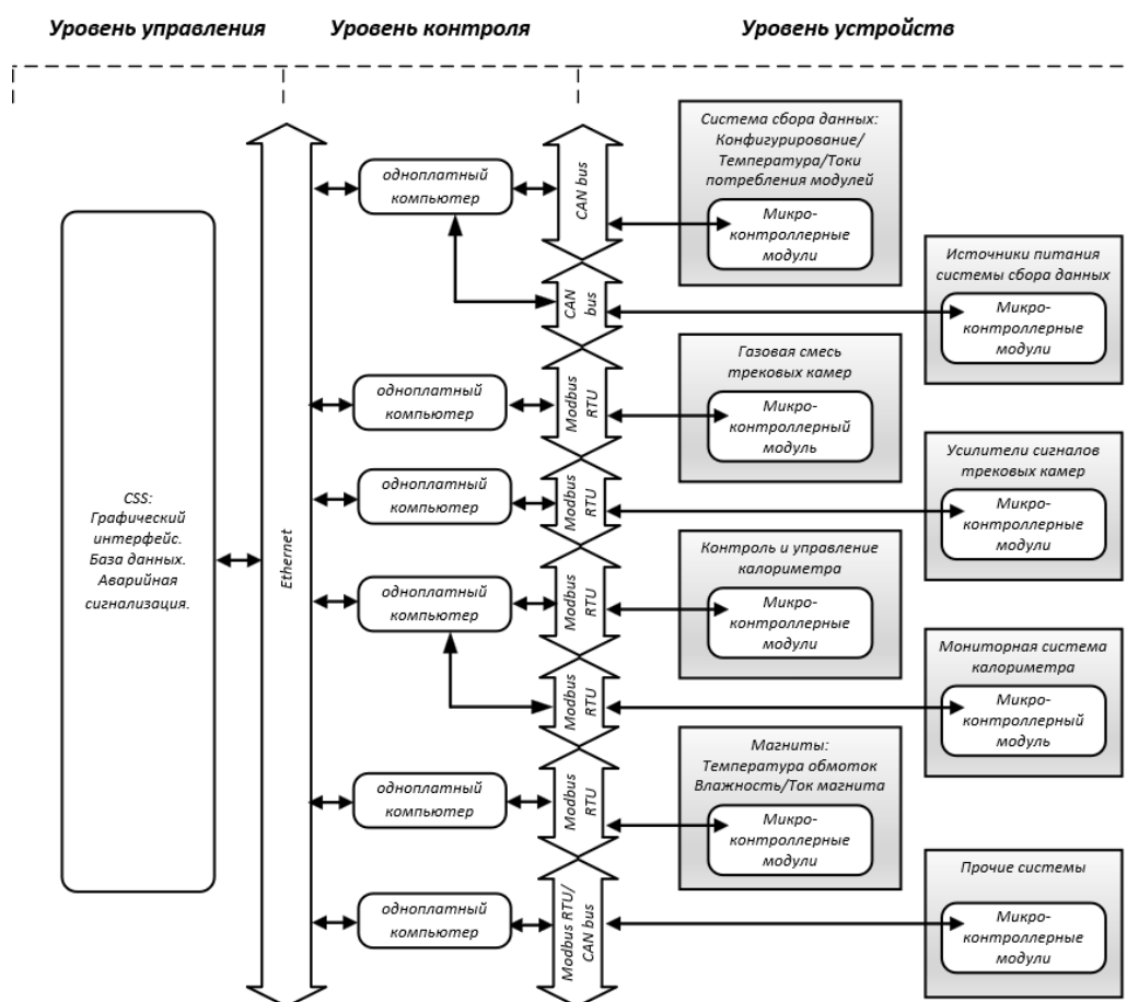
Рис. 3.42 Архитектура системы управления экспериментальной установки СПАСЧАРМ: Control System Studio.
