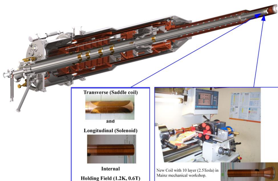
Рис. 3.12 Криостат поляризованной мишени с поляризующей и удерживающей поляризацию сверхпроводящими катушками.
