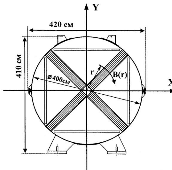
Рис. 3.39 Внешний вид магнита магнитного спектрометра установки «Нейтринный Детектор ИФВЭ-ОИЯИ»
