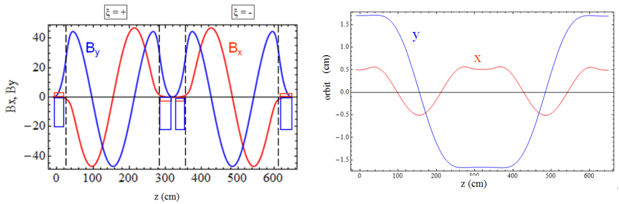
Рис. 2.27 Магнитное поле двух геликоидальных магнитов и траектория частиц внутри змейки при единичной матрице
