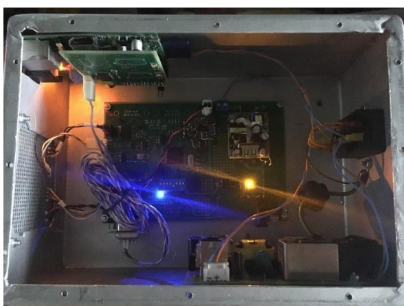
Рис. 3.45 Модуль мониторинга параметров магнита мишени «Динозавр»
