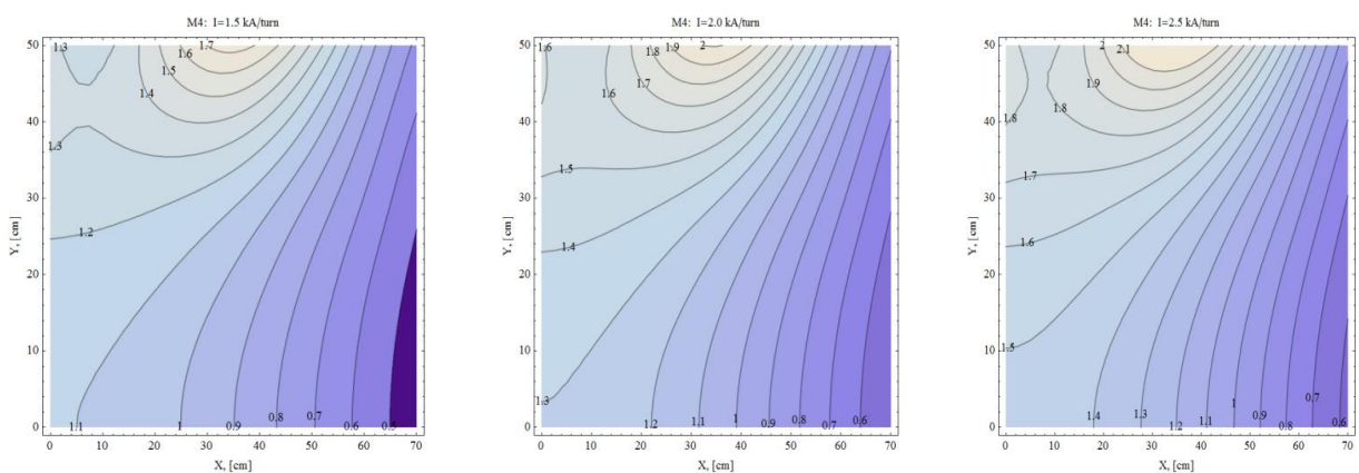
Рис. 3.18 Изолинии интегрального поля в четвертой части рабочей области 700 \times 500 мм 2 . I = 1.5, 2.0 и 2.5 кА/виток
