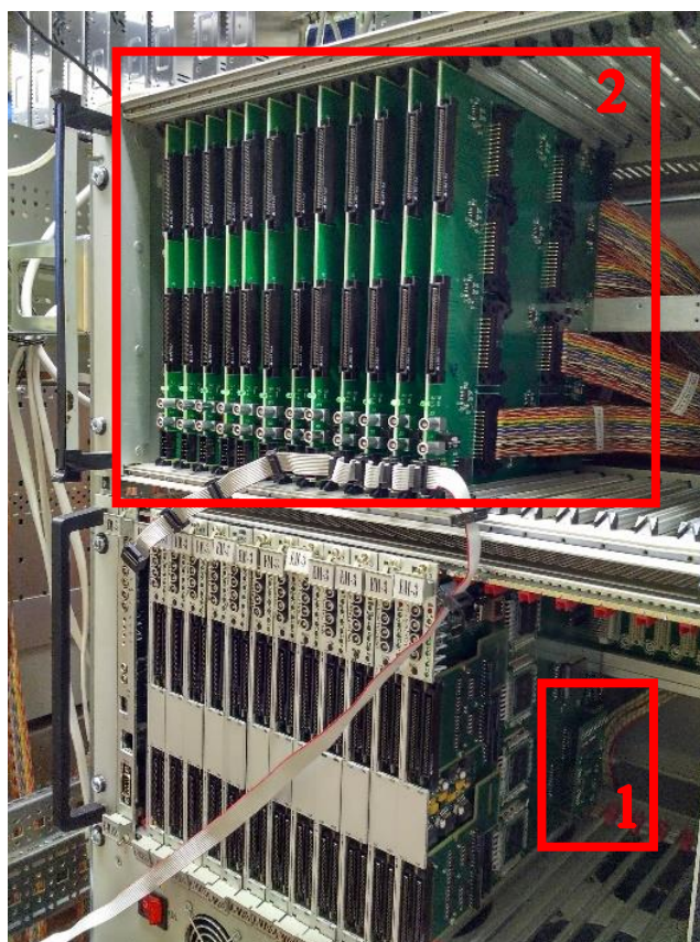
Рис. 3.44 Мезонинная плата, установленная на модуль ЕвроМИСС – 1; переходные платы – 2
