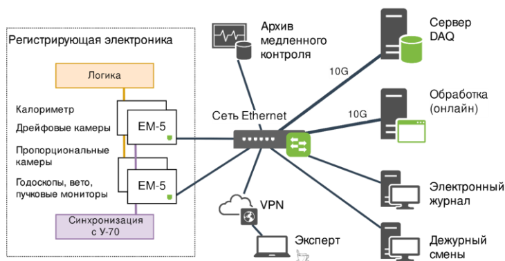
Рис. 3.41 Сеть системы сбора данных установки
