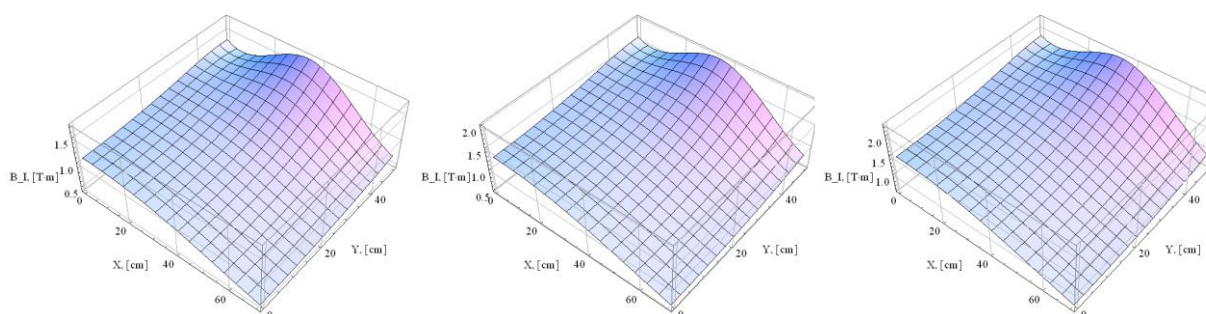
Рис. 3.19 Интегральное поле как функция поперечных координат (X,Y) в рабочей области. I = 1.5, 2.0 и 2.5 кА/виток
