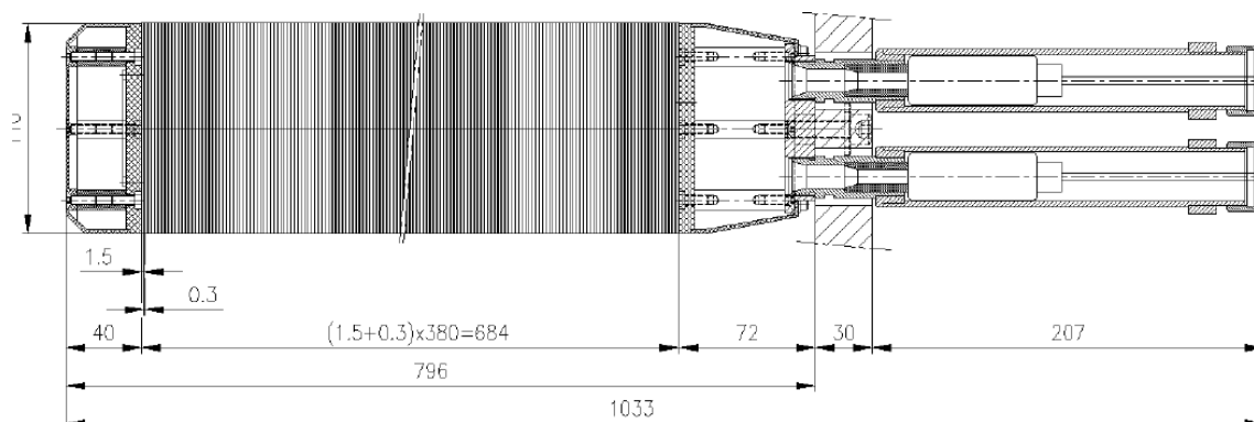
Рис. 3.21 Чертеж супермодуля калориметра
