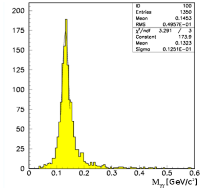
Рис. 3.25 Массовый спектр \pi^0 -мезонов с энергией от 1 до 2 ГэВ (детектор располагался на расстоянии 1,5 м от мишени).
