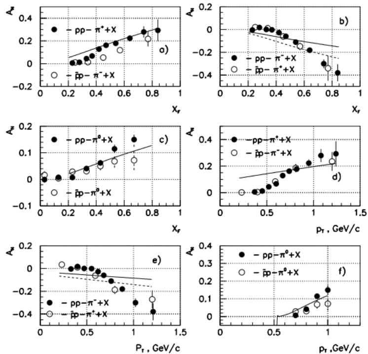
Рис. 6.26 Сравнение данных E704 для p^\uparrow p (черные кружочки) [23] и p^\uparrow p (открытые кружочки) [166], из работы [164].
