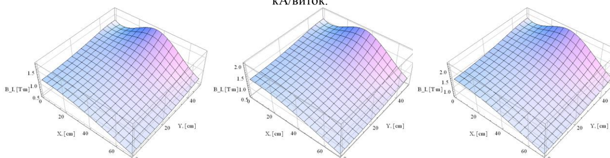
Рис. 3.11 Интегральное поле как функция поперечных координат (X,Y) в рабочей области. I = 1.5, 2.0 и 2.5 кА/виток
