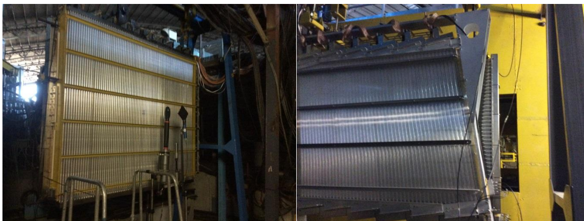
Рис. 3.15 Четвертая станция камер на рабочем месте с установленным перед ней триггерным счетчиком на взаимодействие, справа – третья станция, расположенная сразу после магнита.
