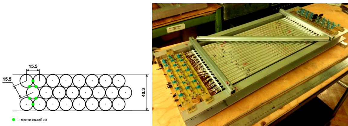
Рис. 3.13 Схема расположения трубок (левая панель) и фото камеры с открытыми платами (правая панель)
