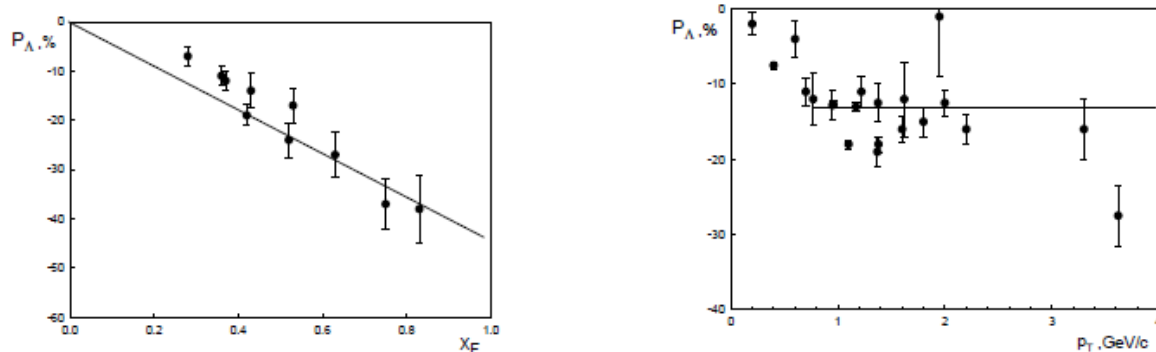
Рис. 6.23 P_N(x_F) (слева) и P_N(p_T) (справа) для реакции pp(A) \rightarrow \Lambda^1 X , сплошные линии – предсказания по модели фильтрации спина [157]
