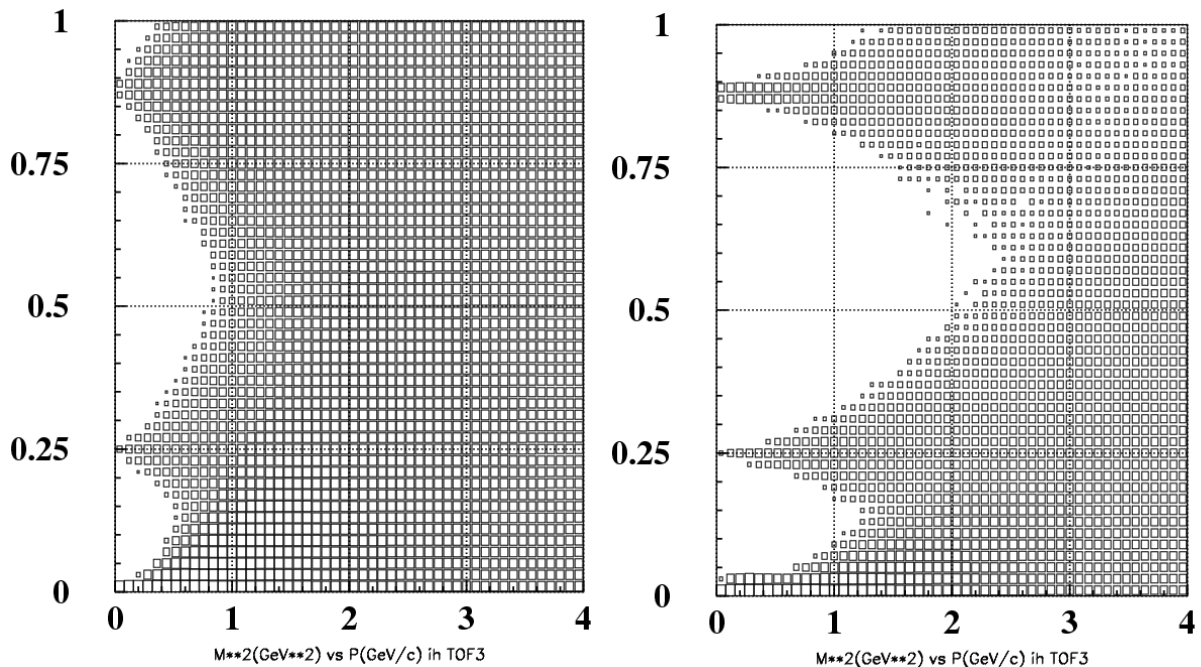
Рис. 3.29 Распределение по квадрату массы M^2 (ГэВ 2 /с 2 ) в зависимости от импульса частицы при расстоянии 7.6 м от мишени
