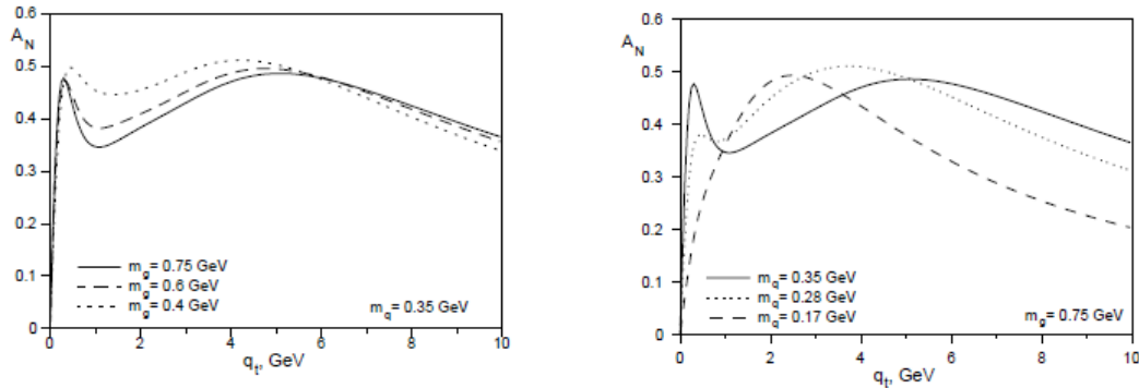
Рис. 6.21 A_N(q_t) для рассеяния кварков, при разных параметрах m_g инфракрасного обрезания (слева) и разных динамических массах кварка (справа) из модели [152]
