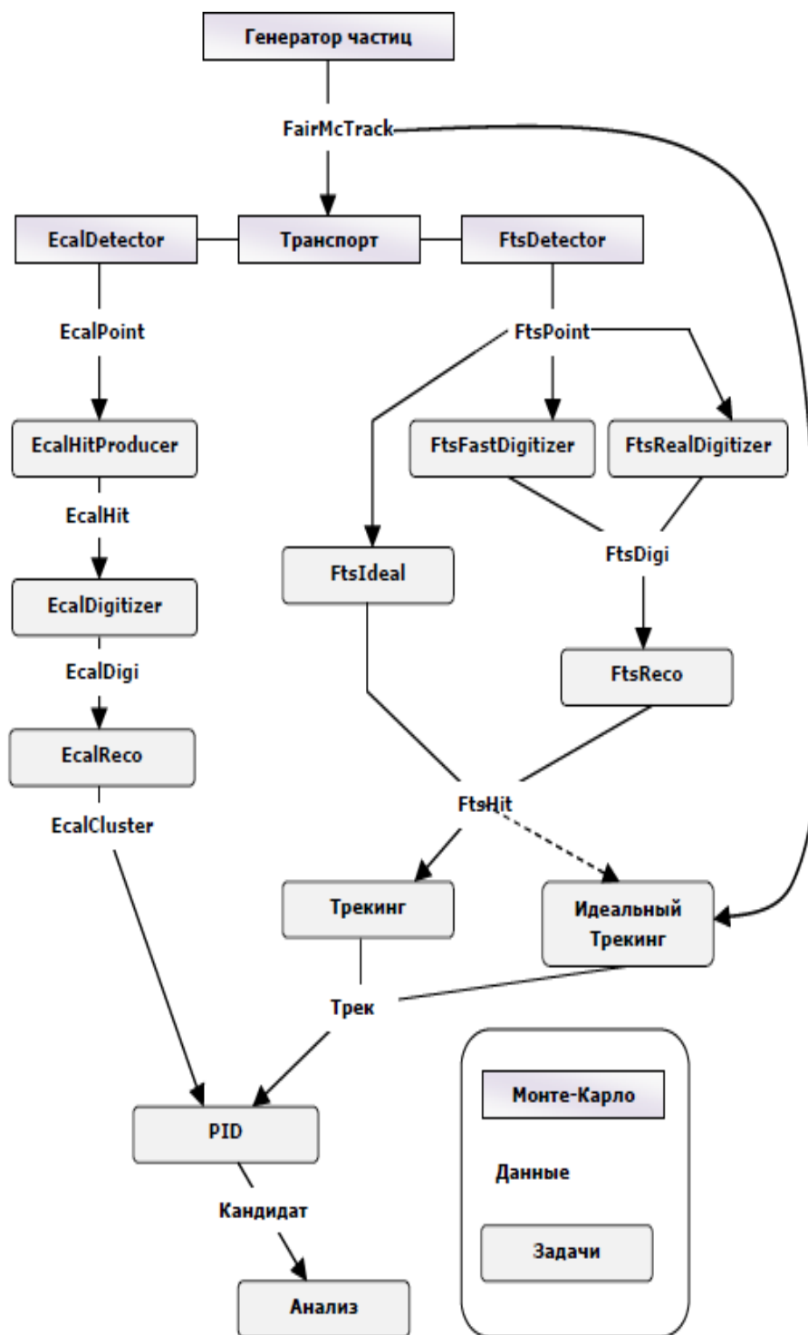
Рис. 3.37. Последовательность выполнения «задач» в среде SpascharmRoot на примере детектора идентифицирующего частицы (калориметр или ECAL) и трекового детектора (система станций дрейфовых трубок или FTS) при моделировании. Модульная архитектура программной среды позволяет подключать компоненты, необходимые для конкретного случая.
